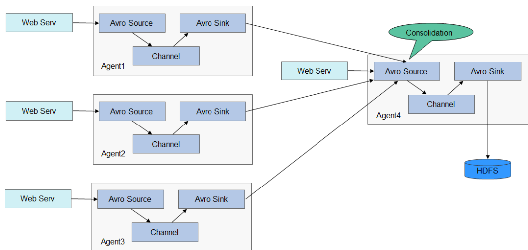
图 1-30 Flume 级联结构图
