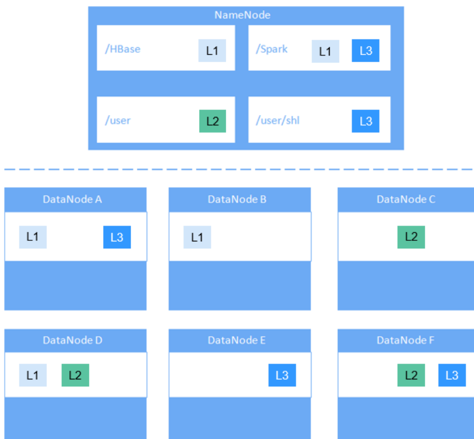
图 1-56 基于标签的数据块摆放策略样例
