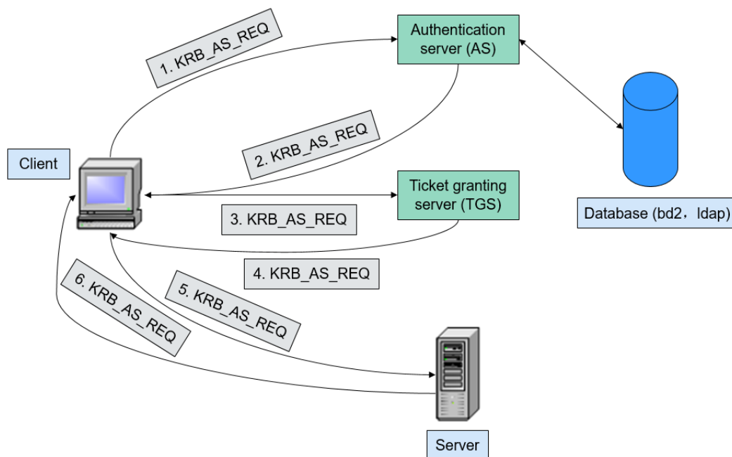
图 1-70 认证流程图
