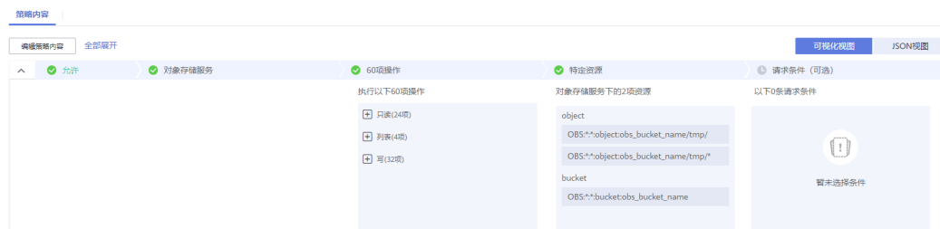
图 18-61 自定义策略
