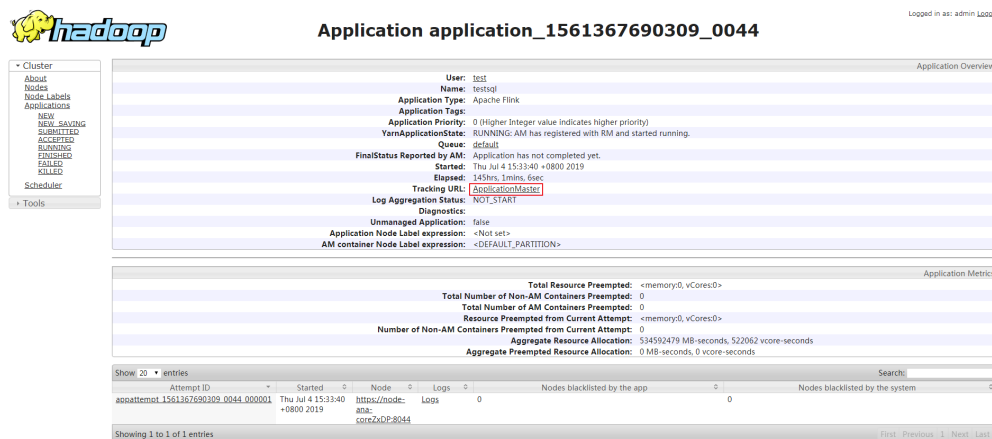
图 10-10 application
