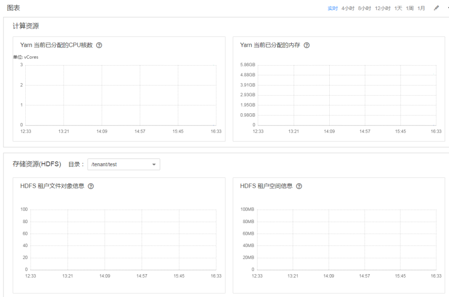
图 12-15 精细化监控
