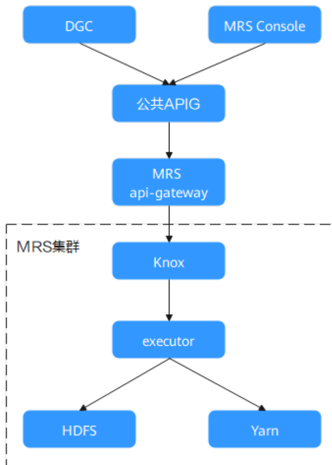
图 18-7 作业流程
