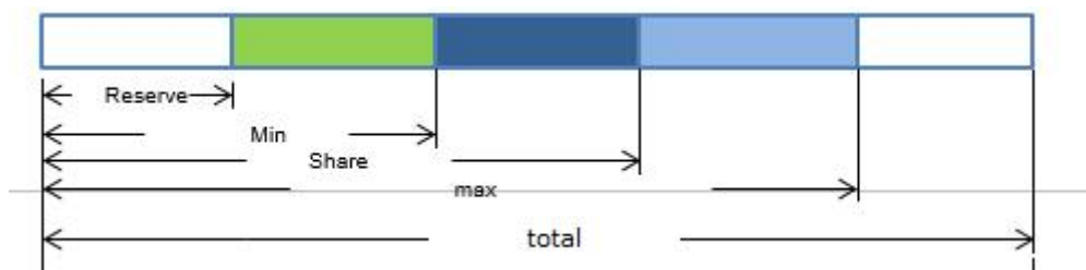
图 1-136 策略示意图
