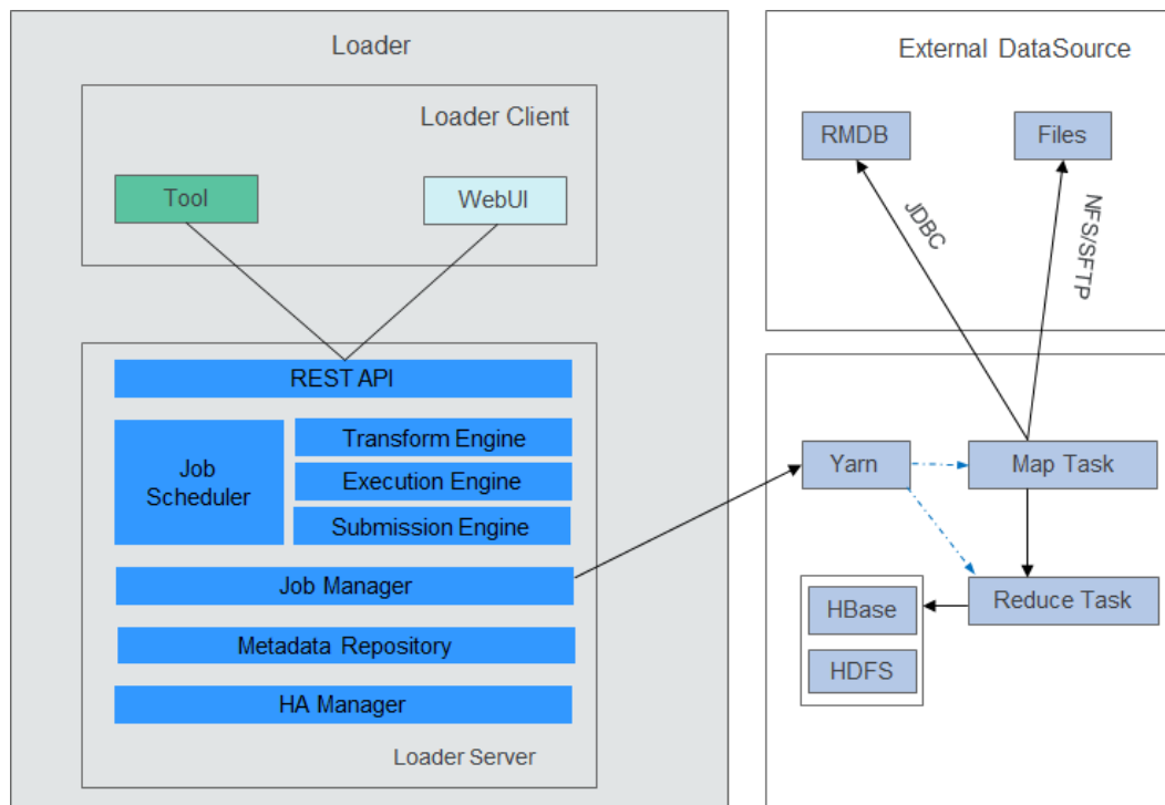
图 1-74 Loader 模型
