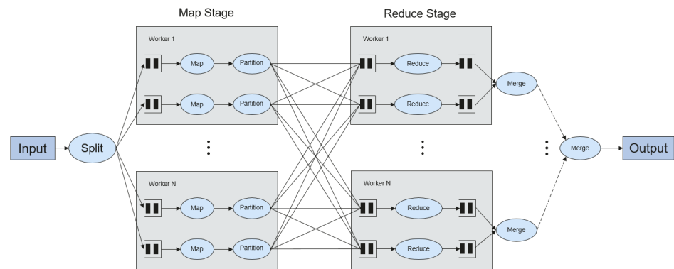
图 1-114 算法流程
