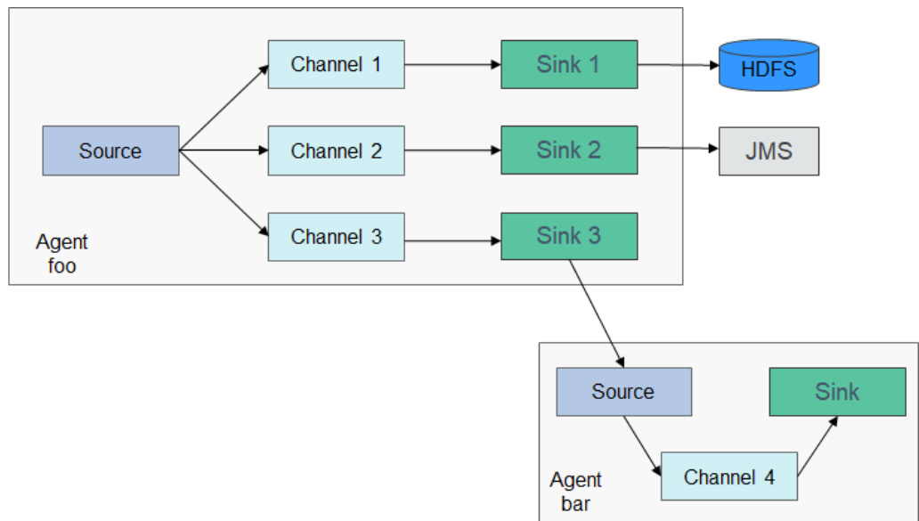
图 1-29 Flume 结构图
