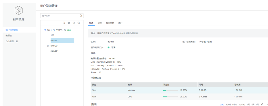
图 12-14 多租户管理
