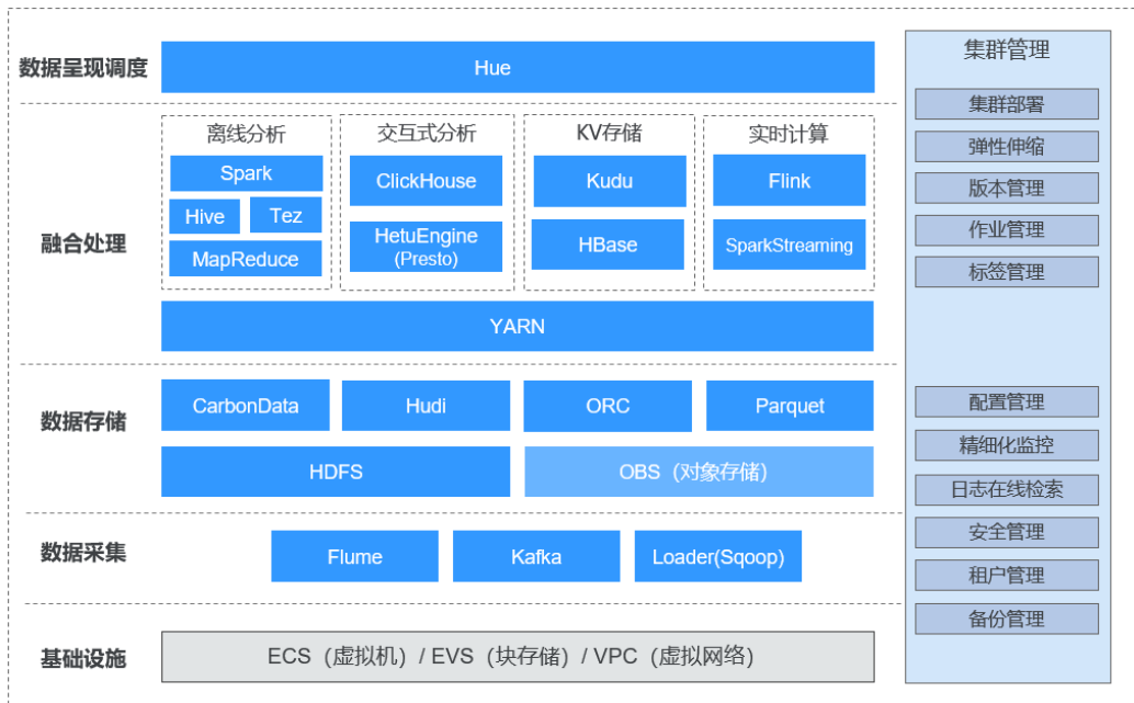
图 1-1 MRS 架构
