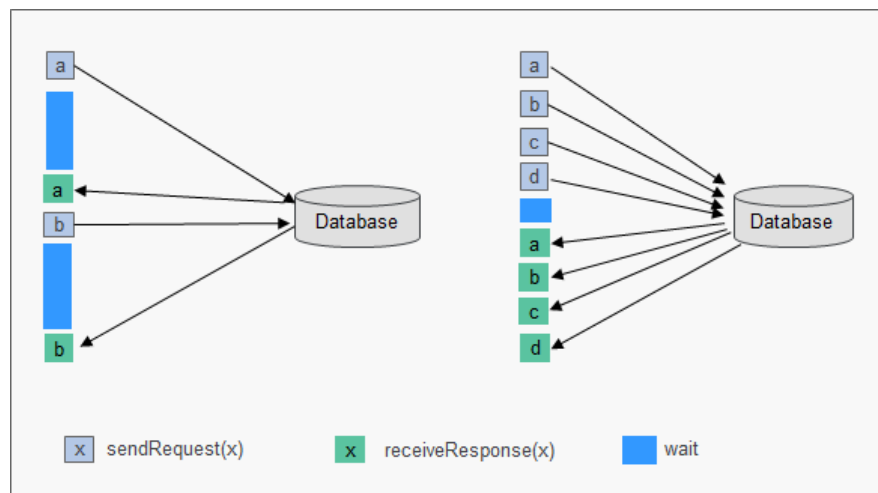
图 1-27 Async.I/O 的比较
