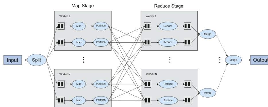
图 1-96 算法流程
