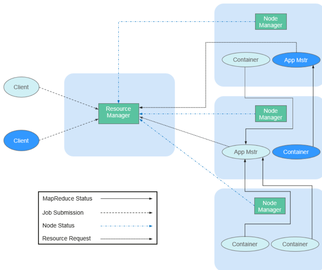
图 1-128 YARN 结构
