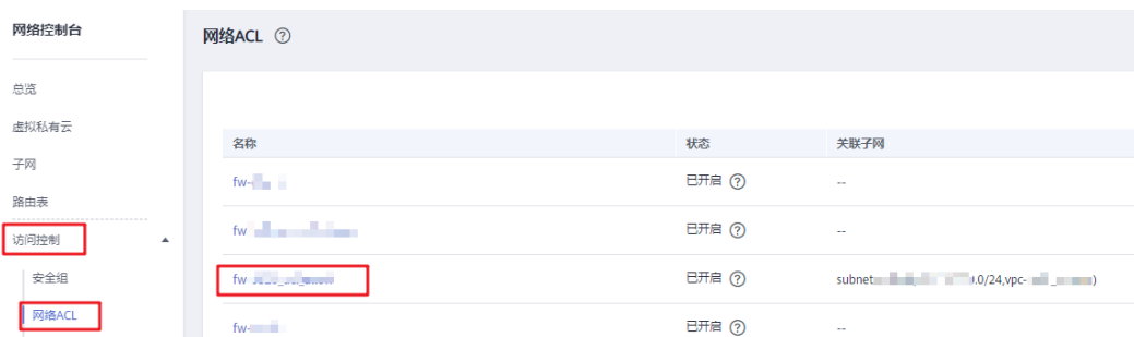
图 5-2 网络 ACL
