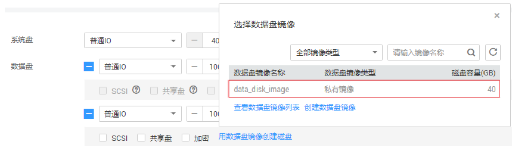
图 3-7 添加数据盘
