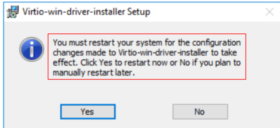
图 4-19 重启提示
