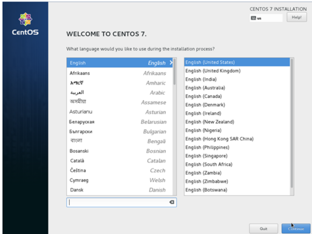
图 3-31 安装界面
