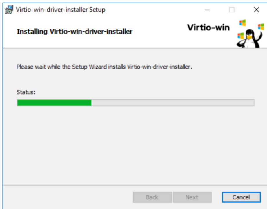
图 4-17 安装中
