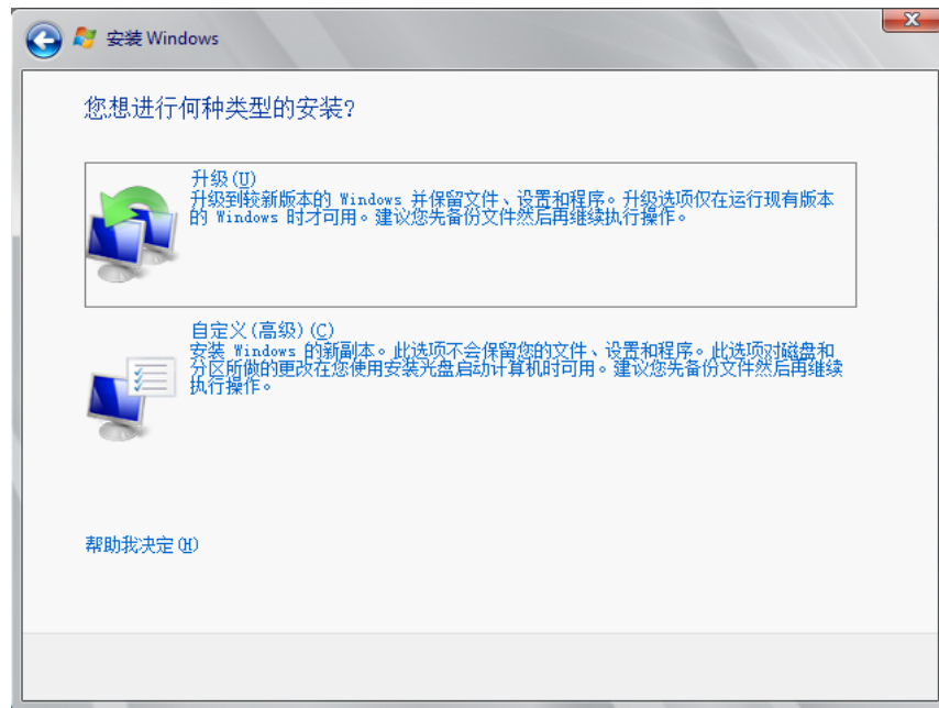
图 3-16 安装类型
