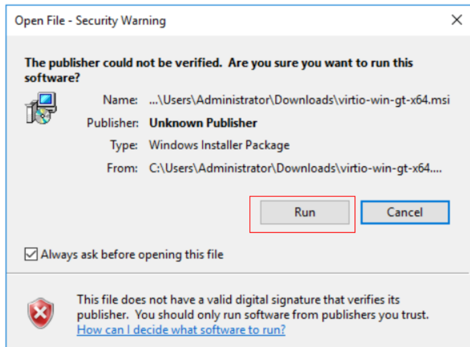
图 4-12 单击 RUN
