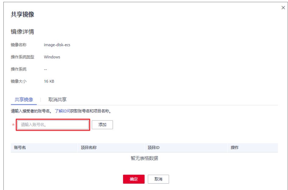
图 4-8 共享镜像
