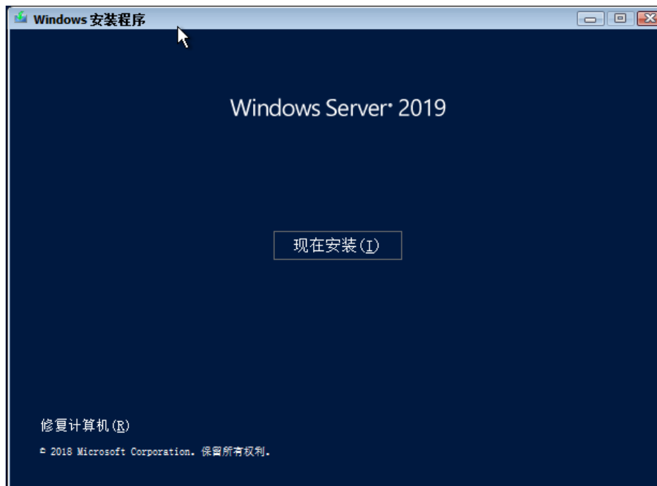
图 3-15 安装确认
