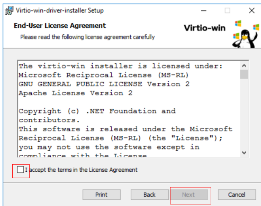
图 4-14 勾选协议
