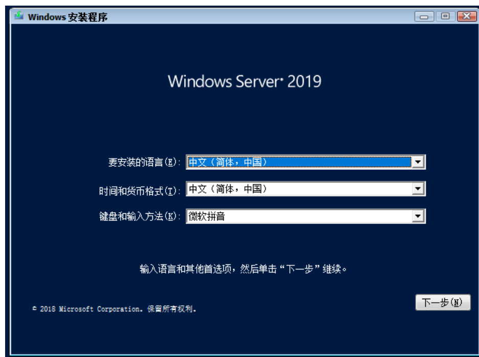
图 3-14 安装首选项
