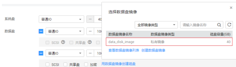
图 3-9 添加数据盘
