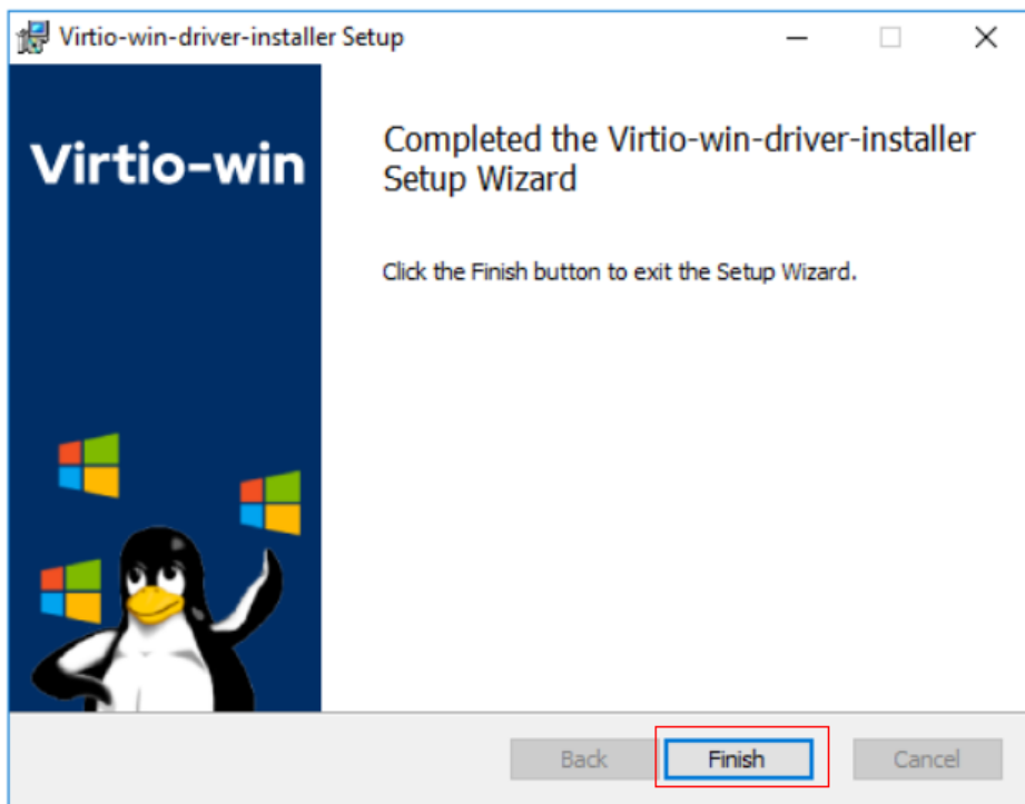
图 4-18 安装完成
