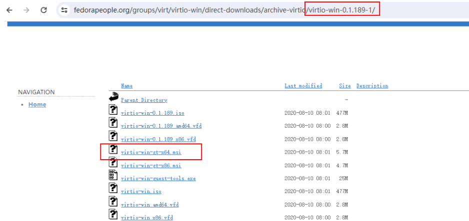
图 4-11 下载驱动
