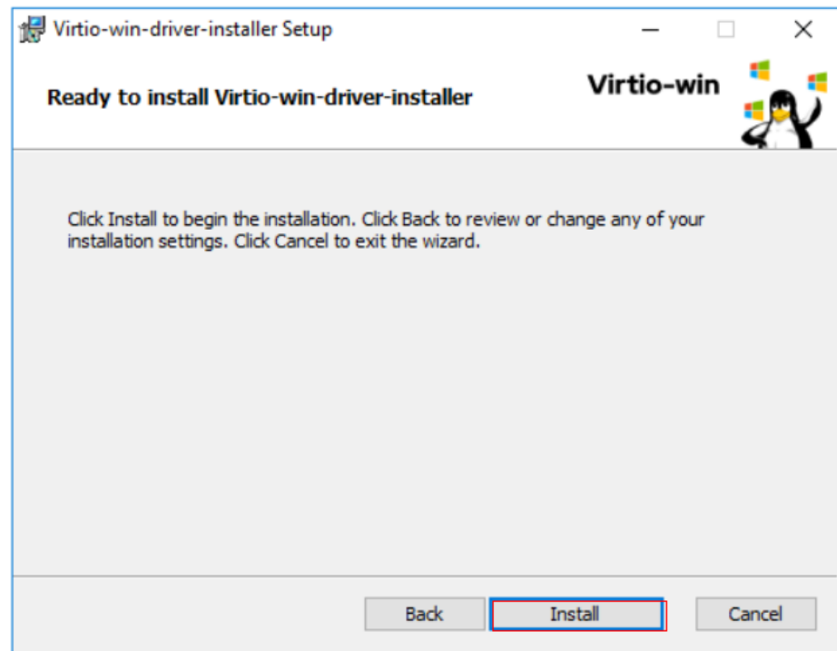
图 4-16 单击安装
