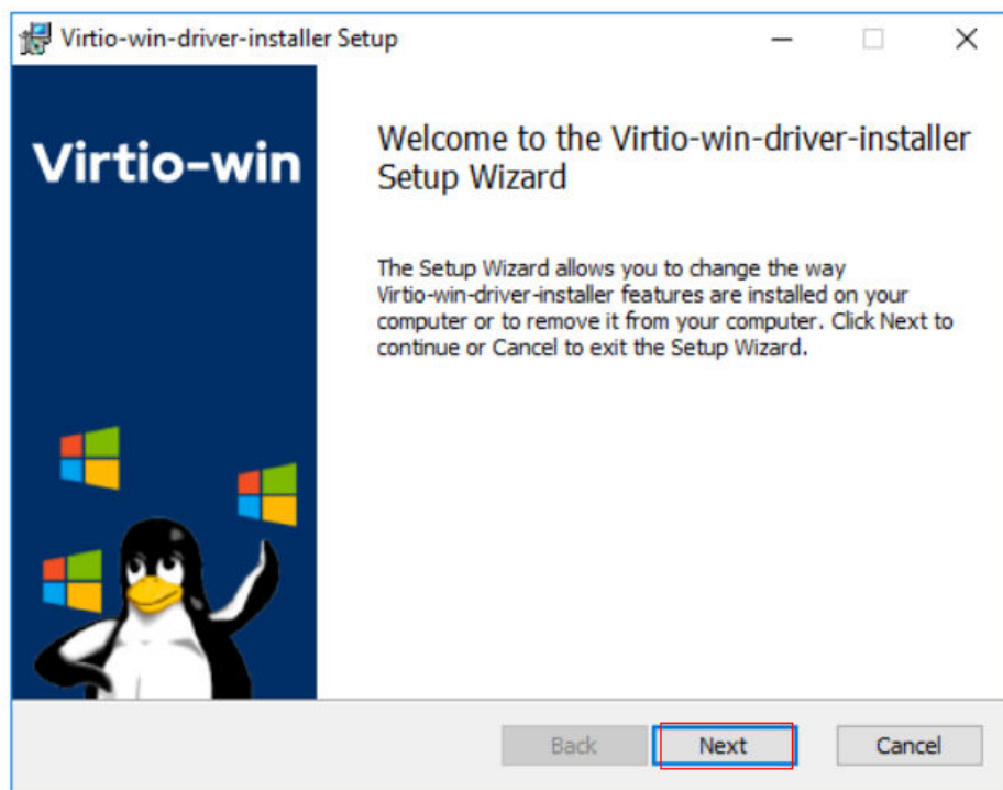
图 4-13 单击 Next
