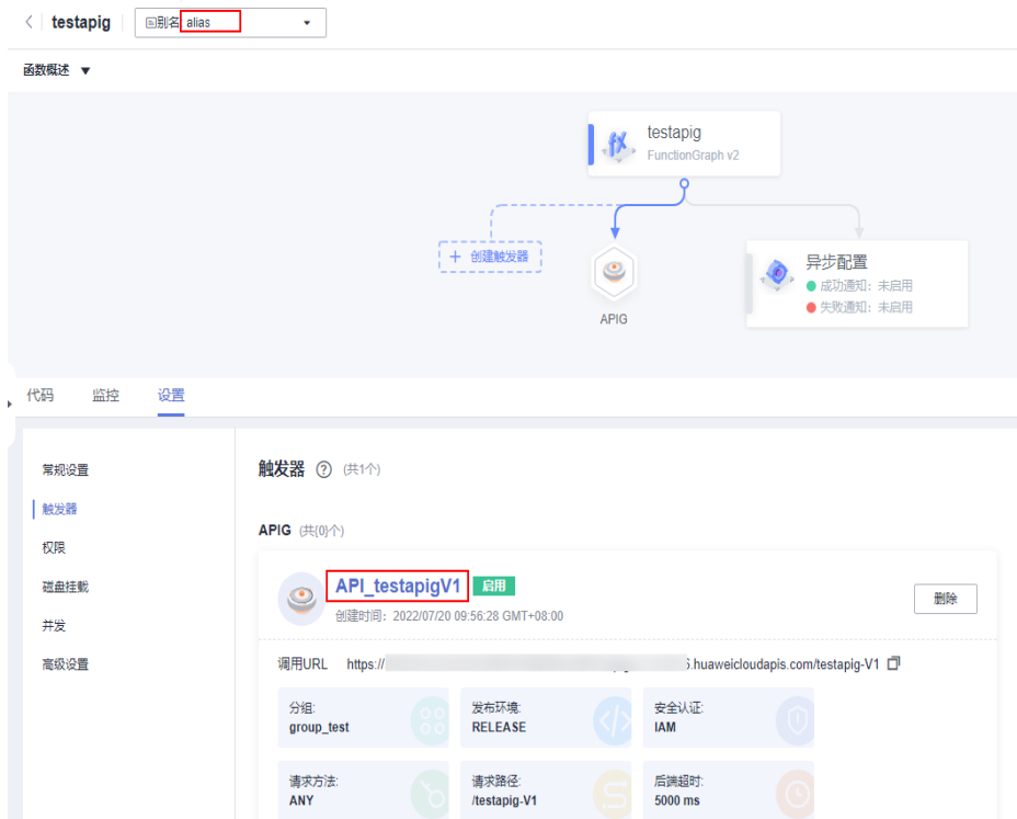
图 15-16 在 alias 下创建触发器
