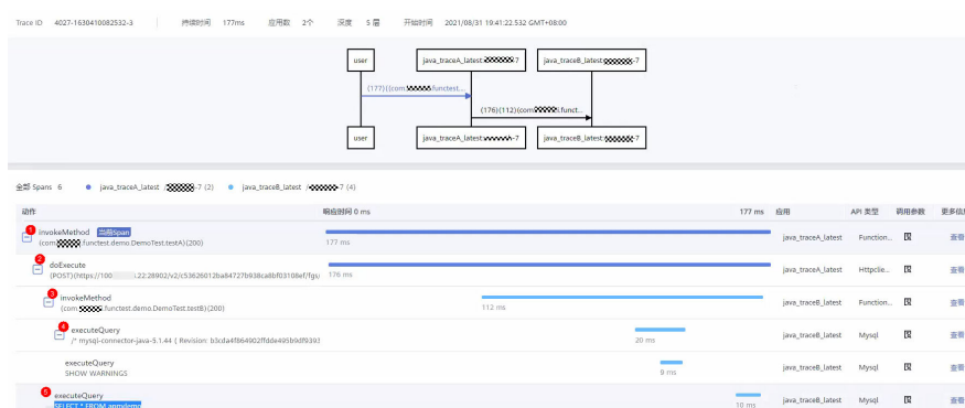
图 9-9 函数 A 调用函数 B 详情
