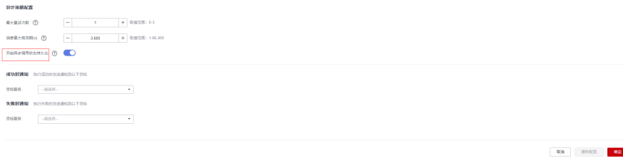
图 15-4 开启异步调用持久化
