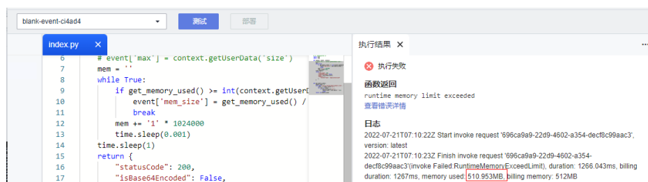
图 15-12 查看 oom 内存大小
