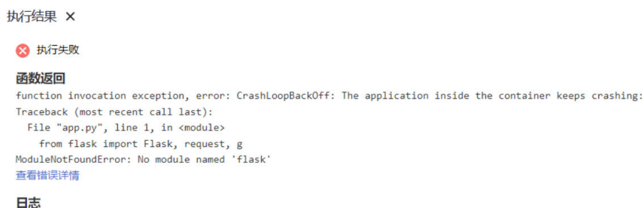
图 15-13 查看执行结果
