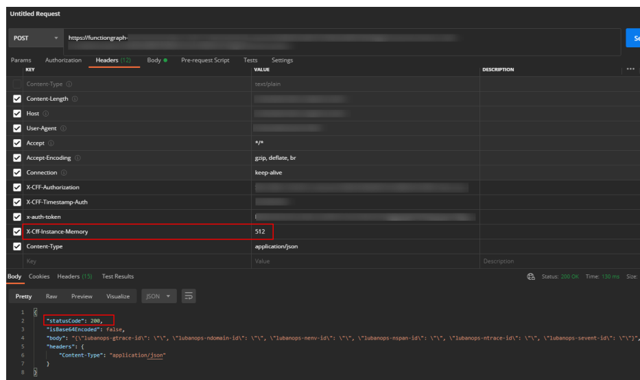
图 5-19 添加请求头并调用
