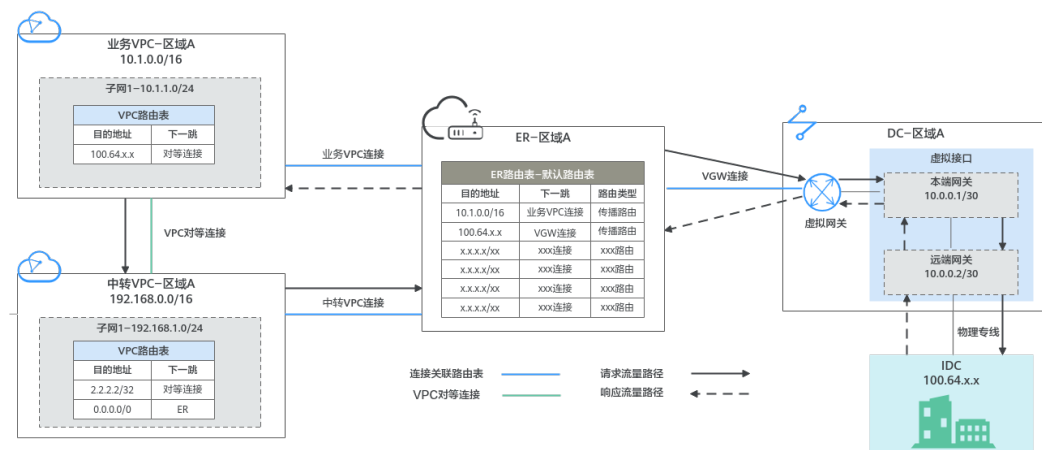
图 16-1 中转 VPC 组网示例
