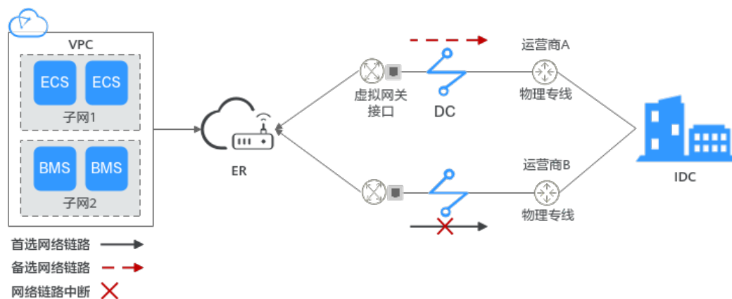
图 1-4 多条专线链路动态选路和切换
