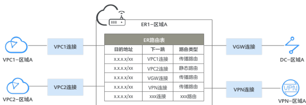
图 4-1 连接概述
