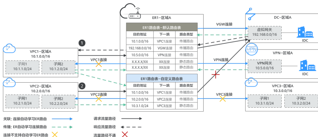
图 1-6 企业路由器工作原理图
