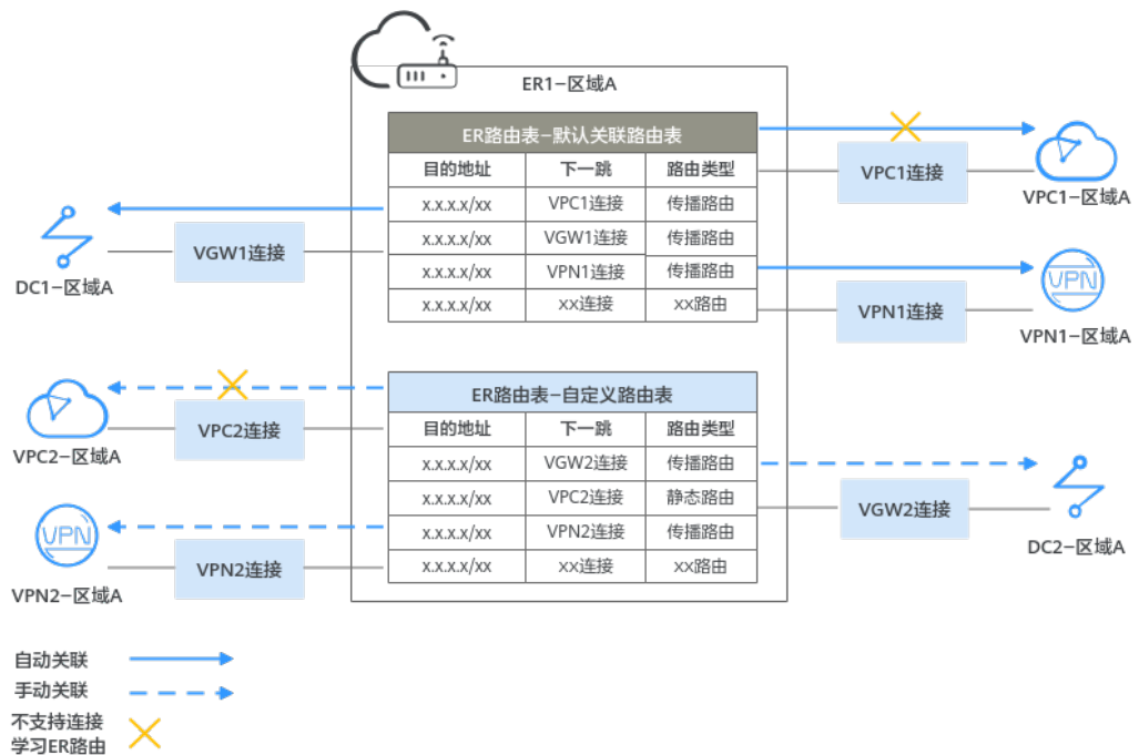
图 6-1 关联概述
