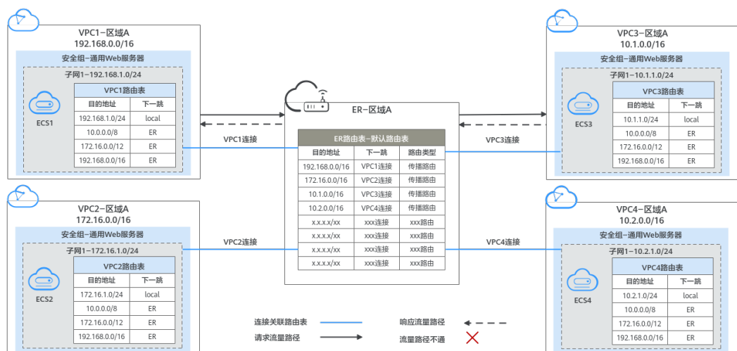
图 2-5 同区域 VPC 互通组网规划
