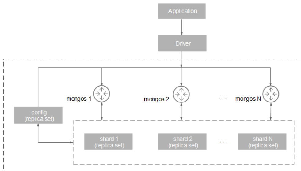
图 1-1 集群架构
