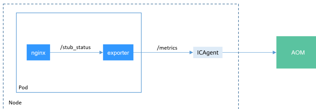
图 12-2 使用 exporter 转换数据格式
