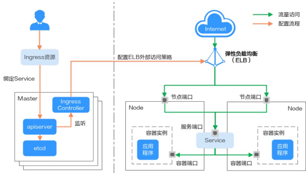
图 10-22 ELB Ingress 工作原理（CCE Standard 集群以及 CCE Turbo 集群使用共享型 ELB 场景）
