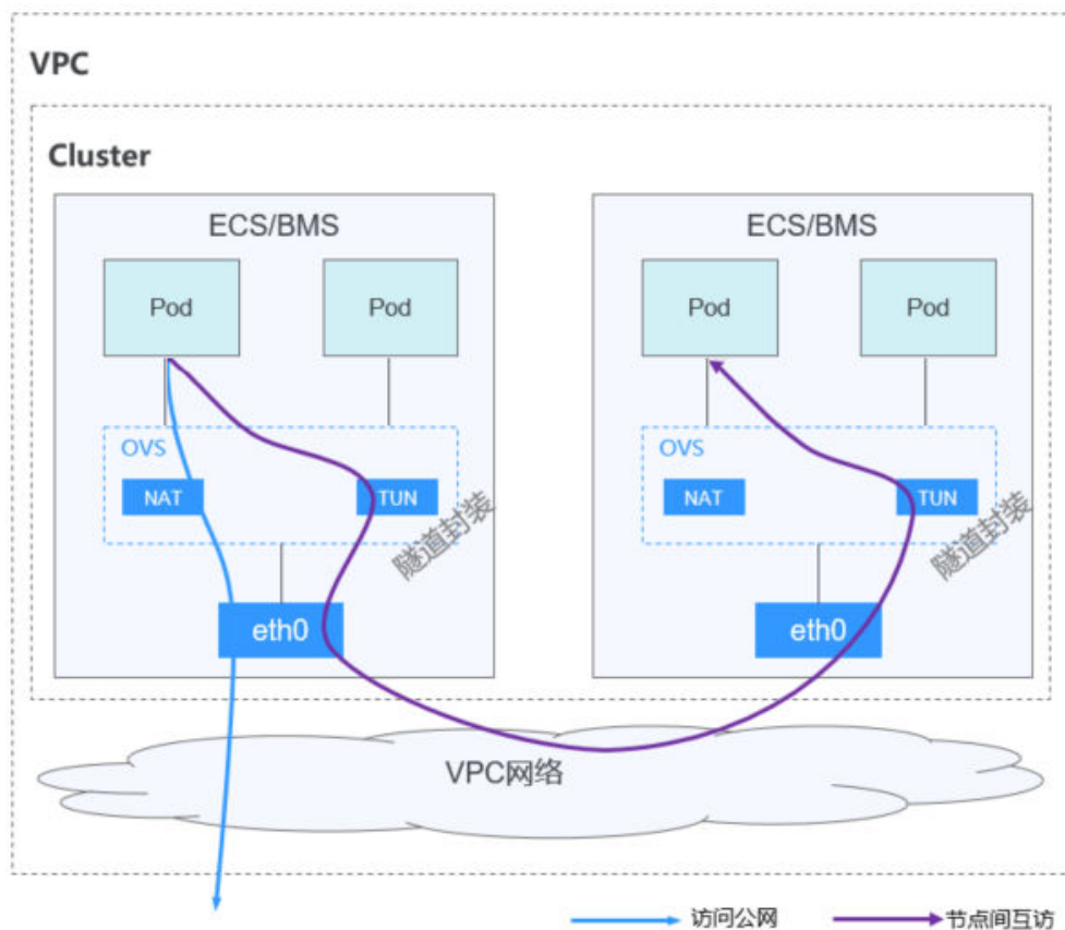
图 10-7 容器隧道网络
