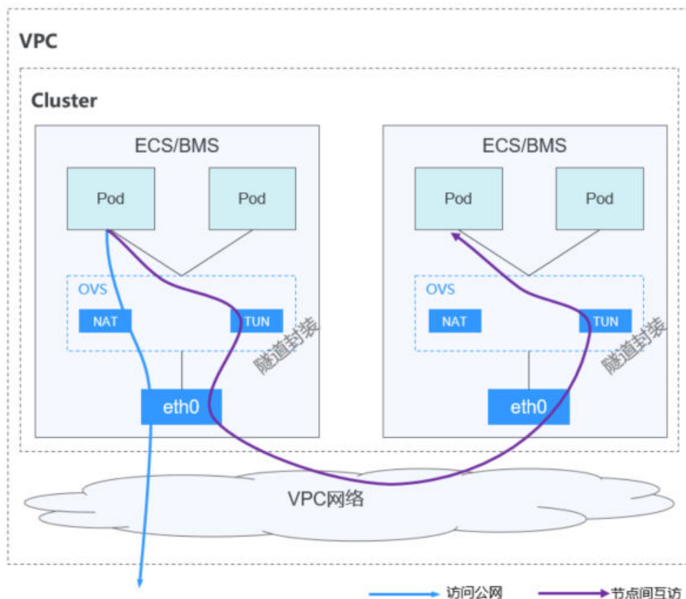
图 20-14 容器隧道网络
