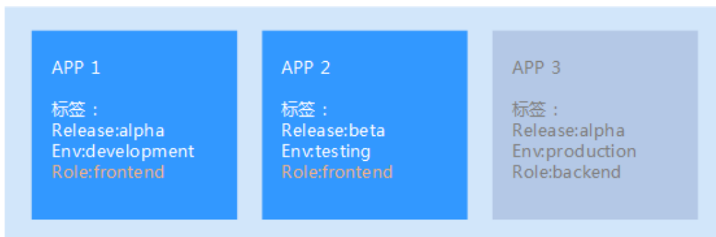
图 8-7 标签案例
