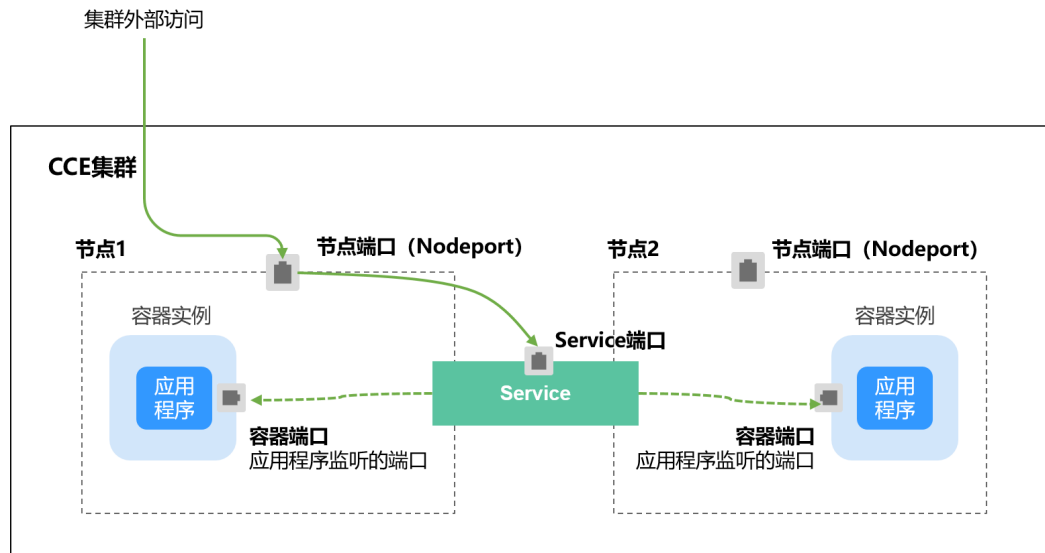
图 10-14 NodePort 访问
