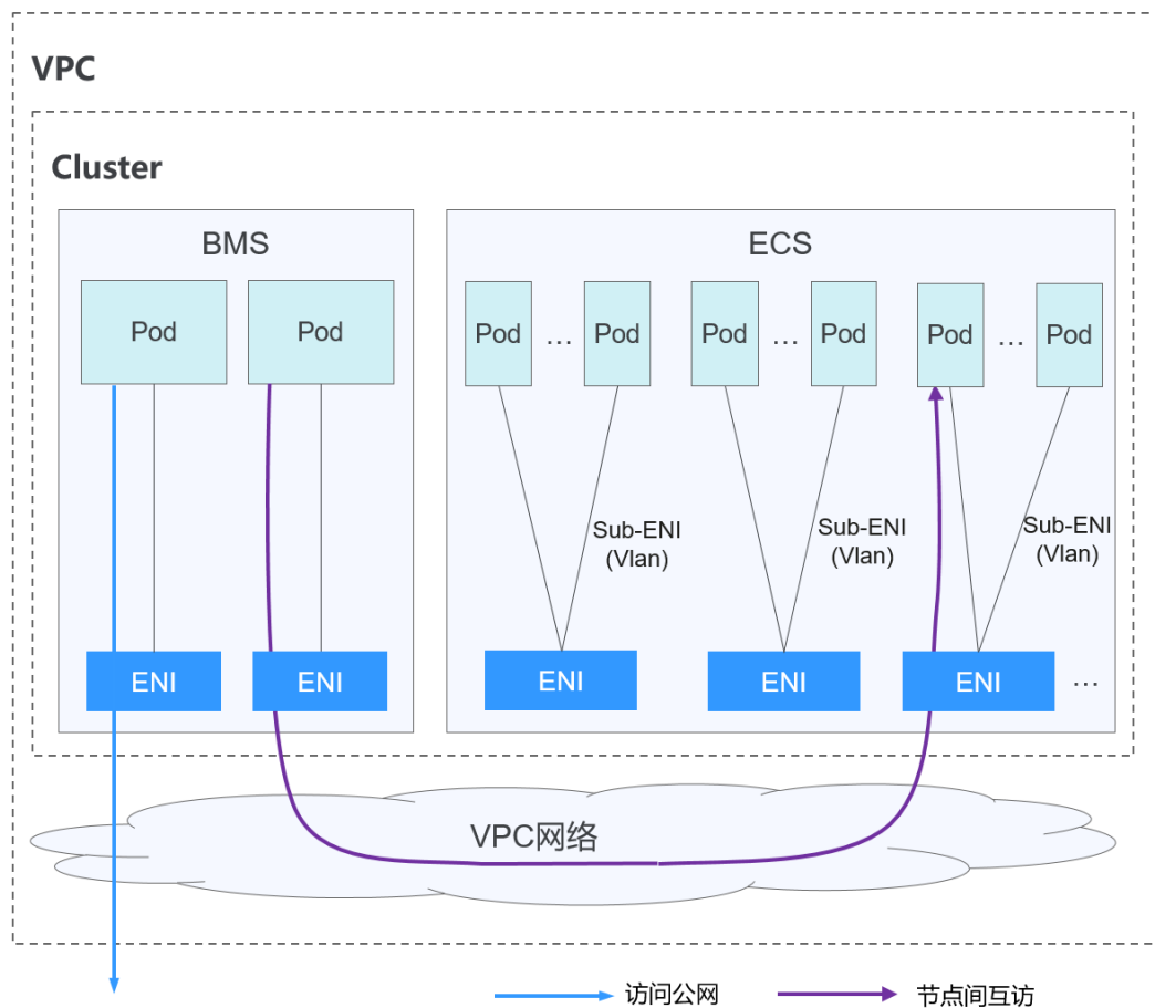
图 10-4 云原生网络 2.0
