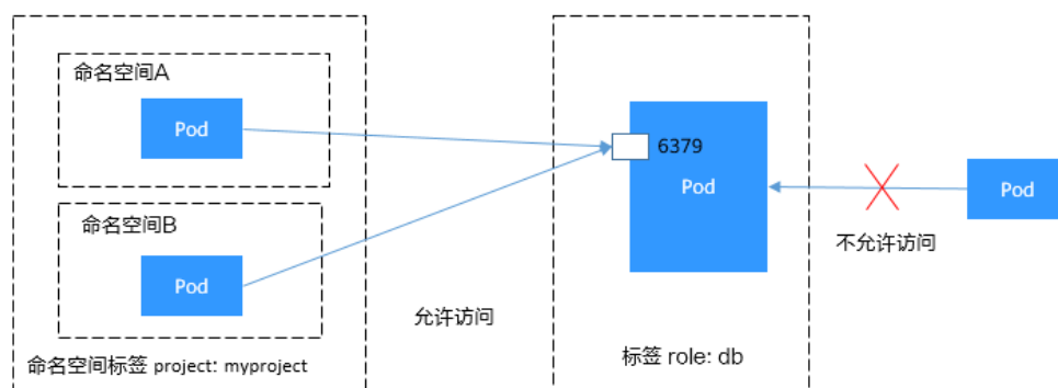
图 10-10 namespaceSelector
