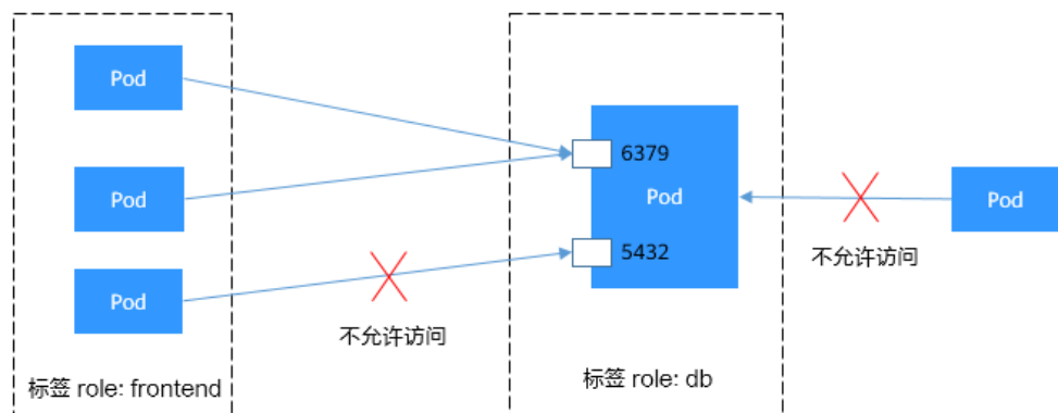
图 10-9 podSelector
