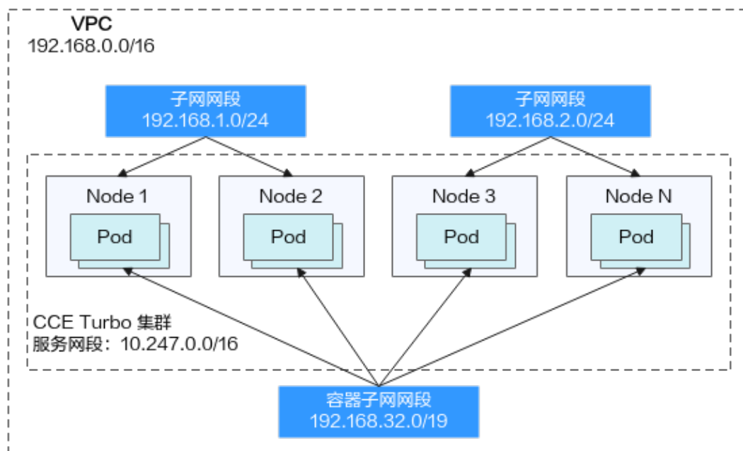
图 20-8 单 VPC 单集群场景网段规划-CCE Turbo 集群
