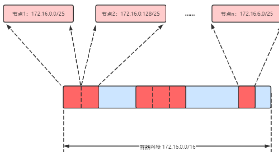
图 10-6 VPC 网络 IP 地址管理
