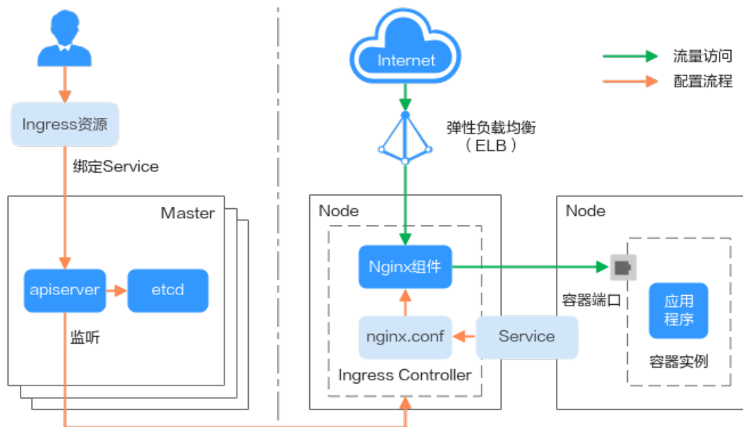
图 10-24 Nginx Ingress Controller 工作原理
