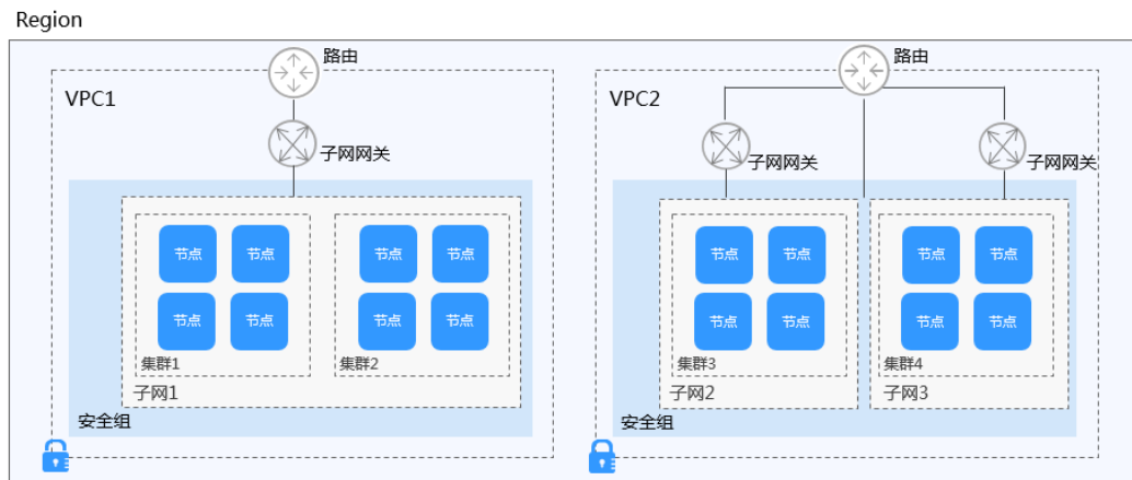
图 21-6 集群与 VPC、Subnet 的关系
