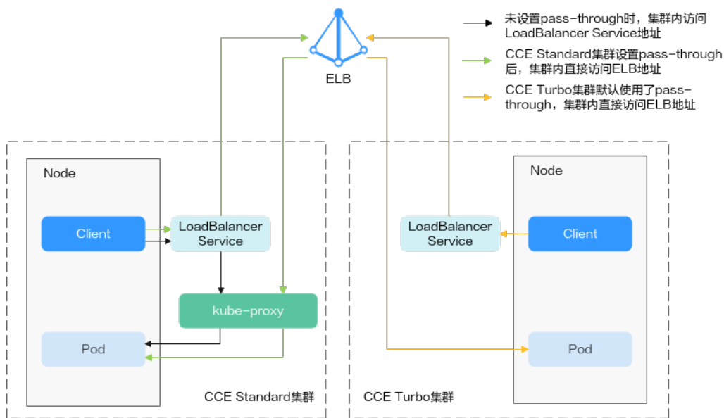
图 10-19 pass-through 访问示例
