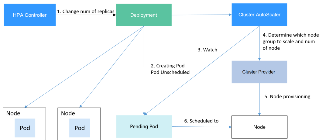
图 20-4 HPA + CA 工作流程
