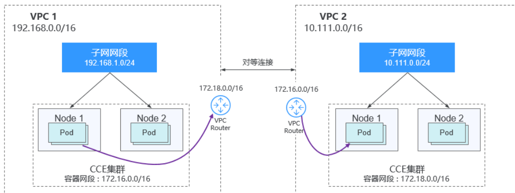
图 20-12 VPC 网络-VPC 互联场景
