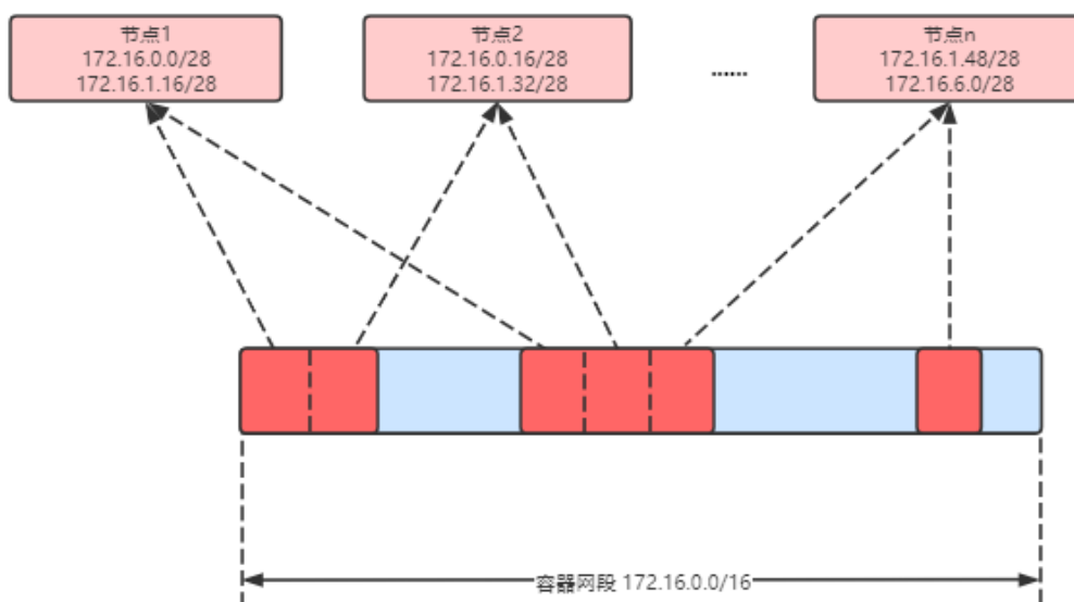
图 10-8 容器隧道网络 IP 地址分配
