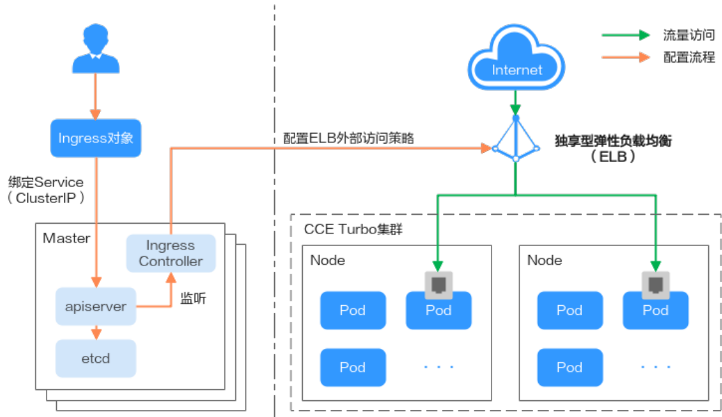
图 10-23 ELB Ingress 直通容器原理（CCE Turbo 集群使用独享型 ELB 场景）
