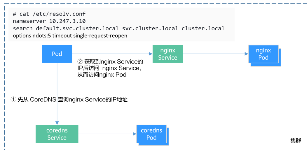
图 10-26 集群内域名解析示例图
