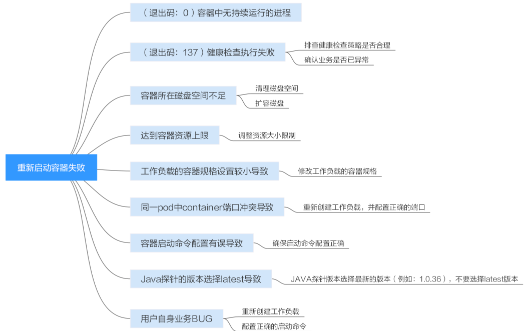
图 21-2 重新启动容器失败排查思路
