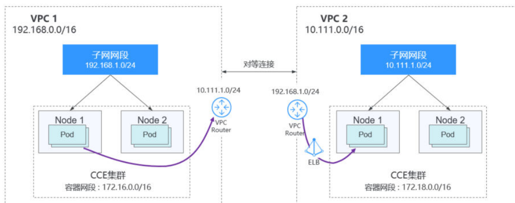
图 20-13 容器隧道网络-VPC 互联场景
