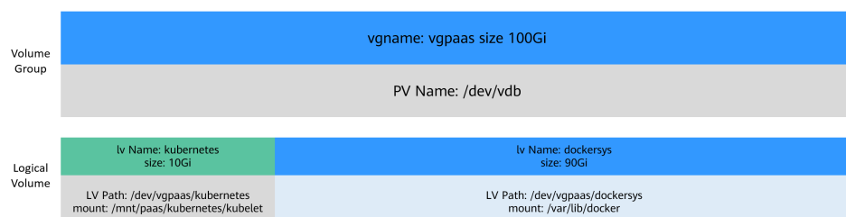
图 6-3 OverlayFS 类型容器引擎空间分配
