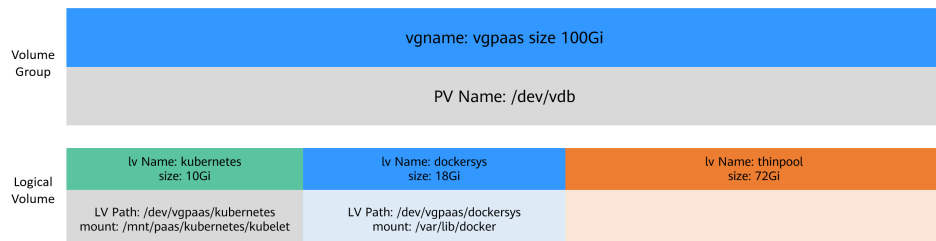
图 6-2 Device Mapper 类型容器引擎空间分配
