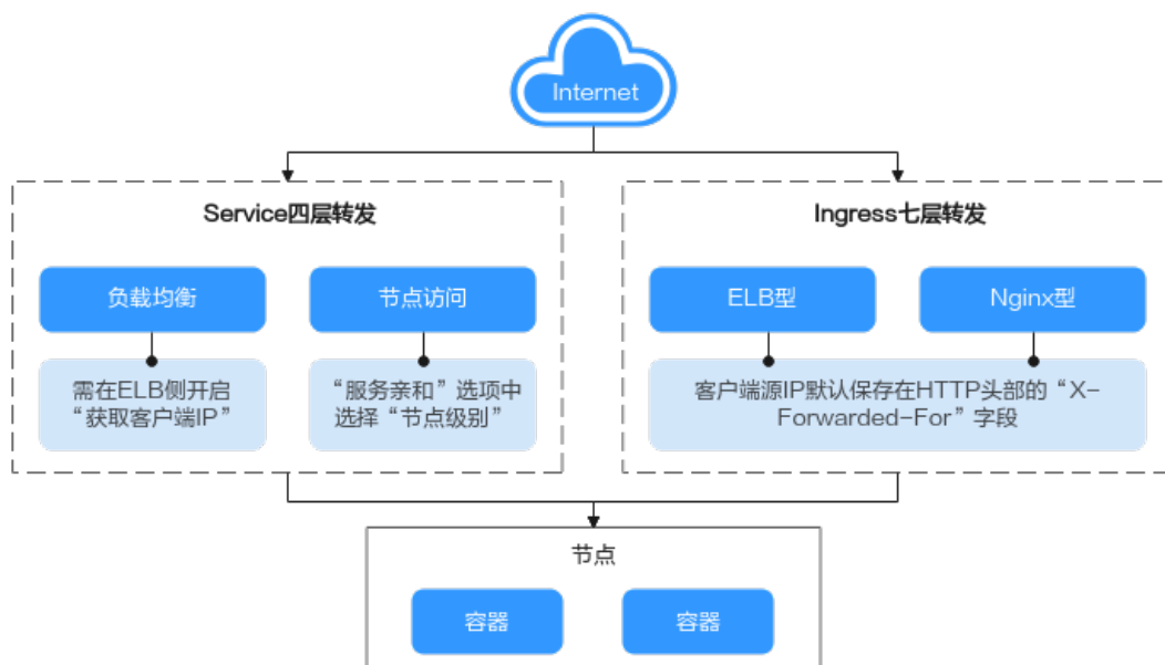
图 20-17 容器中获取源 IP
