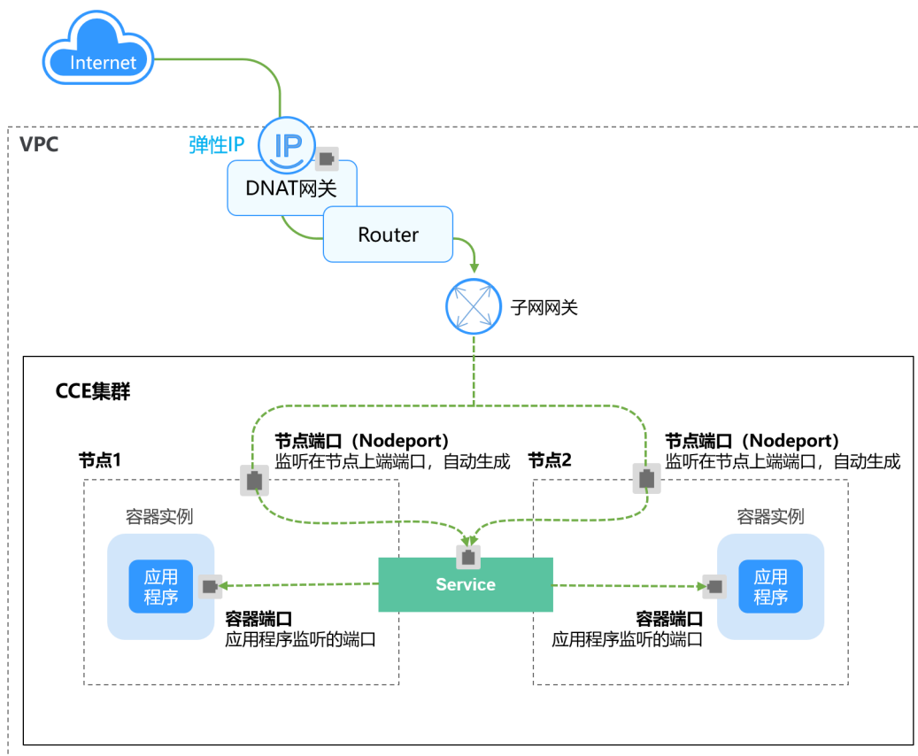
图 10-20 DNAT 网关 ( DNAT )
