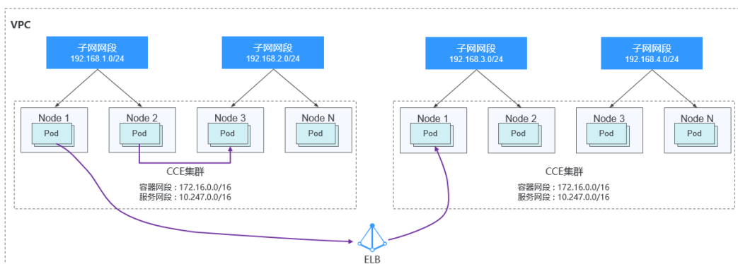
图 20-10 容器隧道网络-多集群场景示例
