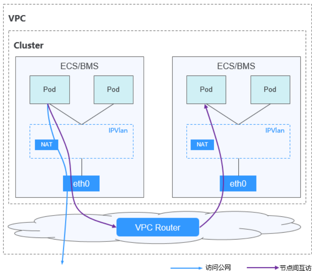
图 10-5 VPC 网络
