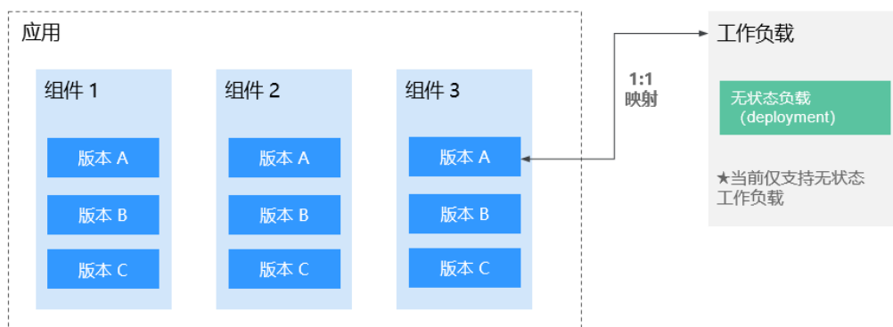
图 1-4 工作负载
