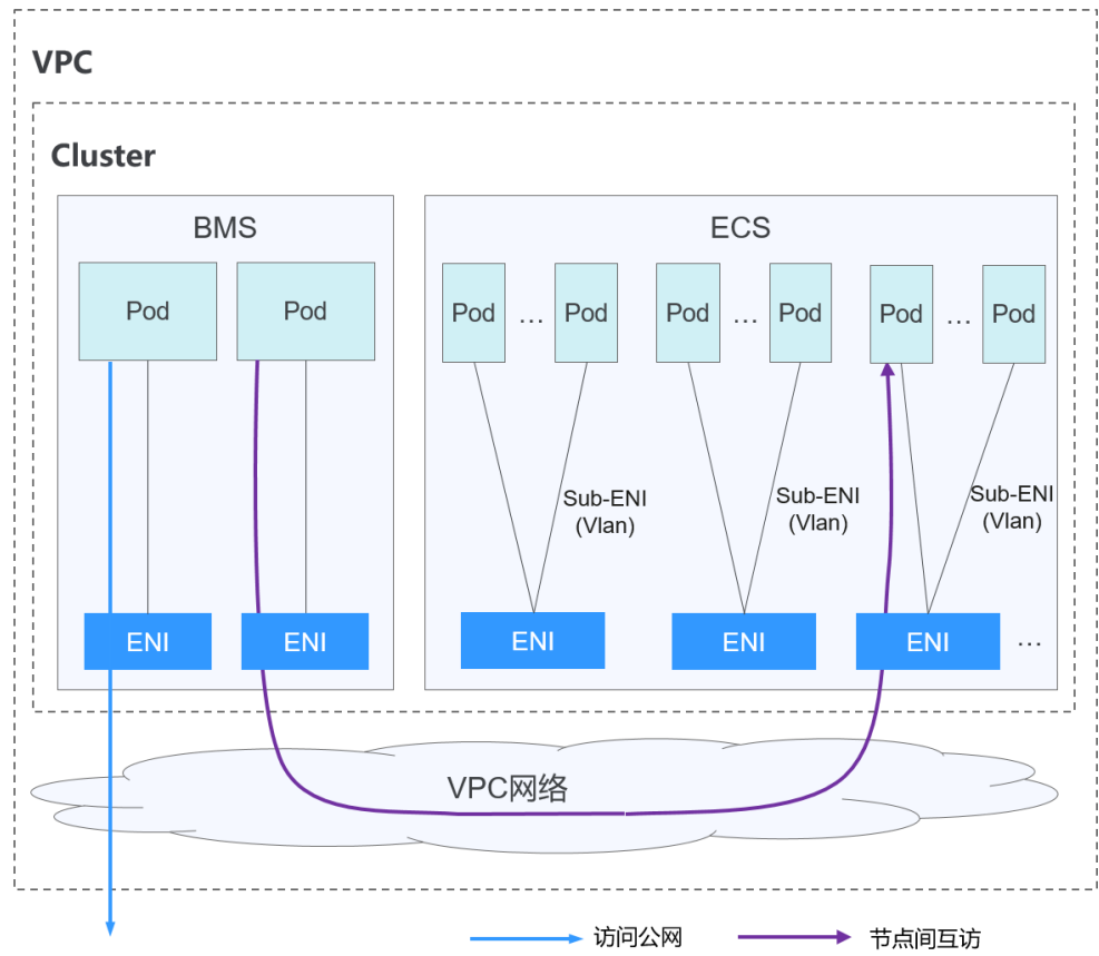
图 20-16 云原生网络 2.0
