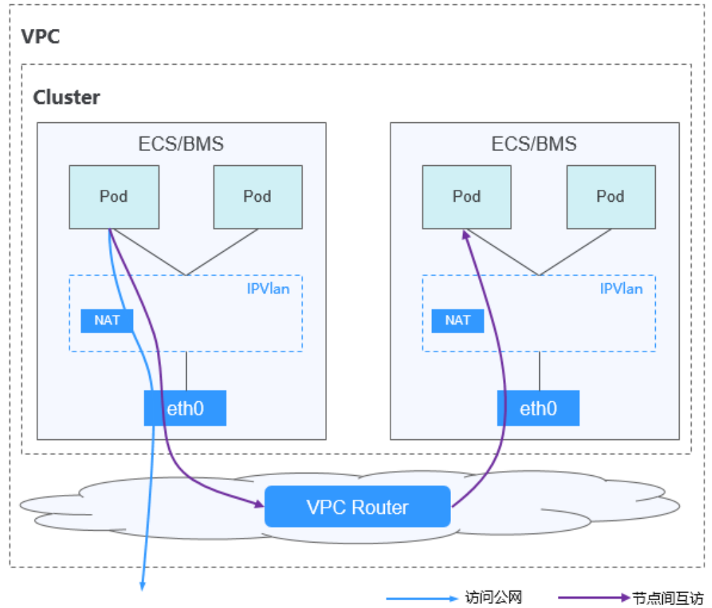
图 20-15 VPC 网络
