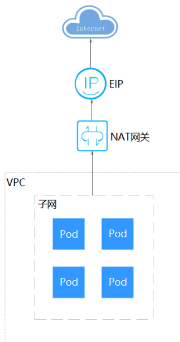
图 10-29 SNAT
