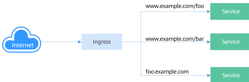
图 10-2 Ingress-Service
