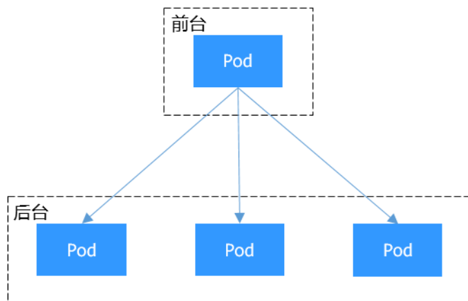
图 10-11 Pod 间访问
