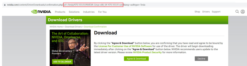
图 16-3 获取链接
