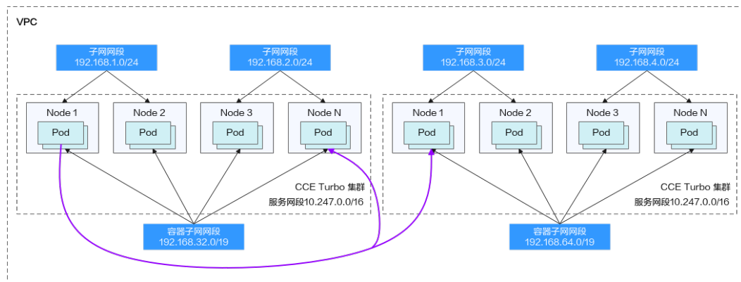
图 20-11 云原生网络 2.0-多集群场景示例
