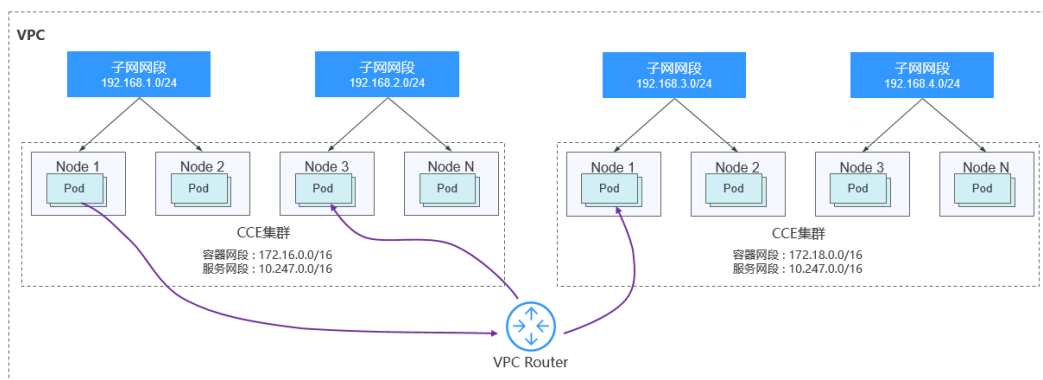
图 20-9 VPC 网络-多集群场景示例
