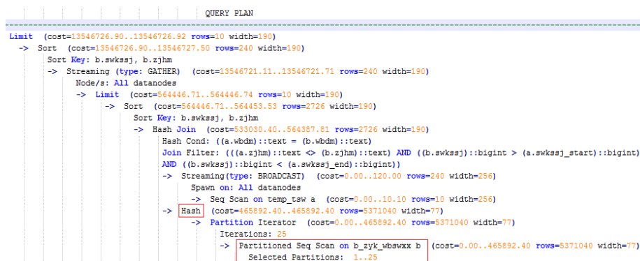
图 16-7 应用 unlogged table 案例（二）
