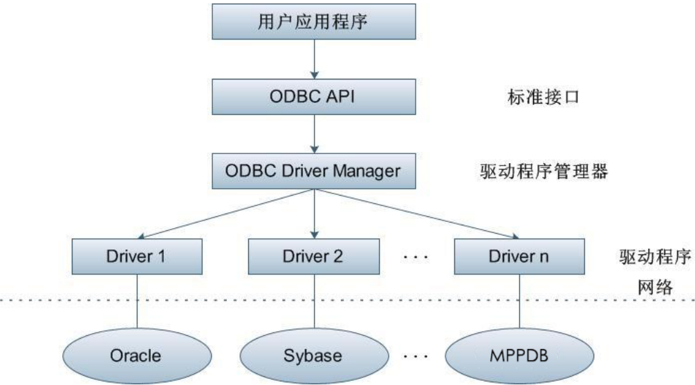
图 13-2 ODBC 系统结构
