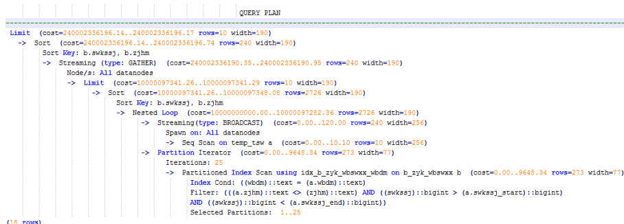
图 16-8 应用 unlogged table 案例（三）
