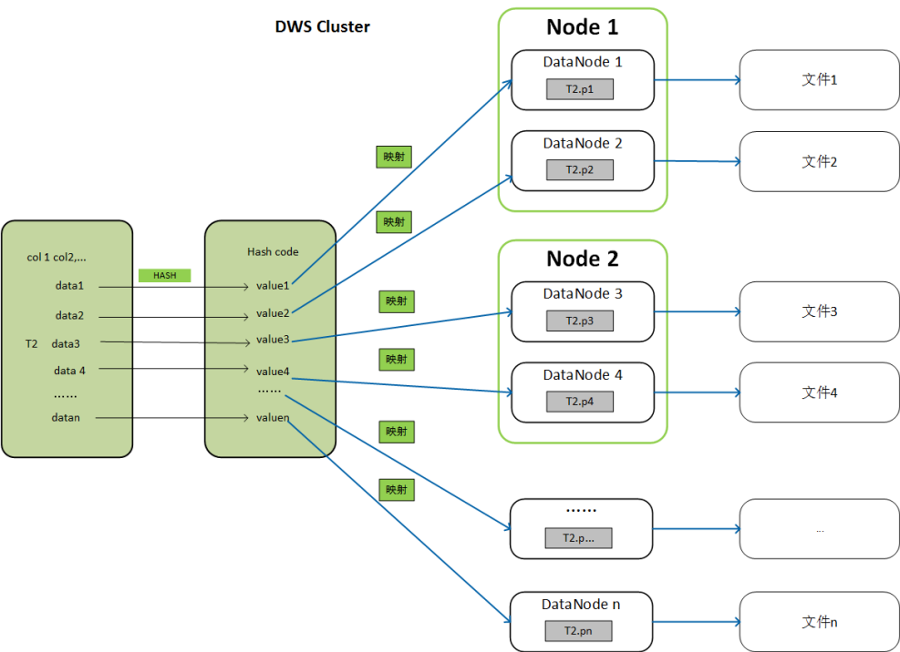
图 2-8 Hash 分布原理
