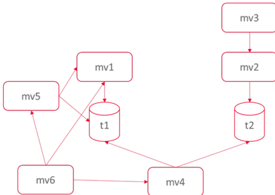
图 9-1 嵌套物化视图依赖关系
