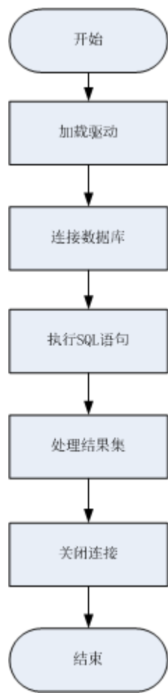
图 13-1 采用 JDBC 开发应用程序的流程
