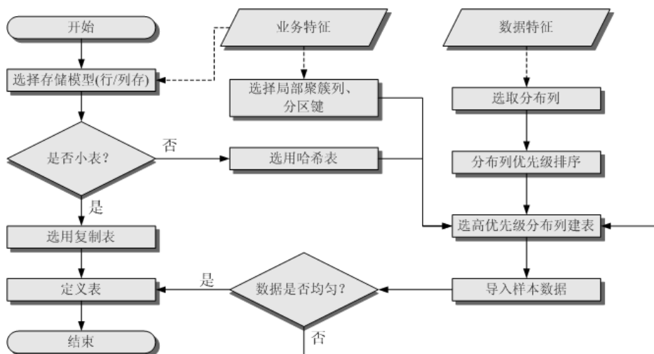
图 16-5 表定义流程
