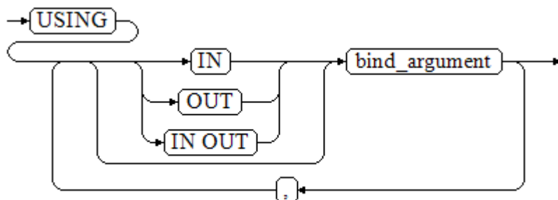
图 11-12 using_clause-3
