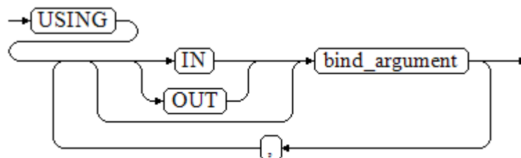
图 11-7 using_clause-1
