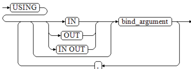
图 11-14 using_clause-4
