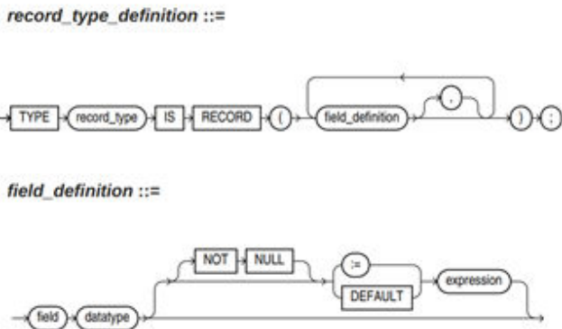
图 11-1 record 类型的语法
