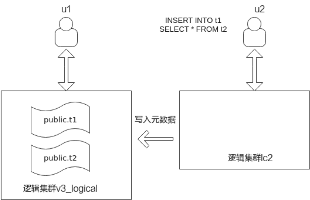
图 7-2 跨逻辑集群实现数据写入
