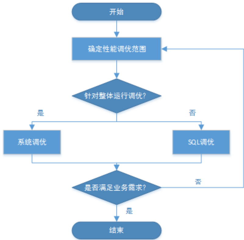
图 16-1 DWS 性能调优流程
