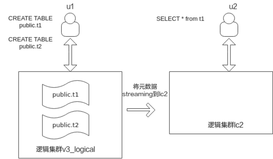
图 7-1 跨逻辑集群实现数据查询
