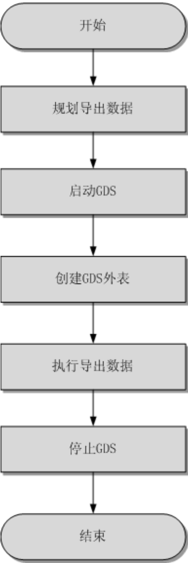
图 2-11 并行导出流程
