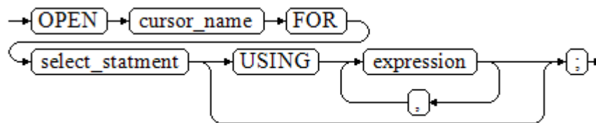
图 11-30 open_dynamic_cursor::=
