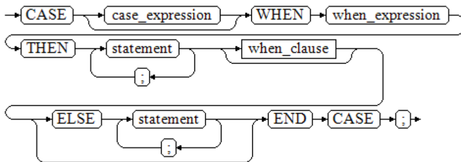
图 11-24 case_when::=
