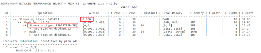
图 16-19 选择合适的分布列案例（一）
