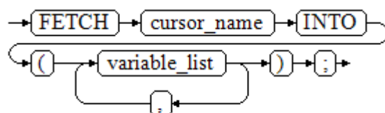
图 11-31 fetch_cursor::=
