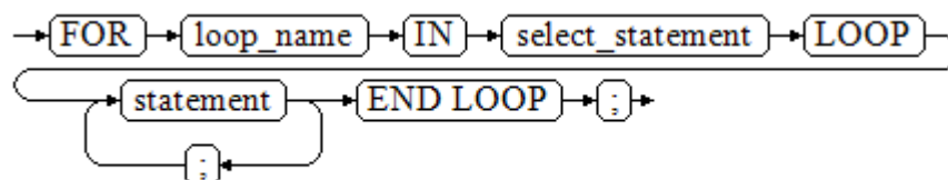
图 11-33 FOR_AS_loop::=
