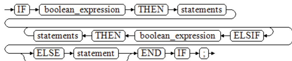
图 11-18 IF_THEN_ELSE IF::=
