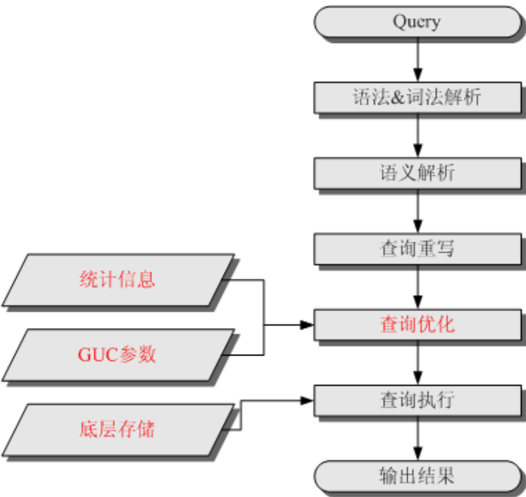
图 16-2 SQL 引擎执行查询类 SQL 语句的流程
