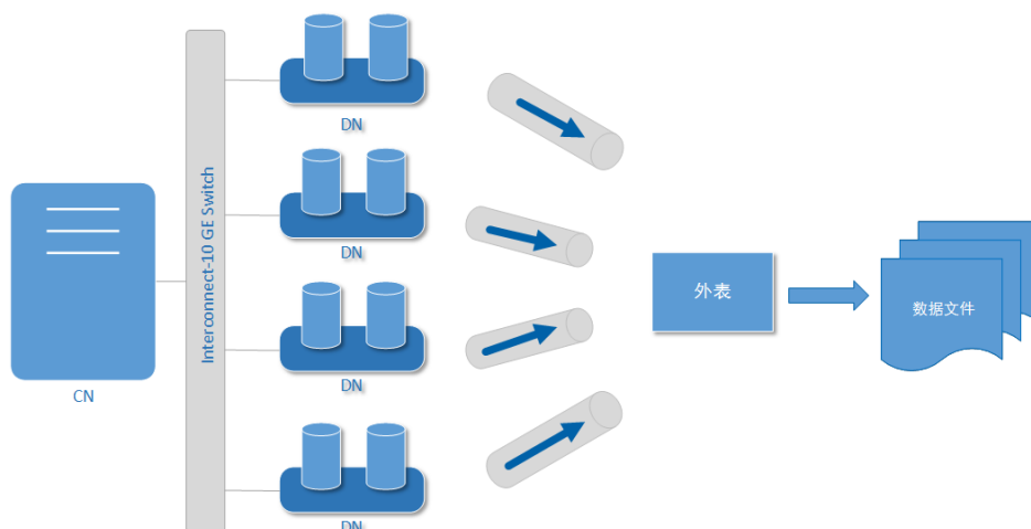
图 2-10 通过外表导出数据
