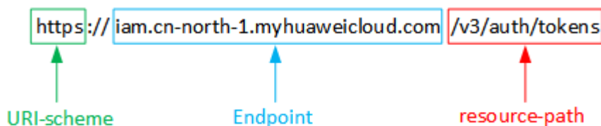
Figura 5-1 Exemplo de URI
