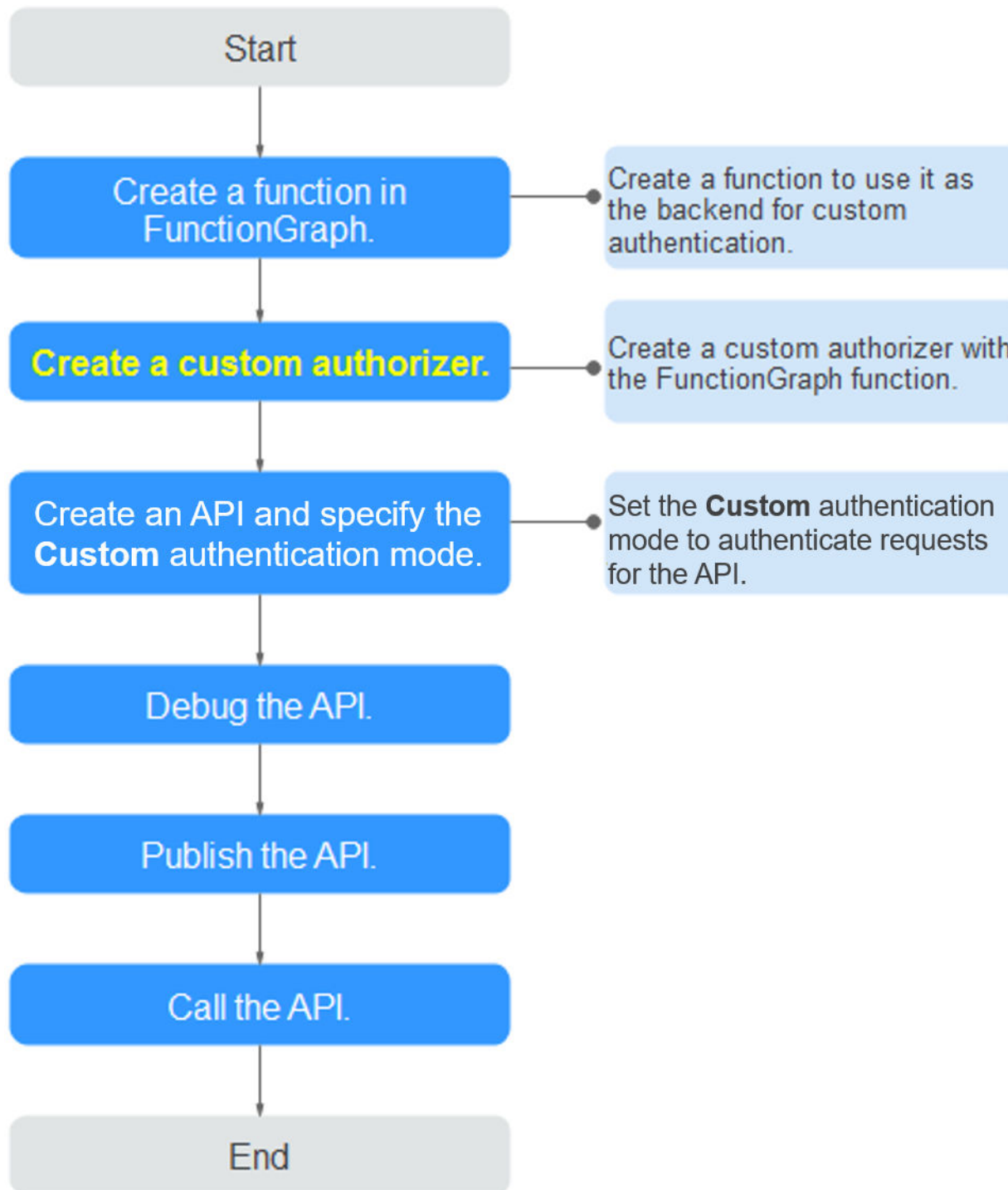
Figura 3-30 Llamar a las API mediante autenticación personalizada
