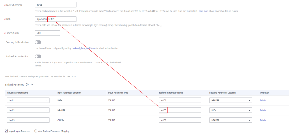
Figura 3-4 Configuración de parámetros de backend
