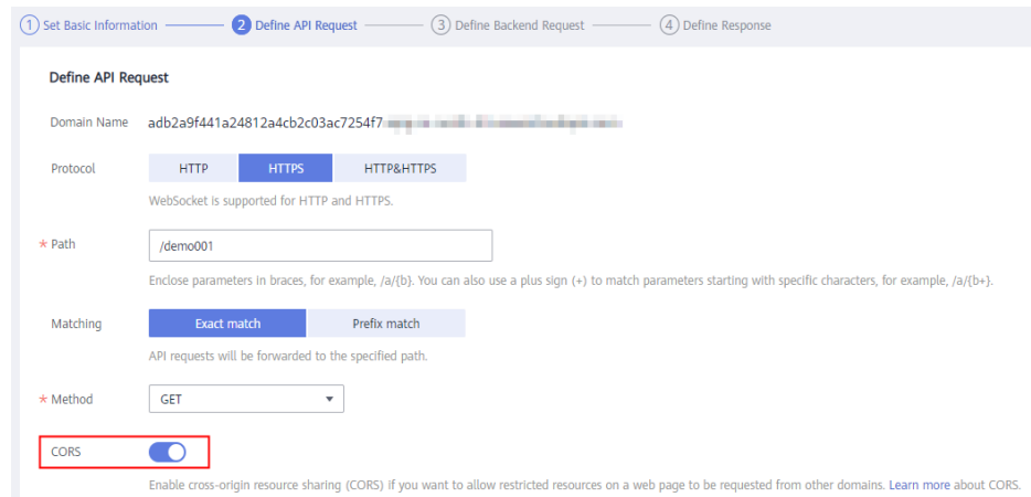
Figura 3-8 CORS
