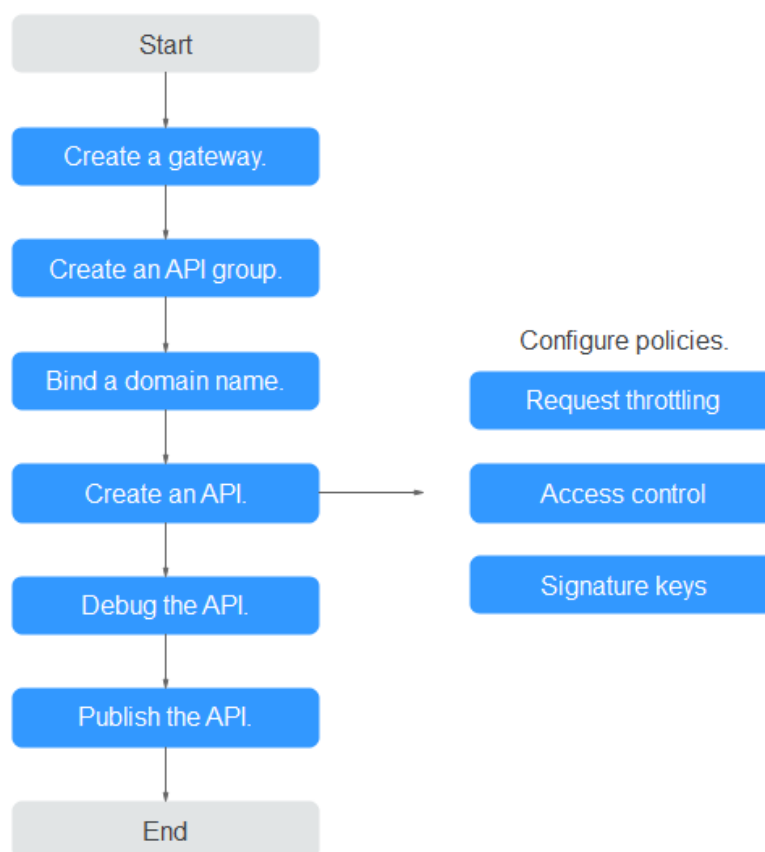
Figura 1-2 Proceso de API opening
