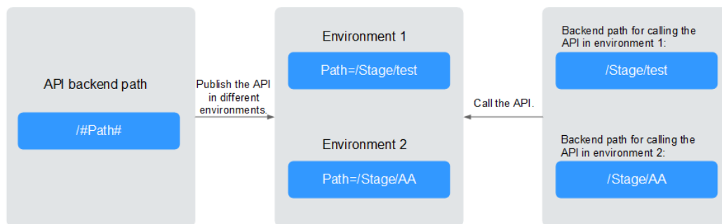
Figura 3-24 Uso de variables de entorno
