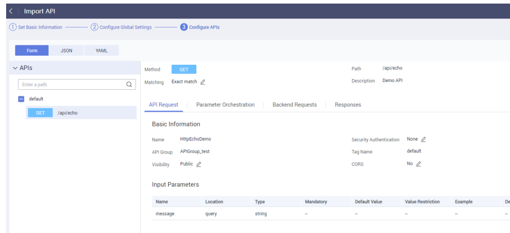
Figura 3-18 Modificación de APIs
