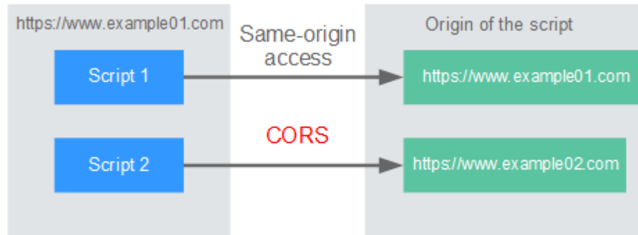
Figura 3-7 Flujo de proceso del mecanismo CORS
