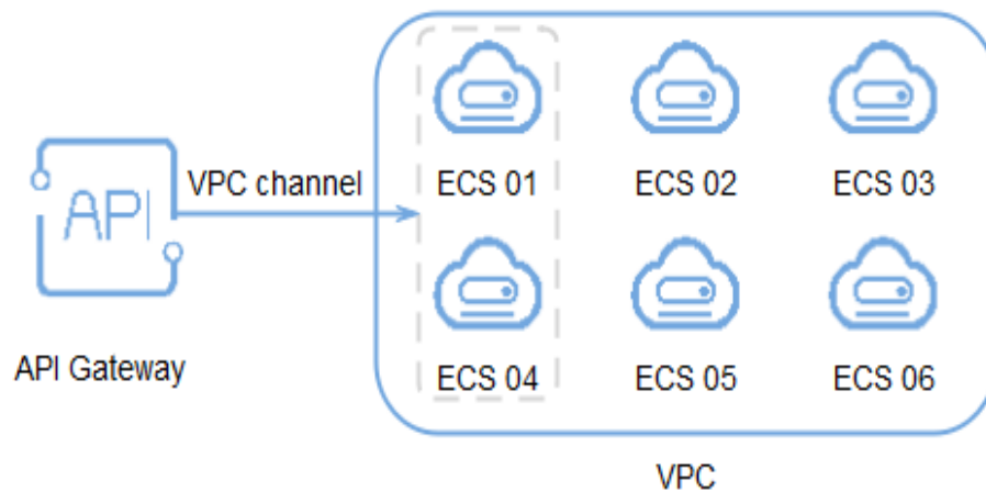
Figura 3-28 Acceso a ECS en un canal de VPC a través de API Gateway
