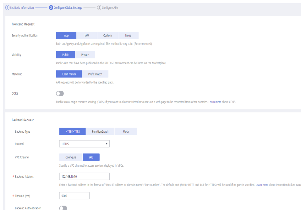
Figura 3-17 Configuración de la ajuste global
