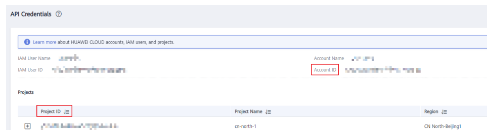
Figura 3-22 Ver el ID de cuenta y el ID de proyecto
