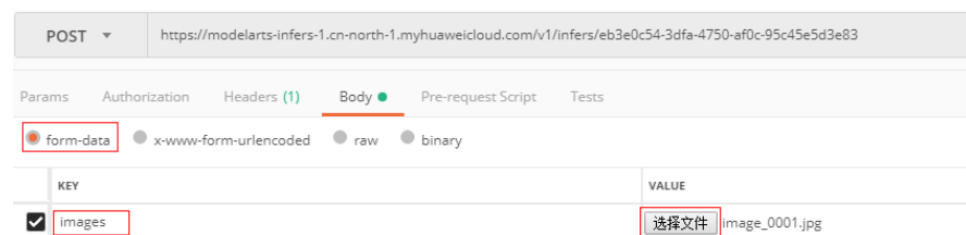
图 3-13 填写 Body
