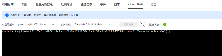
图 3-40 CloudShell 界面
