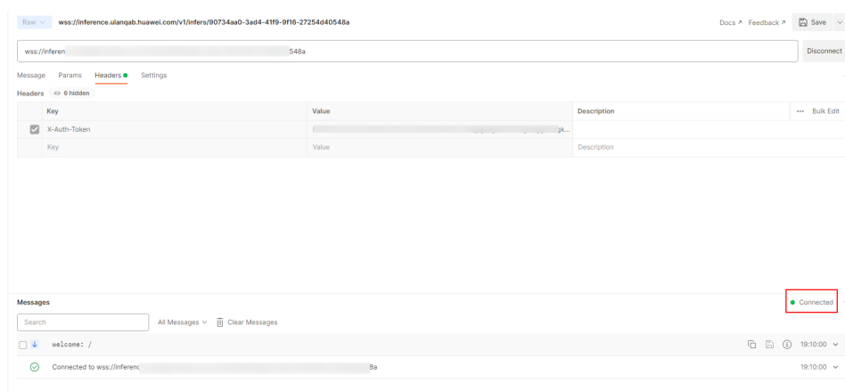
图 3-36 连接成功
