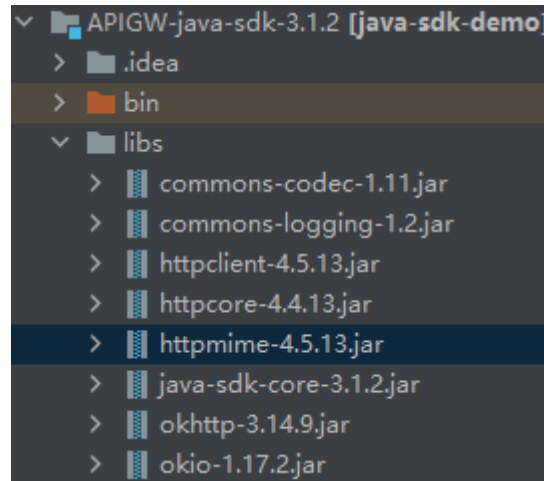
图 3-25 Java 依赖库
