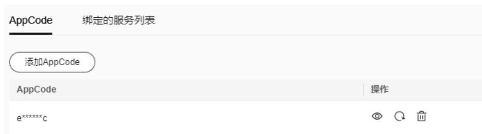
图 3-23 添加 AppCode
