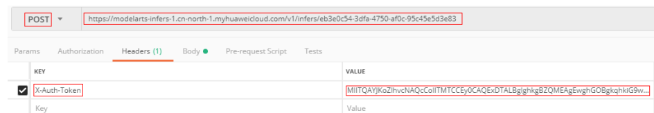
图 3-12 参数填写
