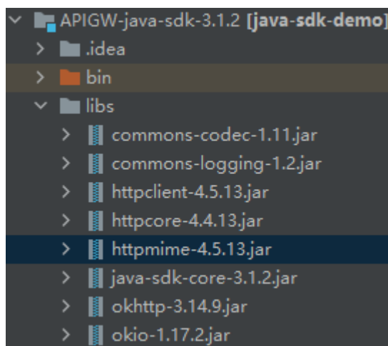
图 3-16 Java 依赖库
