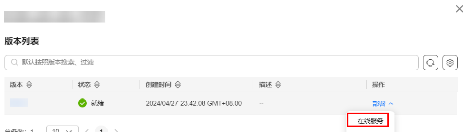
图 2-10 部署模型
