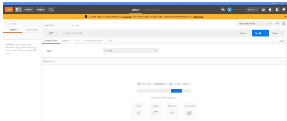
图 3-11 Postman 界面
