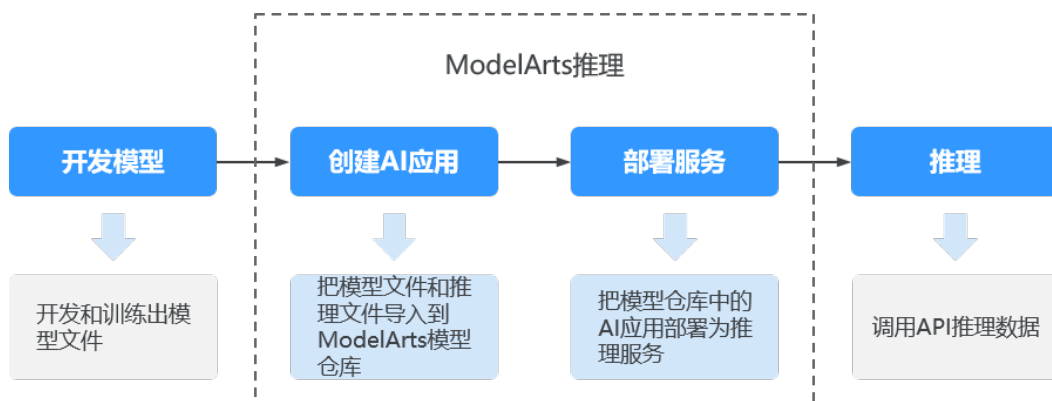
图 1-1 推理简介
