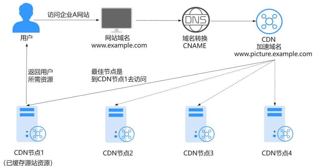
图 3-4 网站使用华为云 CDN 加速
