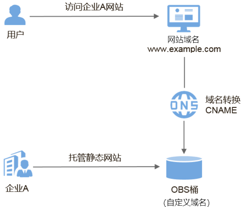
图 3-3 OBS 托管静态网站
