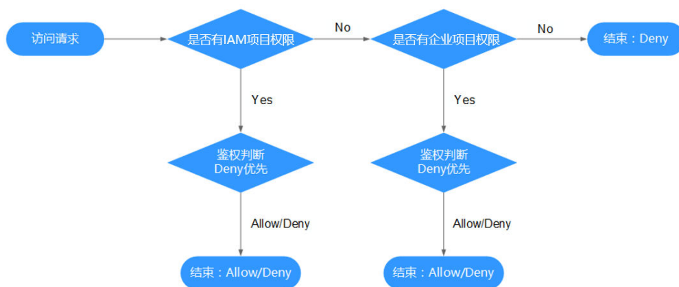
图 5-1 请求鉴权逻辑图
