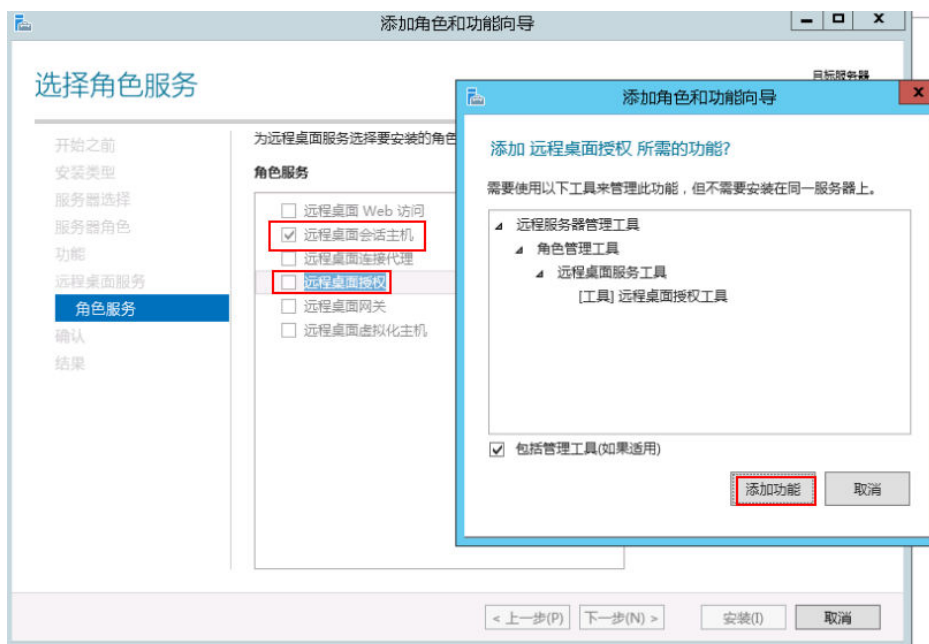
图 1-36 添加功能
