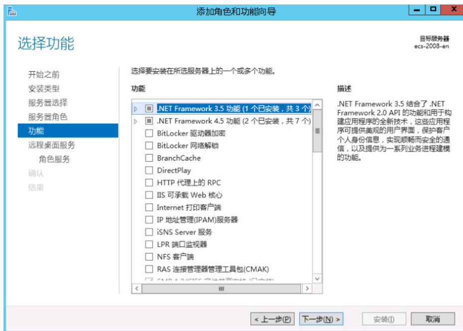
图 1-35 功能页面
