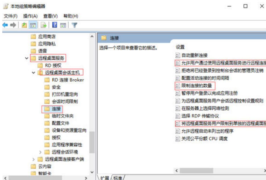
图 1-41 设置“连接”
