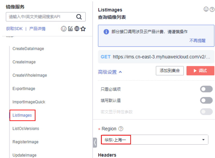
图 1-1 设置区域
