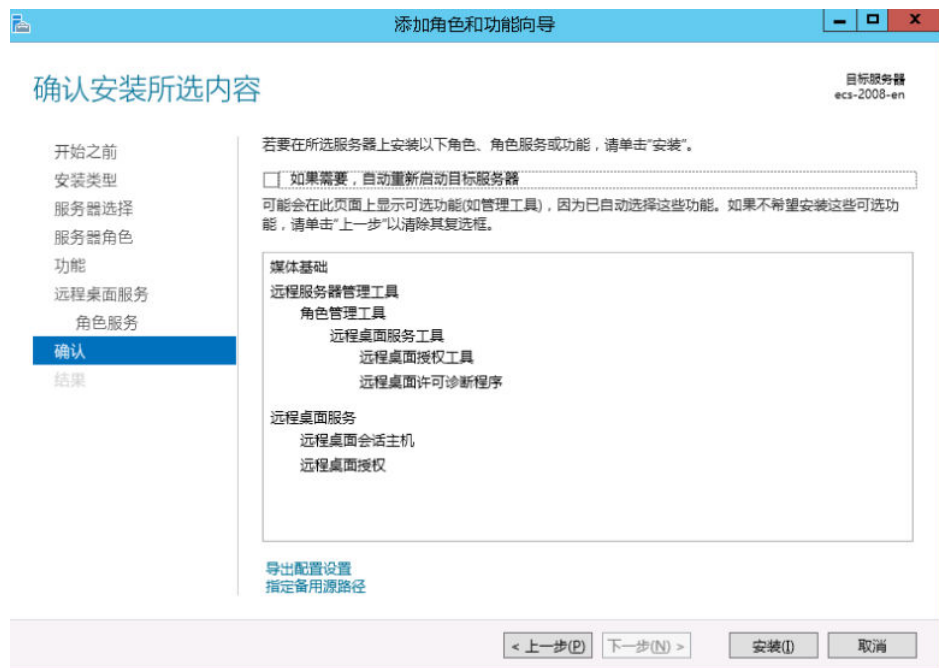
图 1-38 安装
