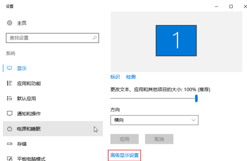
图 1-28 设置
