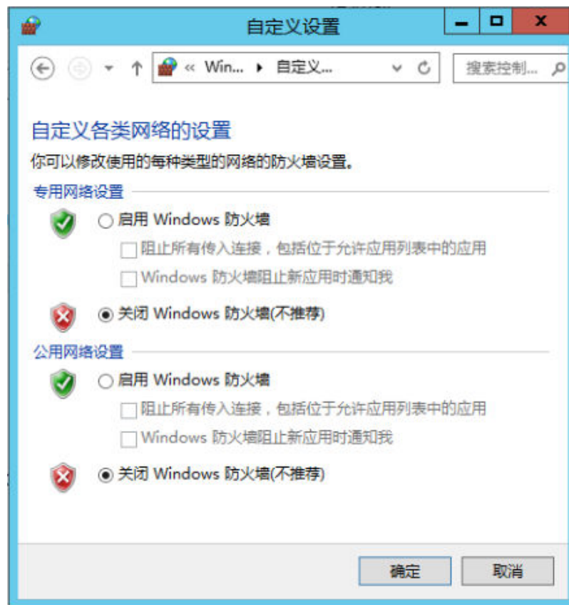
图 1-16 关闭防火墙
