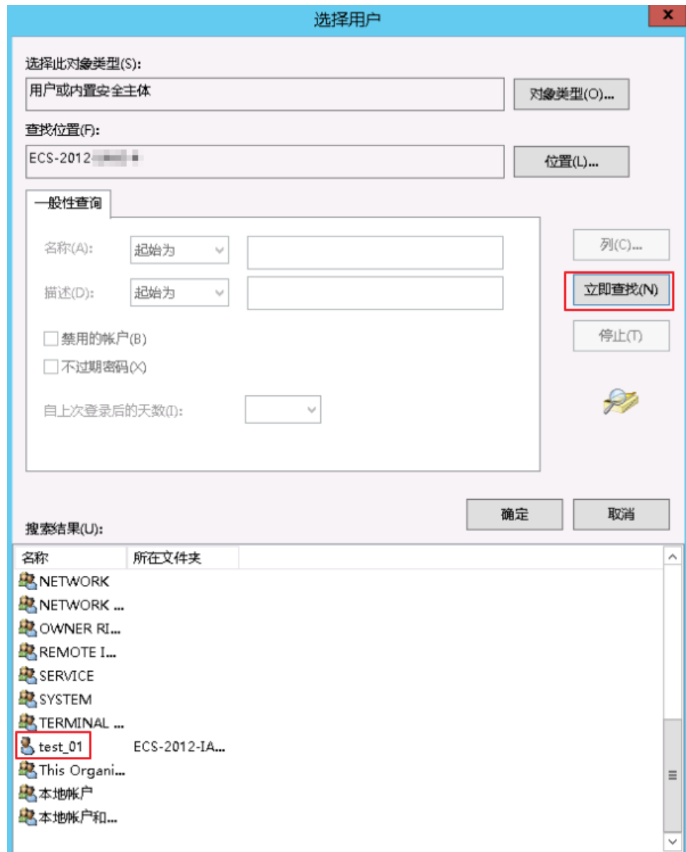
图 1-50 选择用户
