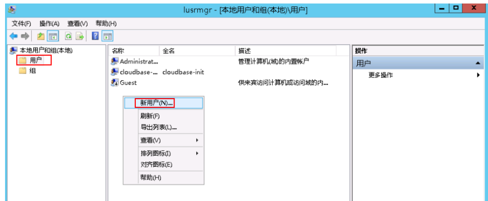
图 1-46 选择新用户
