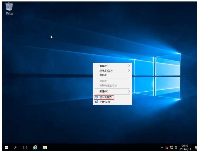
图 1-27 显示设置
