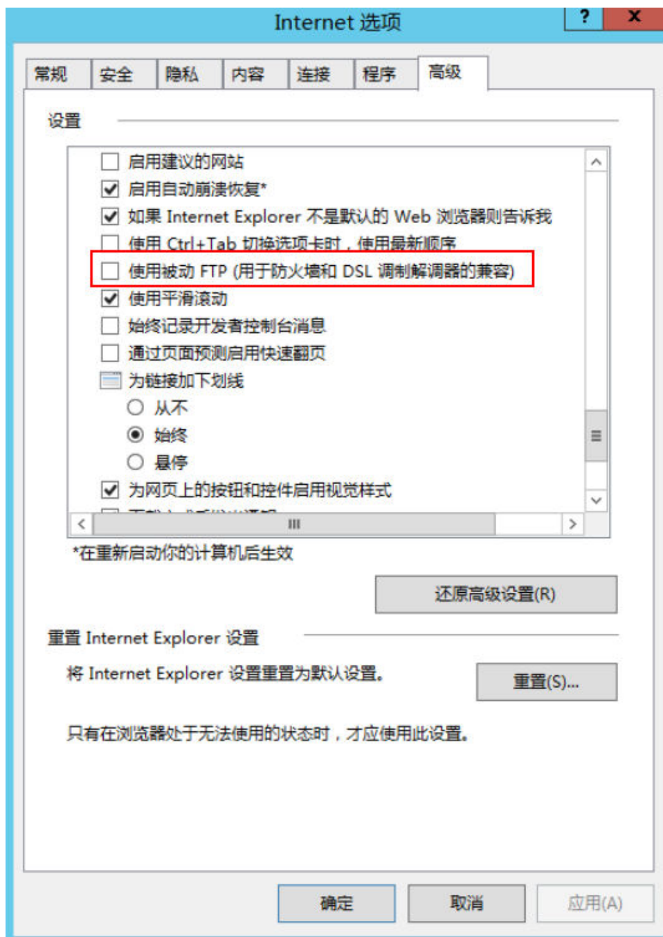
图 1-99 Internet 选项
