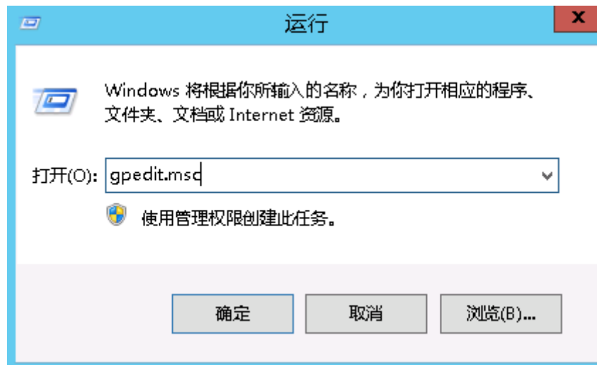
图 1-40 gpedit.msc
