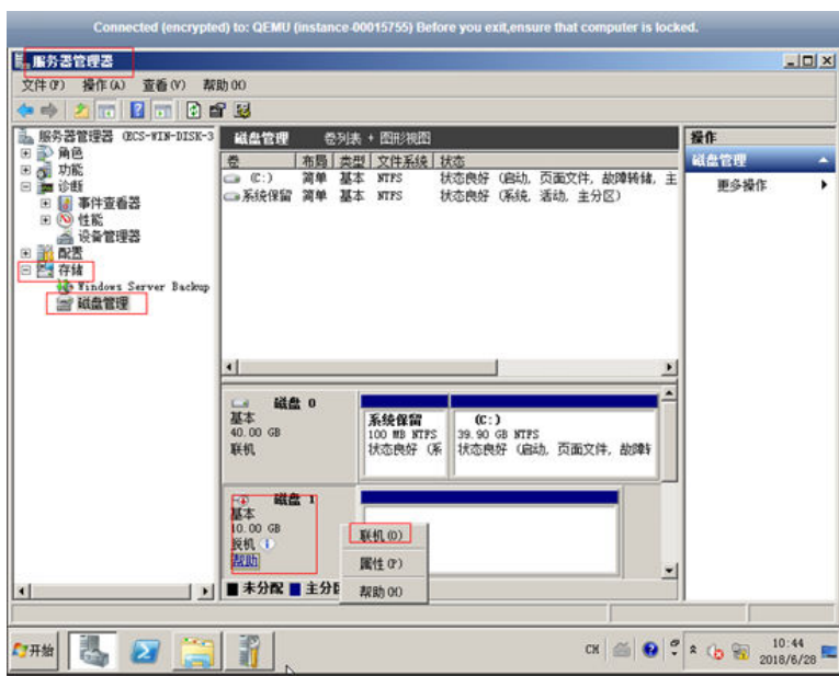
图 1-105 联机
