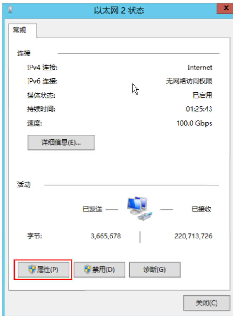
图 1-76 本地连接
