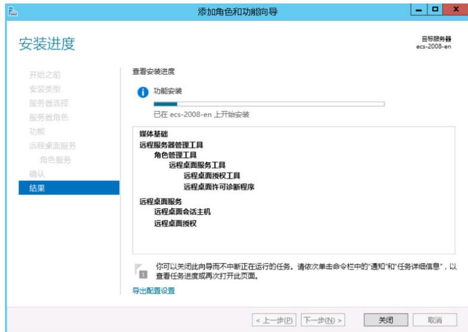
图 1-39 功能安装
