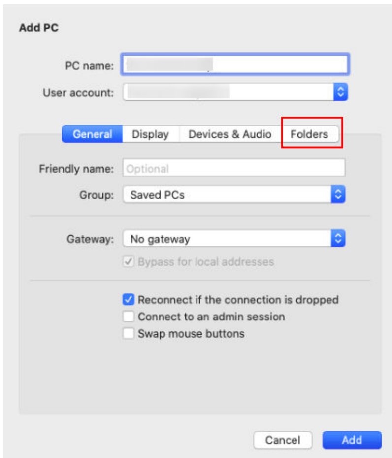
图 1-83 Add PC
