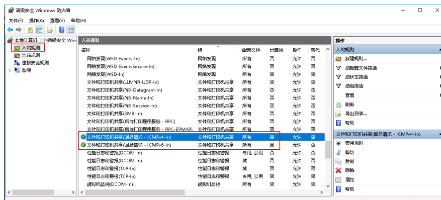
图 1-58 进站规则
