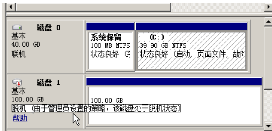
图 1-102 磁盘脱机
