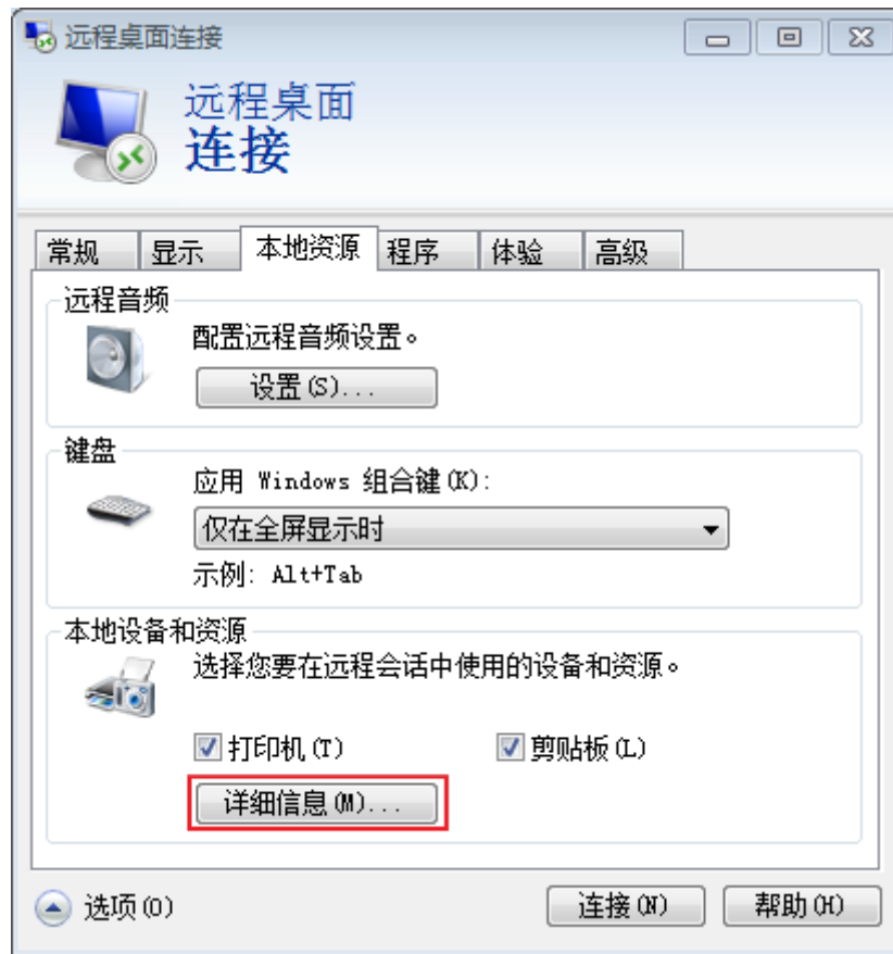
图 1-91 本地资源
