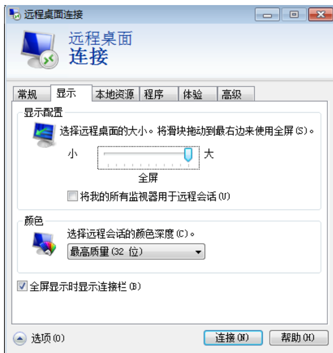
图 1-31 显示
