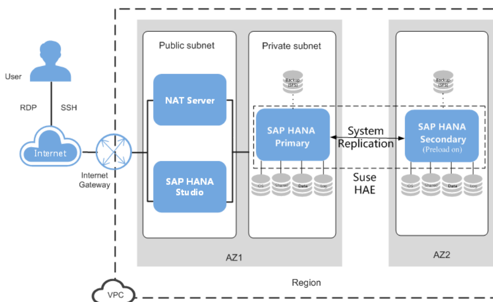
图 5-4 跨 AZ 部署 SAP HANA 高可用
