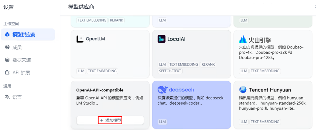
图 3-31 选择供应商
