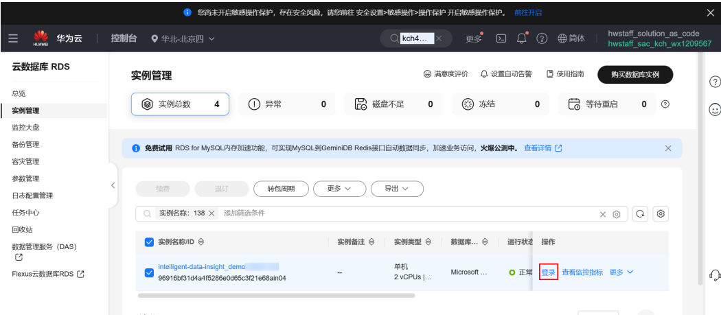
图 3-39 登录数据库
