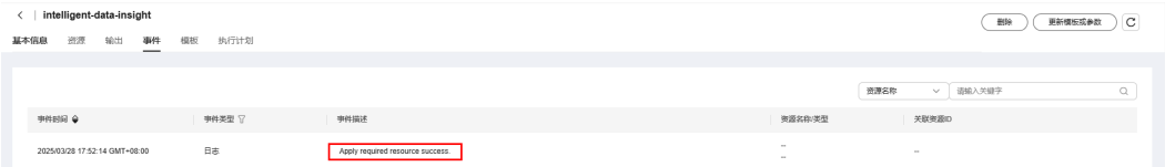
图 3-17 部署完成
