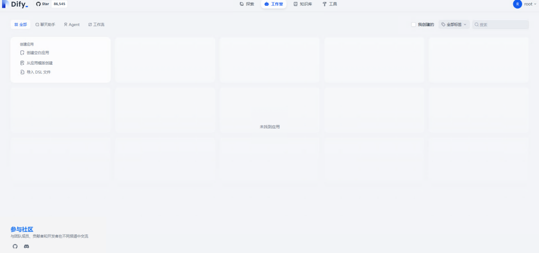
图 3-30 Dify 平台
