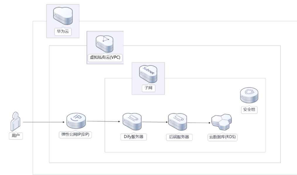
图 1-1 方案架构图
