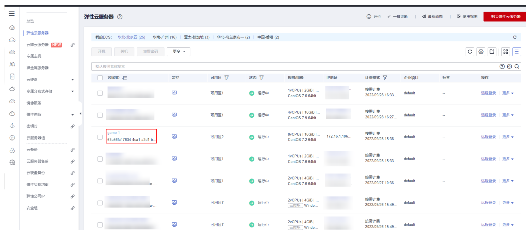
图 3-17 ECS 控制台
