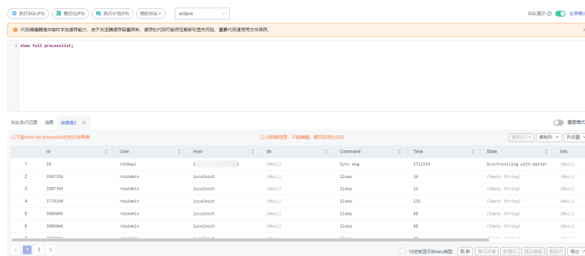
图 3-8 查询线程
