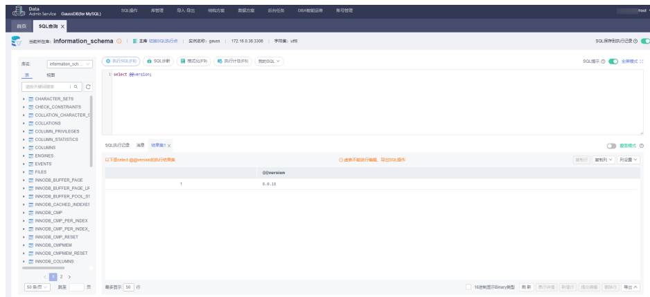
图 12-2 查看版本号
