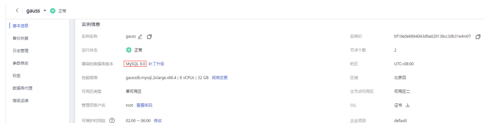
图 12-1 基本信息
