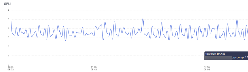
图 6-1 CPU 使用率
