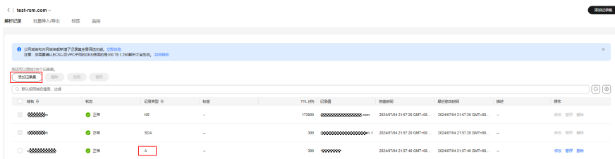
图 3-2 添加记录集
