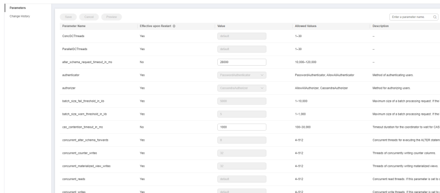
Figure 3-71 Modifying parameters in a parameter template
