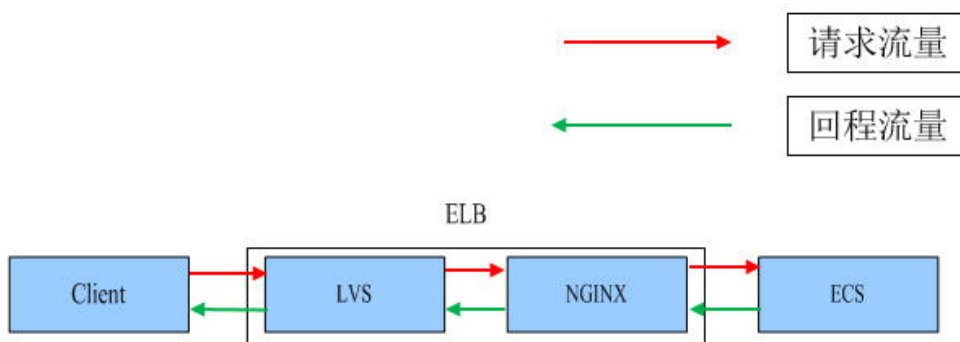
图 5-5 七层转发协议
