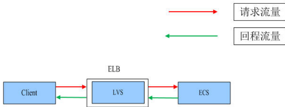
图 5-1 四层转发协议
