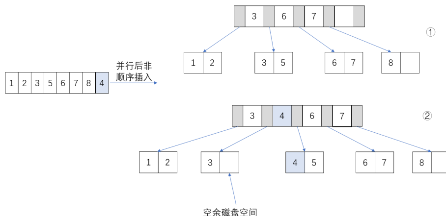
图 1-18 并行非顺序插入
