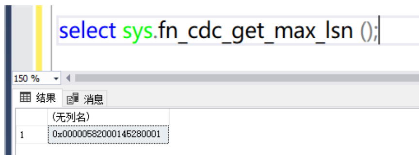
图 6-4 查询 lsn
