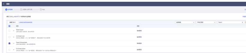
图 3-2 选择策略
