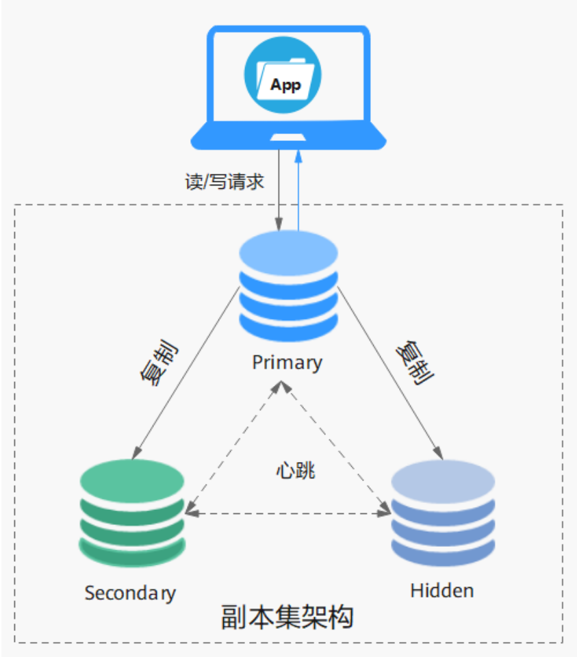
图 4-2 副本集
