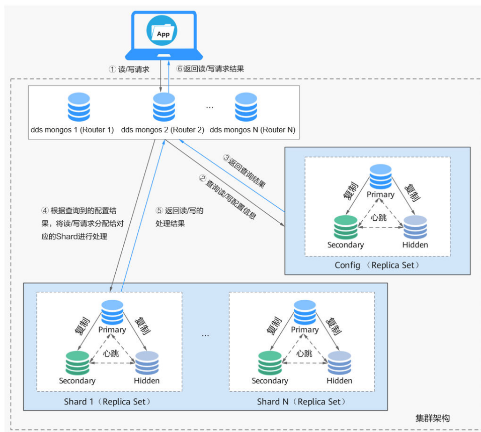
图 4-1 集群
