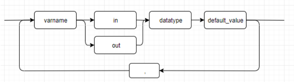
图 2-43 parameter 格式使用参考图
