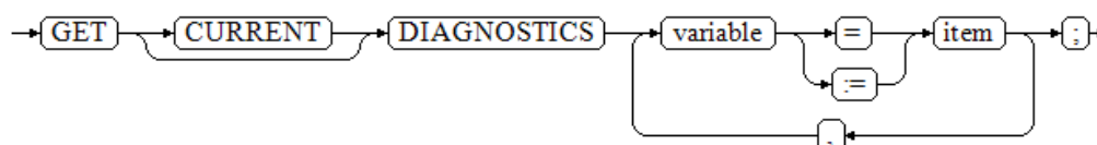
图 2-38 获取当前执行信息语法
