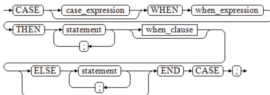
图 2-35 case_when::=
