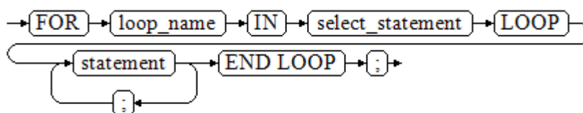
图 2-50 FOR_AS_loop::=
