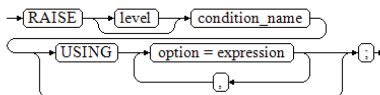
图 2-52 raise_condition::=
