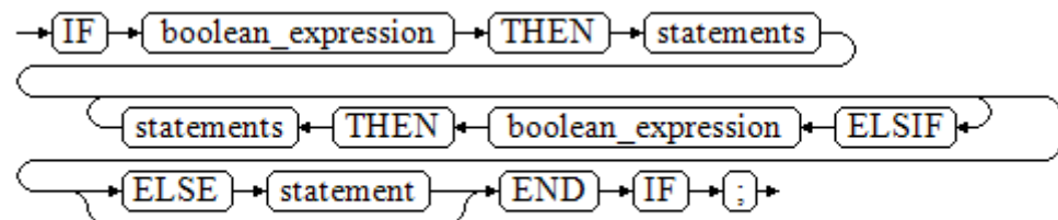
图 2-24 IF_THEN_ELSEIF_ELSE::=
