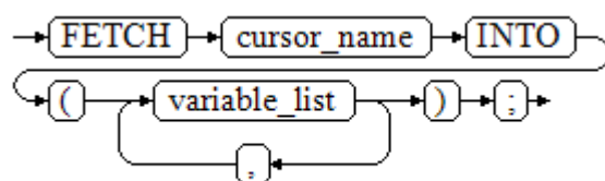
图 2-48 fetch_cursor::=
