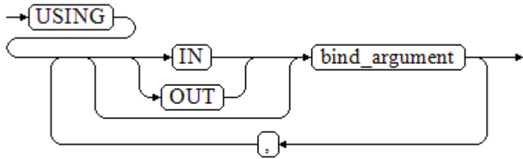
图 2-11 using_clause::=
