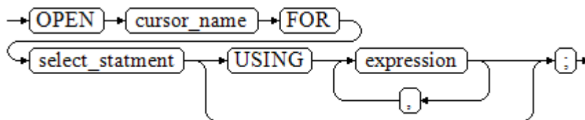
图 2-47 open_dynamic_cursor::=
