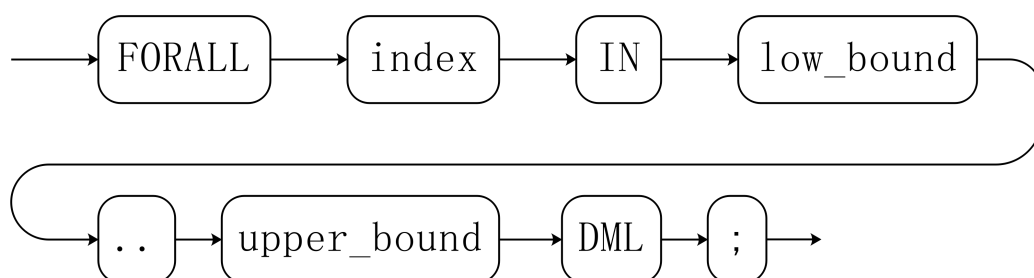
图 2-33 forall::=
