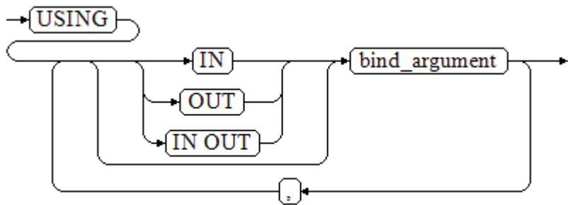
图 2-18 using_clause::=
