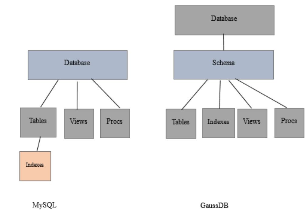
图 3-1 MySQL 和 GaussDB 中 Database 和 Schema 之间的差异
