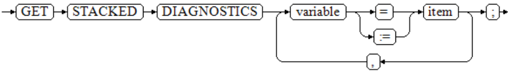
图 2-37 获取有关错误信息语法
