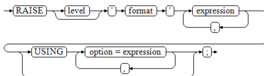
图 2-51 raise_format::=
