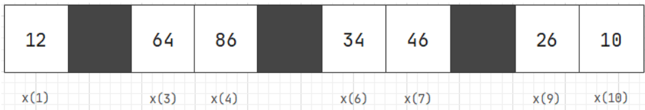
图 2-3 存储方式
