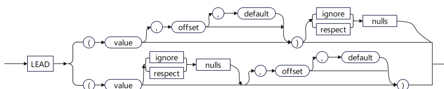
图 1-2 LEAD 语法图
