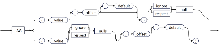
图 1-1 LAG 语法图
