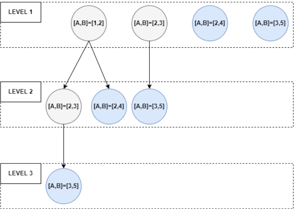
图 1-15 执行逻辑结构图
