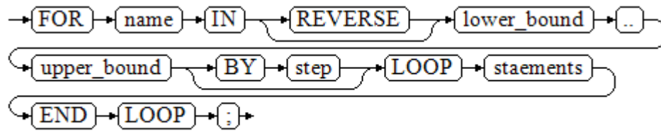
图 10-24 for_loop::=
