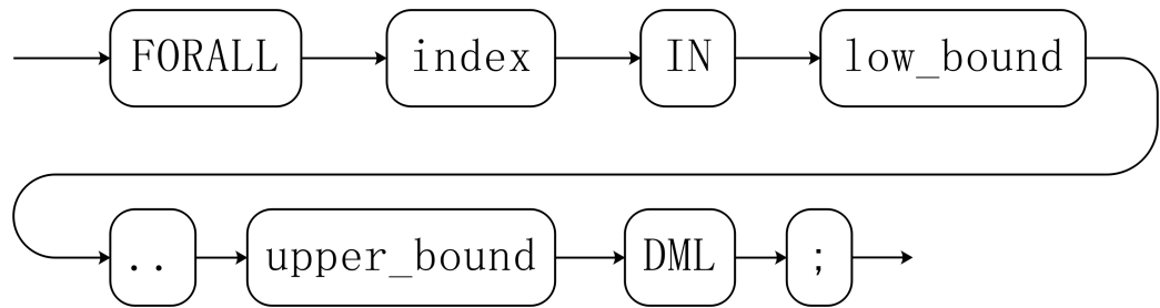
图 10-28 forall::=
