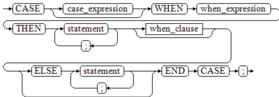
图 10-30 case_when::=
