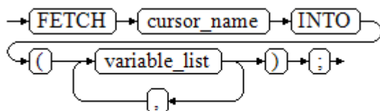
图 10-41 fetch_cursor::=
