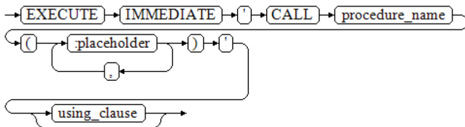
图 10-10 call_procedure::=
