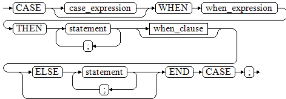
图 10-23 case_when::=
