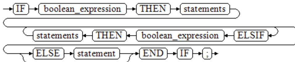
图 10-17 IF_THEN_ELSIF_ELSE::=
