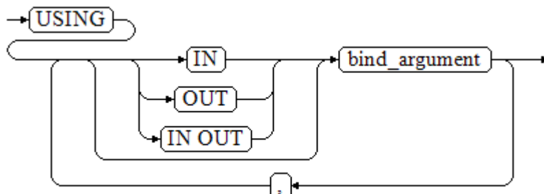
图 10-11 using_clause::=
