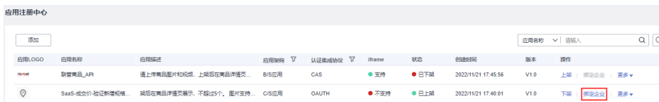
图 2-10 绑定企业
