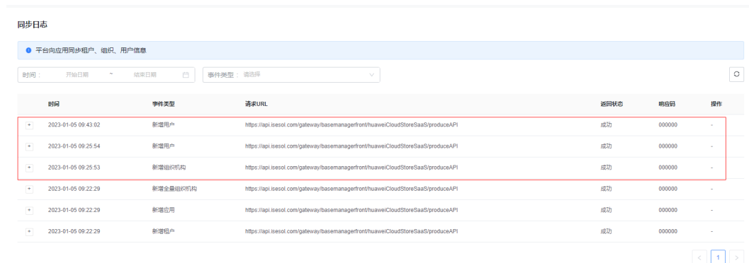
图 2-32 同步日志
