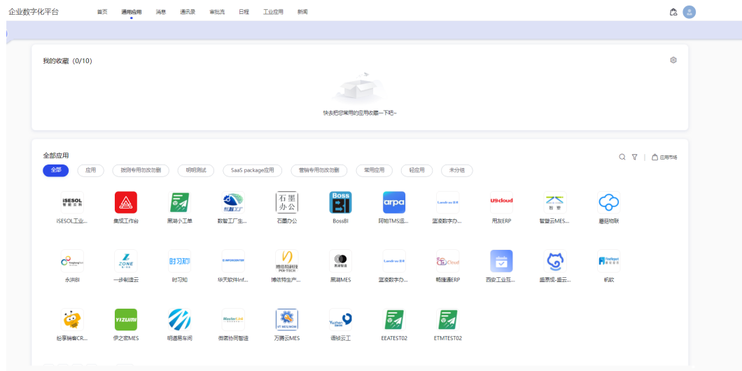
图 2-37 应用界面
