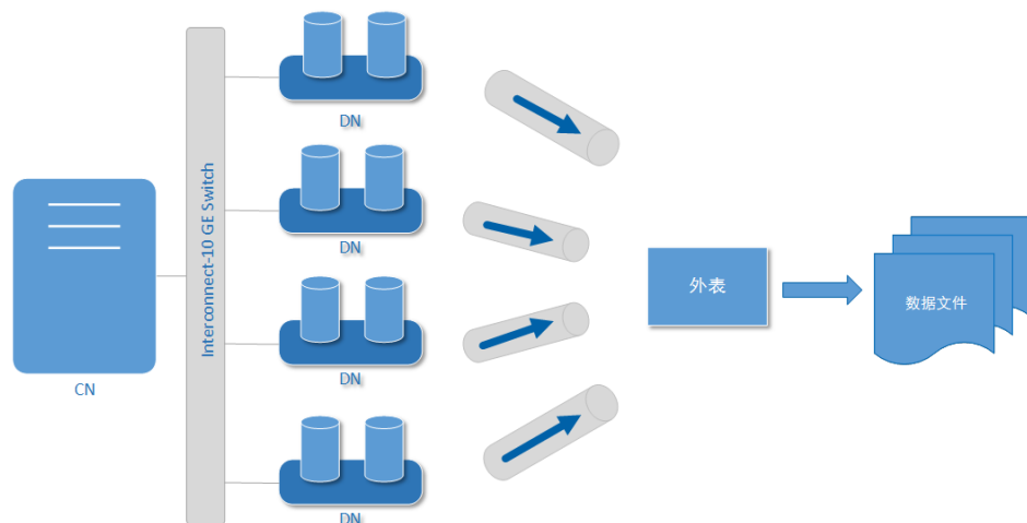
图 9-1 通过外表导出数据
