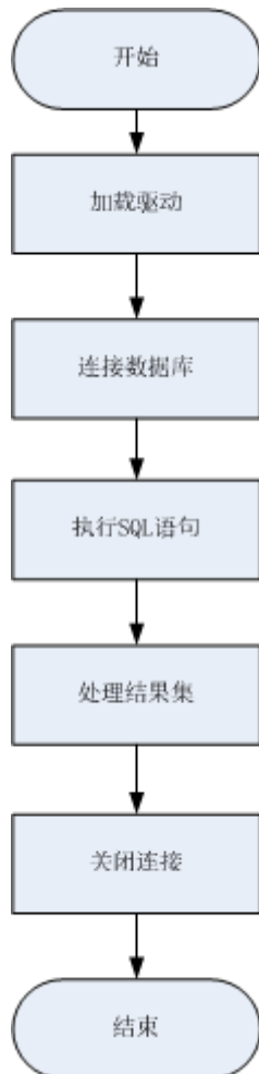
图 6-4 采用 Psycopg2 开发应用程序的流程
