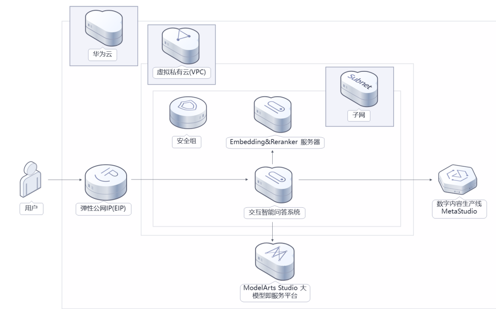
图 1-1 方案架构图
