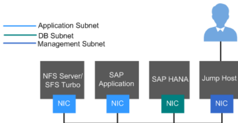
图 2-2 网络平面规划
