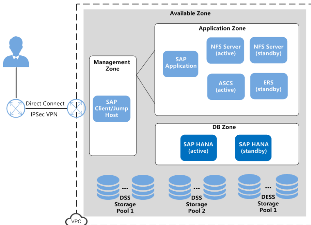
图 3-1 单节点部署
