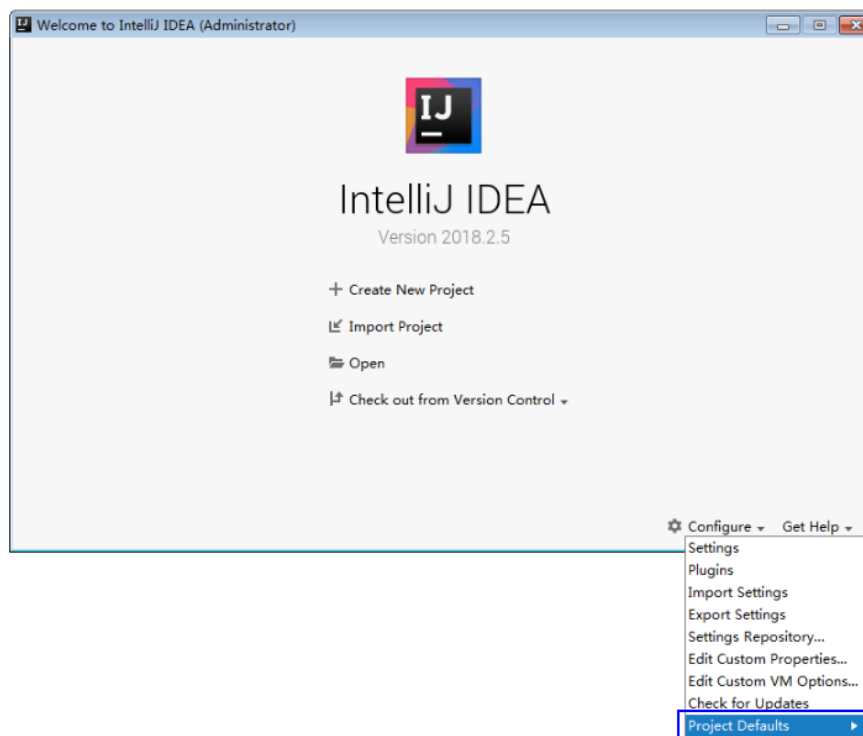
图 27-11 Configure
