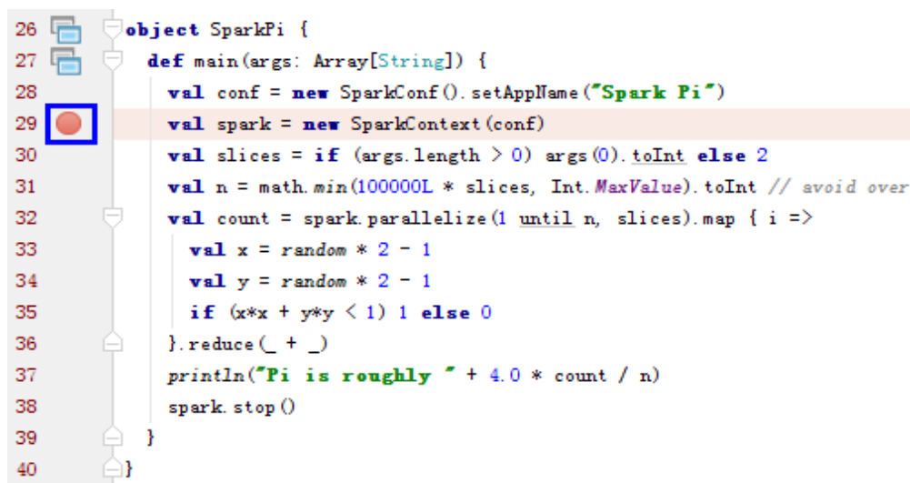
图 28-49 设置断点
