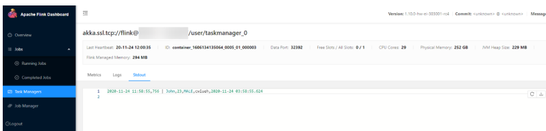
图 9-59 运行结果
