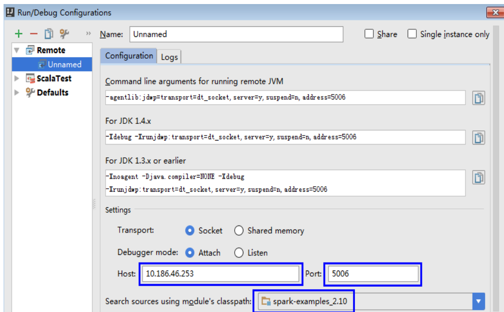
图 28-46 选择 Remote
