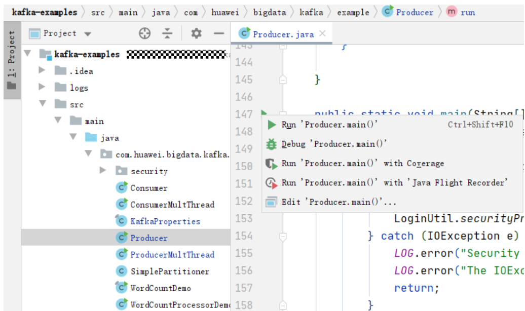
图 19-11 运行 Producer.java
