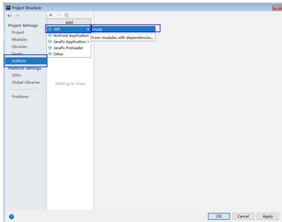
图 30-14 添加 Artifacts
