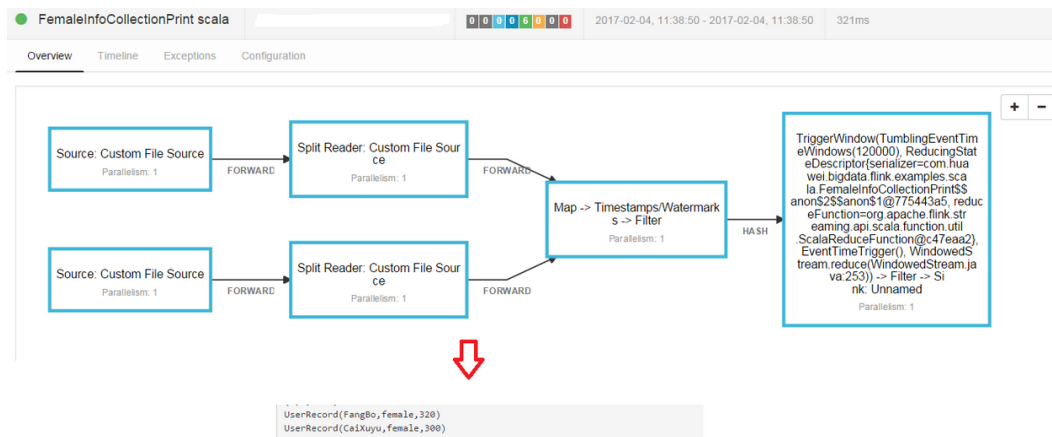
图 10-34 显示图
