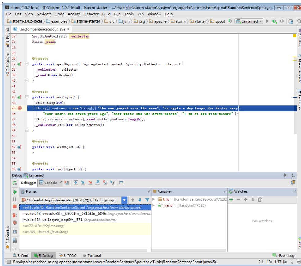
图 30-25 调试
