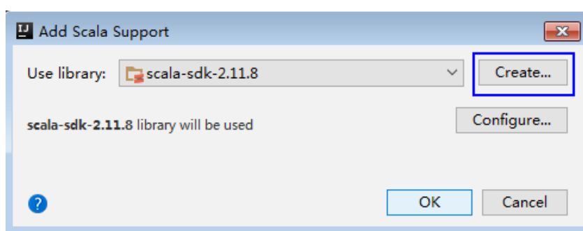
图 28-27 Create...
