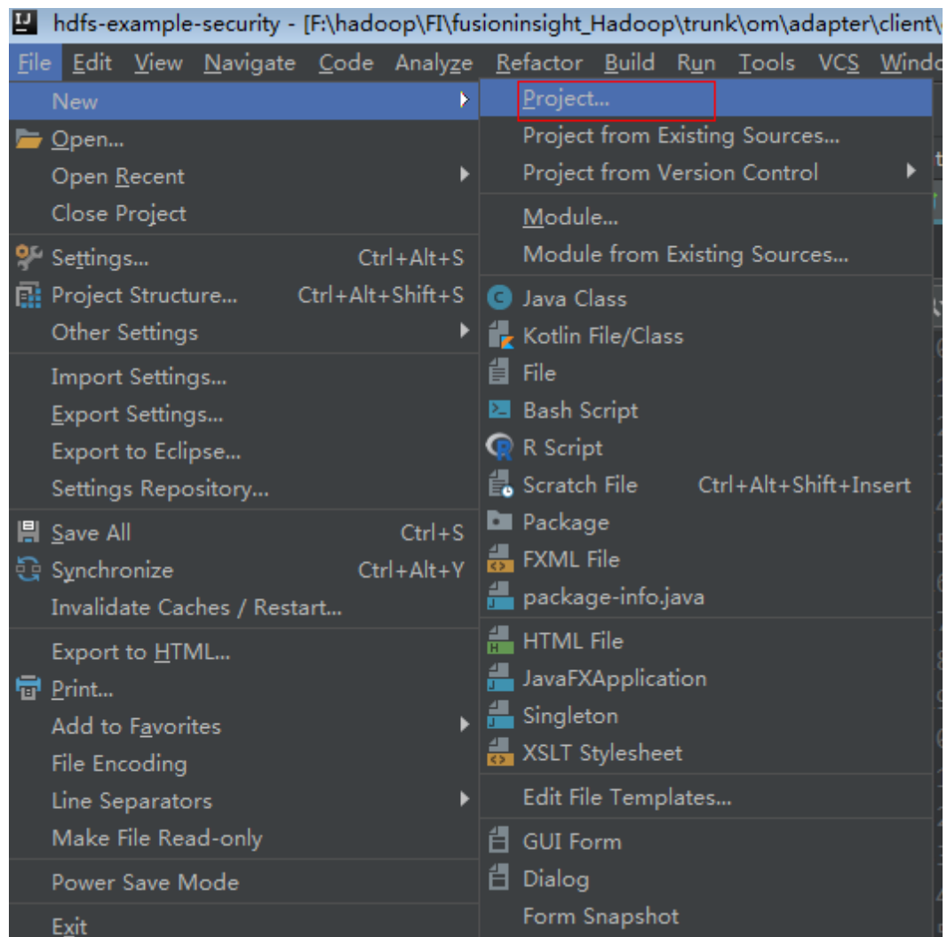
图 23-5 创建工程
