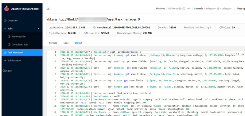
图 9-53 输出结果
