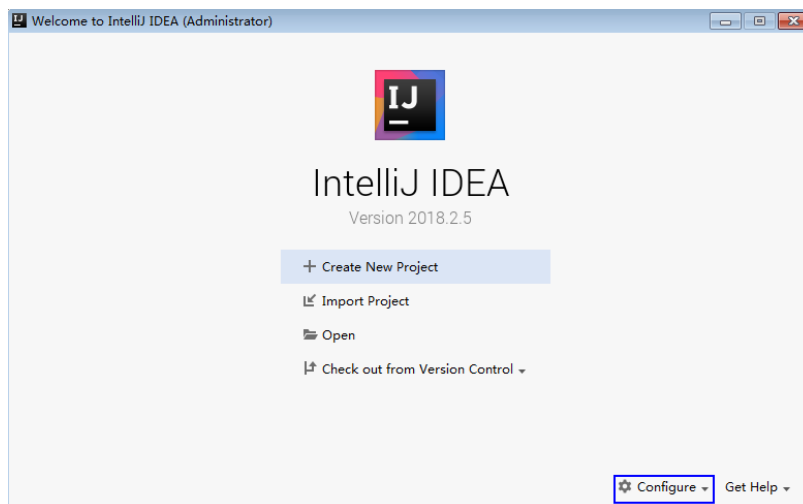
图 28-10 Quick Start
