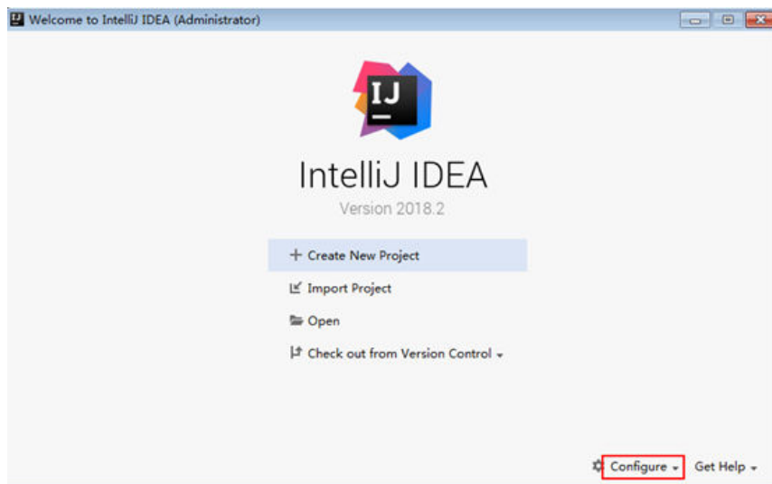
图 20-2 Quick Start
