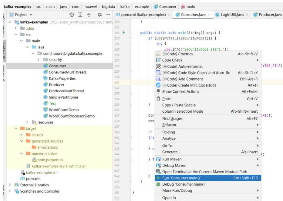
图 19-19 运行 Consumer.java
