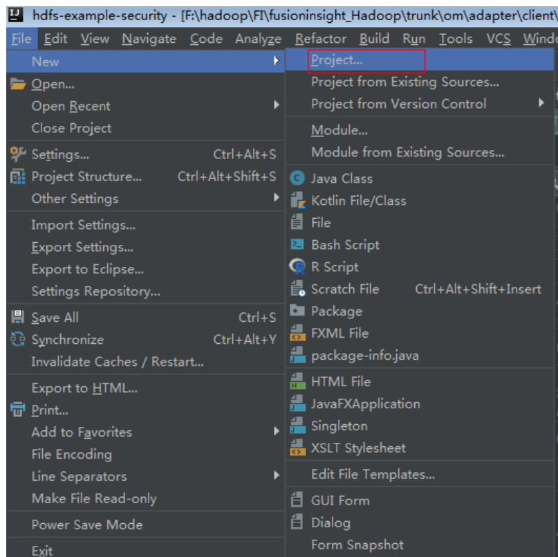
图 24-5 创建工程
