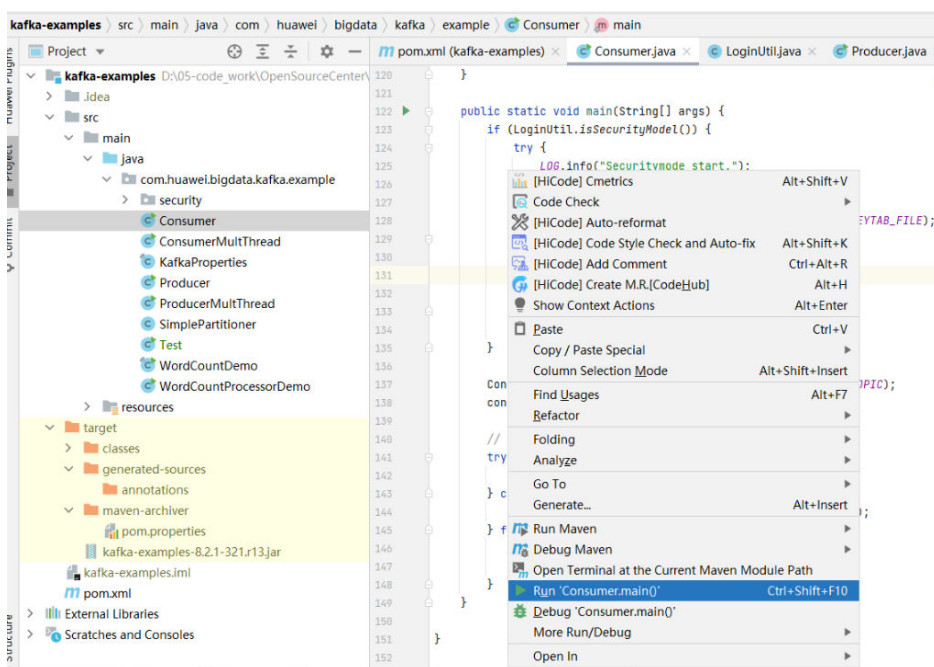
图 20-15 运行 Consumer.java
