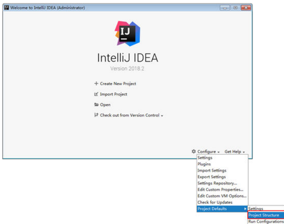
图 14-4 Configure
