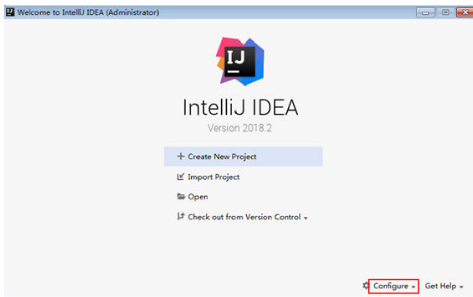
图 14-3 Quick Start
