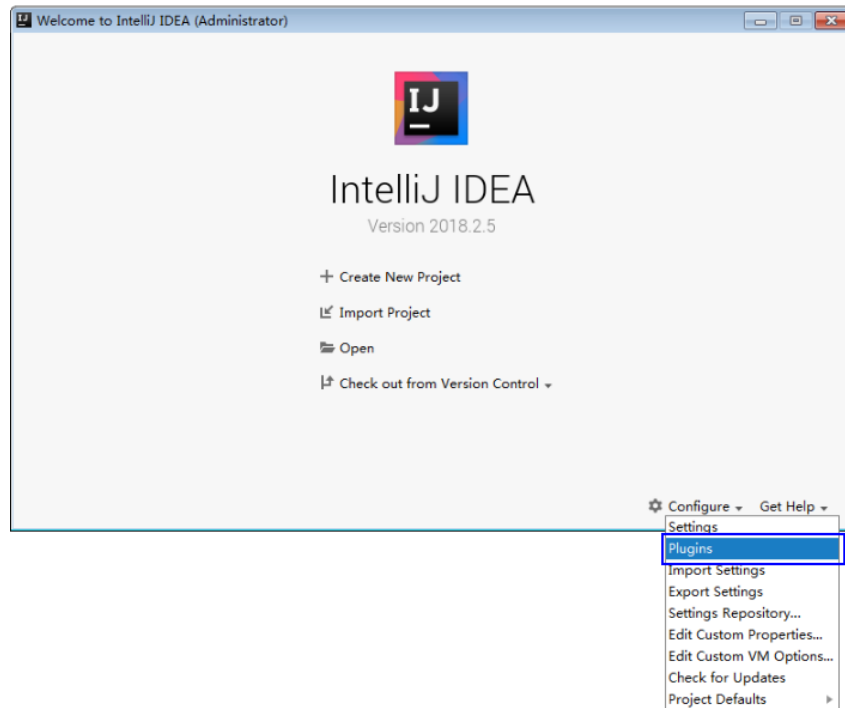
图 27-16 Plugins
