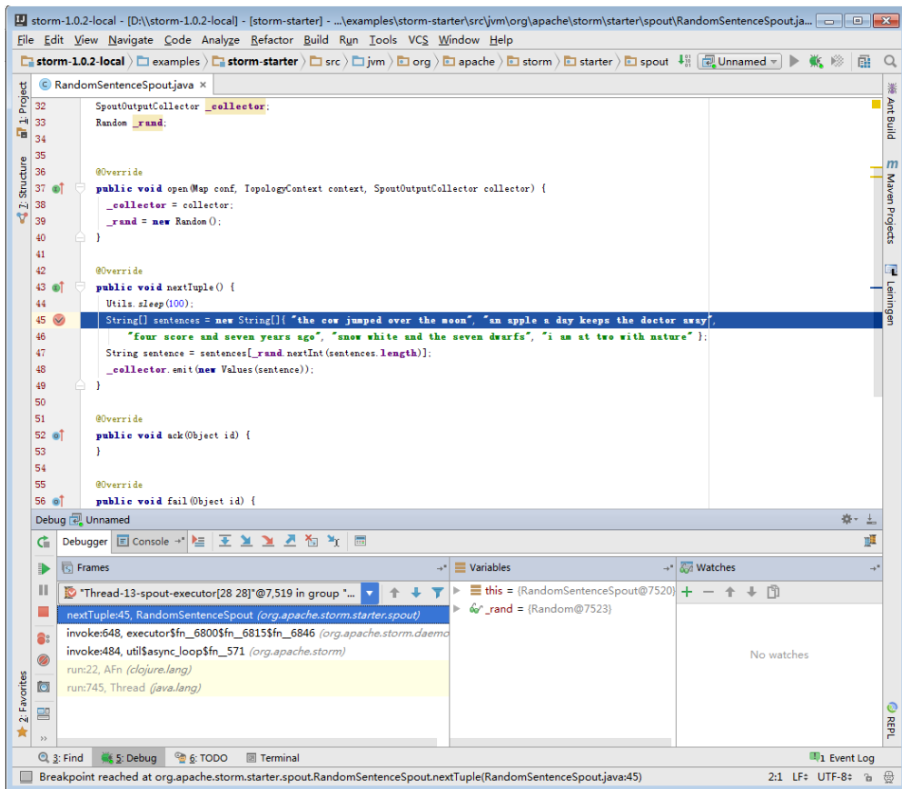
图 29-25 调试
