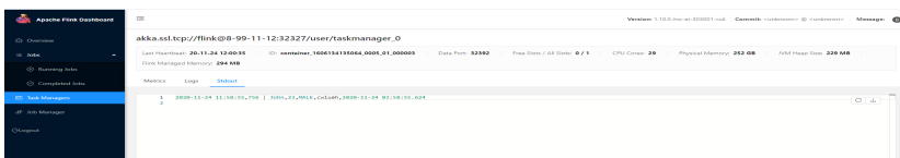
图 10-51 运行结果
