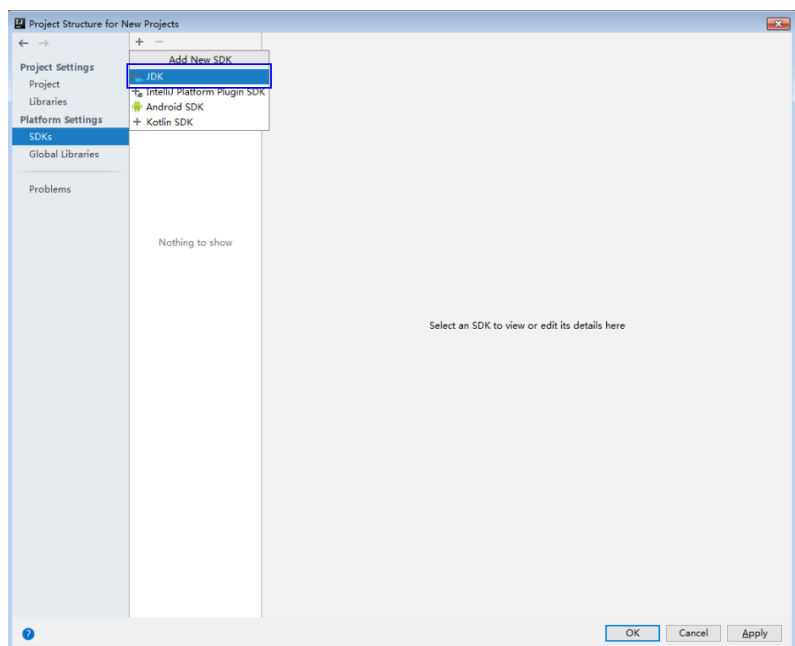
图 28-13 添加 JDK
