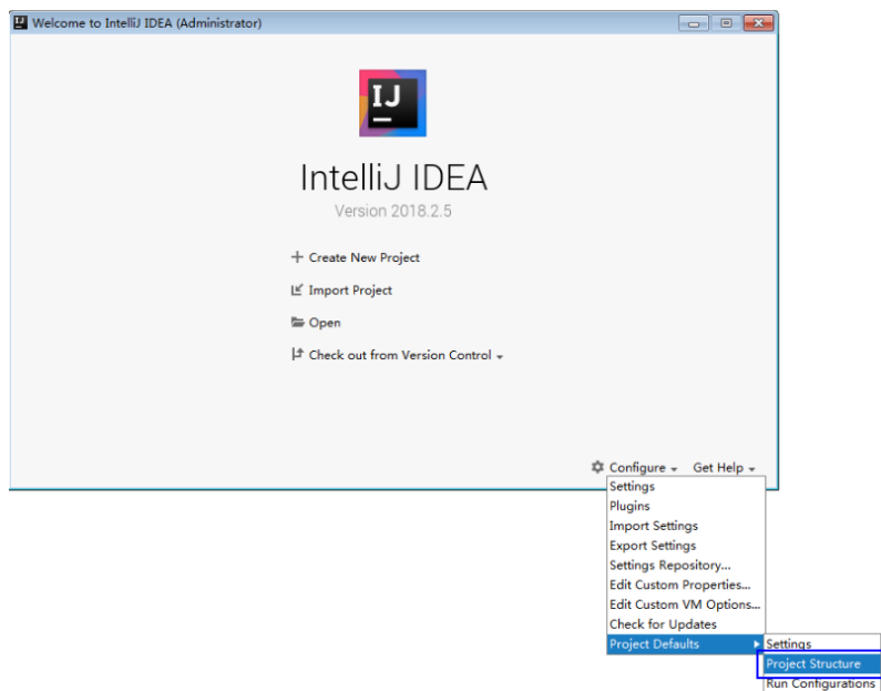
图 28-12 Project Defaults
