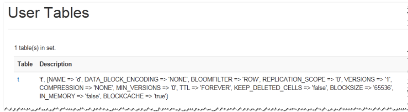
图 11-30 TableDetails
