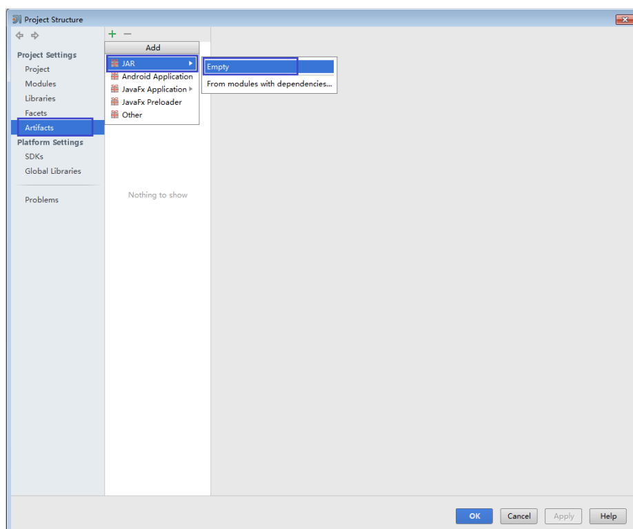
图 9-40 添加 Artifacts
