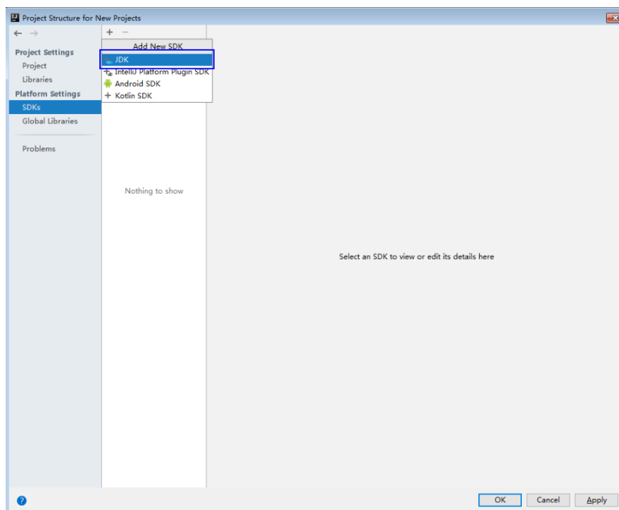
图 27-13 添加 JDK
