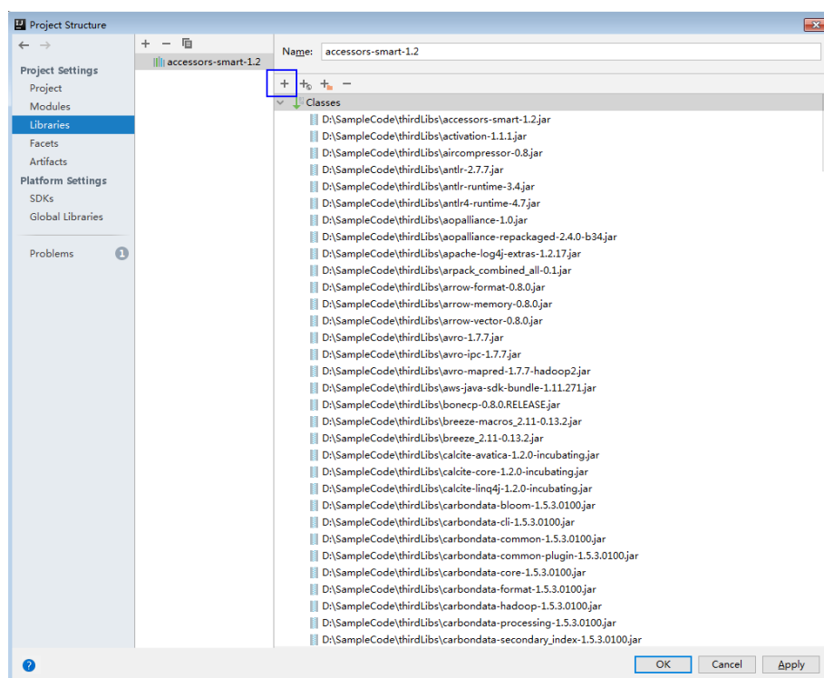
图 28-41 添加依赖包
