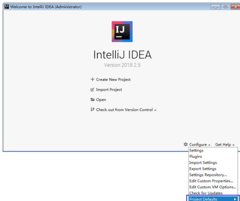
图 28-11 Configure
