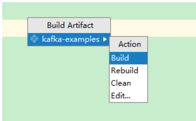
图 19-17 Build
