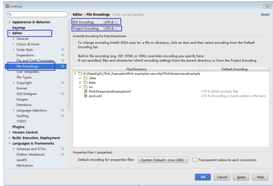
图 9-29 Settings
