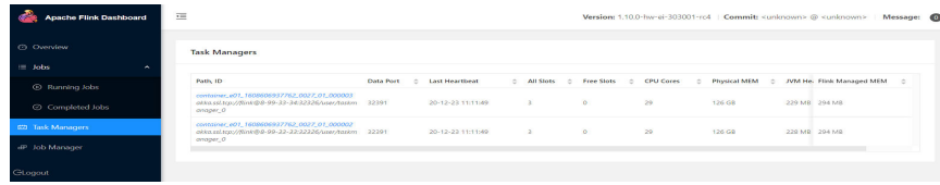
图 10-43 提交的任务
