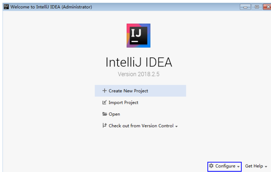
图 27-10 Quick Start
