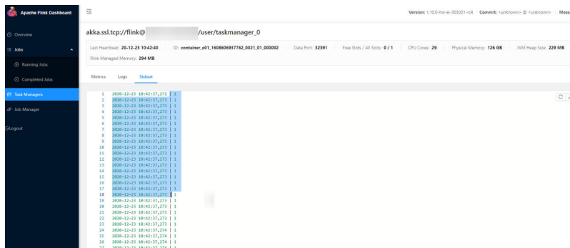
图 9-46 运行结果
