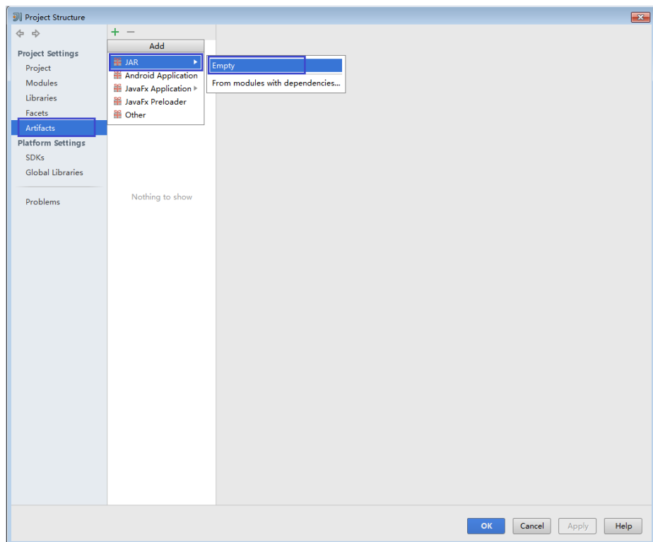
图 10-35 添加 Artifacts
