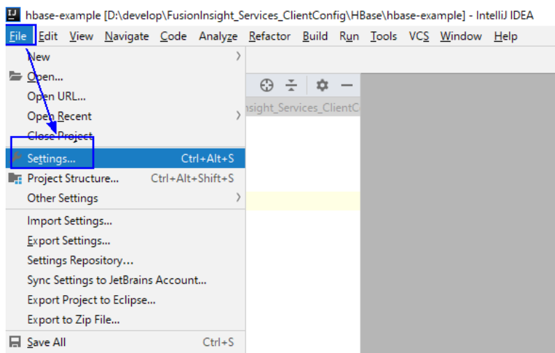
图 12-14 Settings
