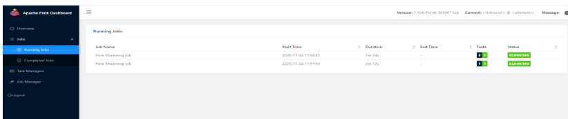
图 10-49 运行的作业
