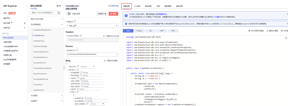
图 1-2 获取 SDK 代码示例
