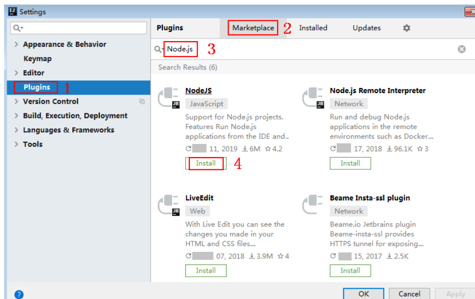
图 2-27 安装 NodeJS 插件
