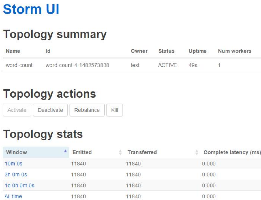
图 15-3 Storm 应用程序执行界面
