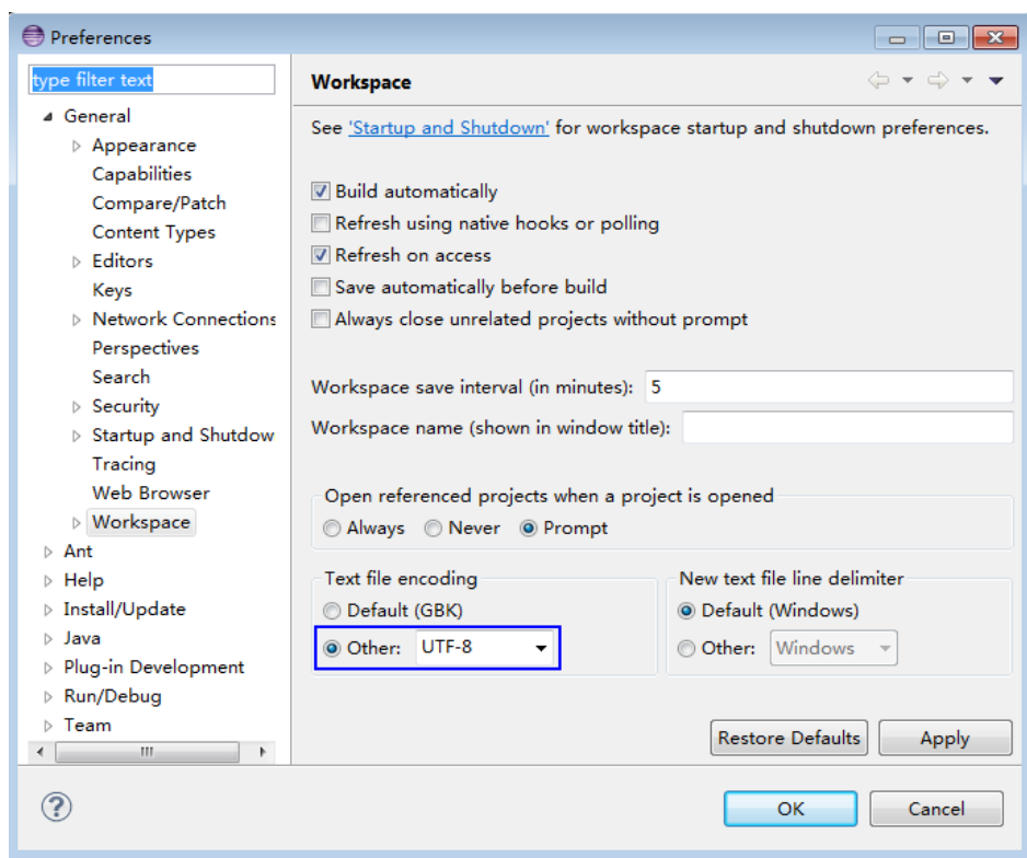
图 10-2 设置 Eclipse 的编码格式
