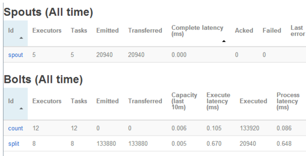
图 15-4 Storm 应用程序算子发送数据总量
