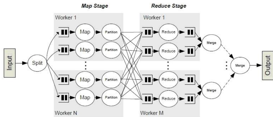
图 14-4 算法流程
