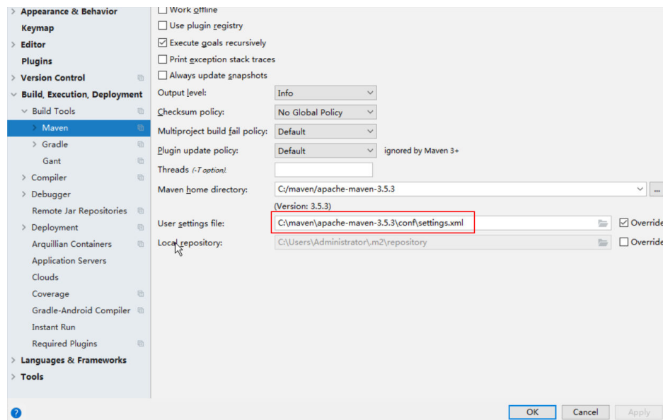
图 25-4 “settings.xml”文件放置目录
