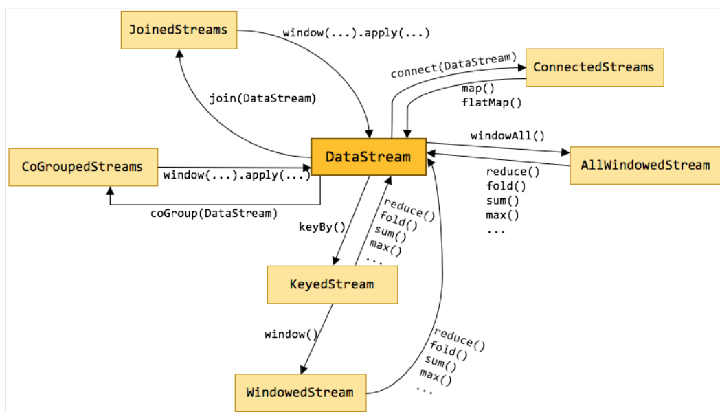
图 11-56 Flink Stream 的各种流类型转换
