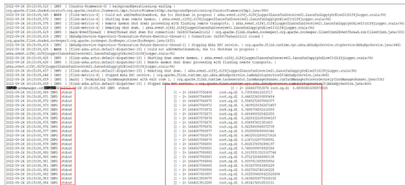
图 20-27 读取 IoTDB 数据成功
