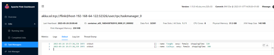
图 5-19 查看程序运行结果
