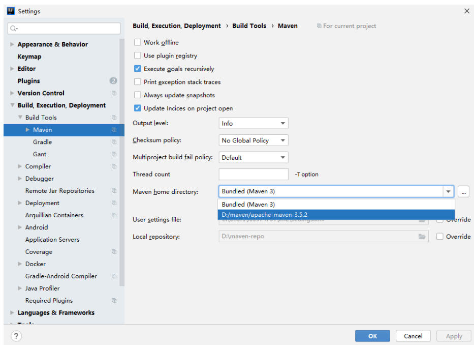
图 23-12 选择本地 Maven 安装目录
