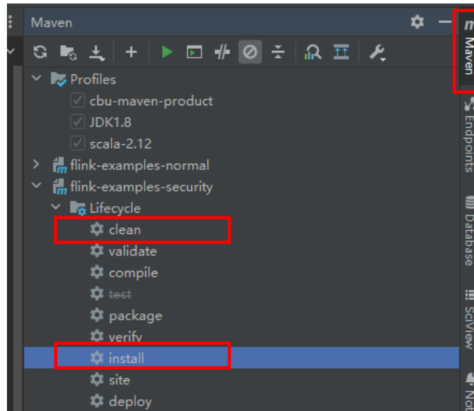
图 12-42 maven 工具 clean 和 install
