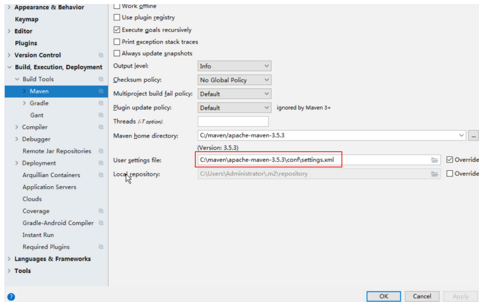
图 26-4 “settings.xml”文件放置目录
