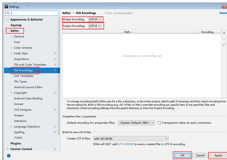
图 18-9 设置 IntelliJ IDEA 的编码格式
