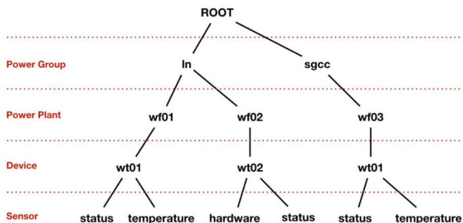
图 21-1 电力场景属性层级组织结构
