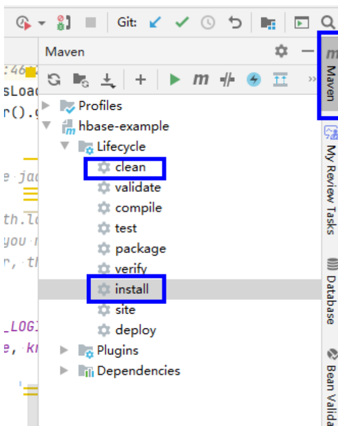
图 11-11 maven 工具 clean 和 install
