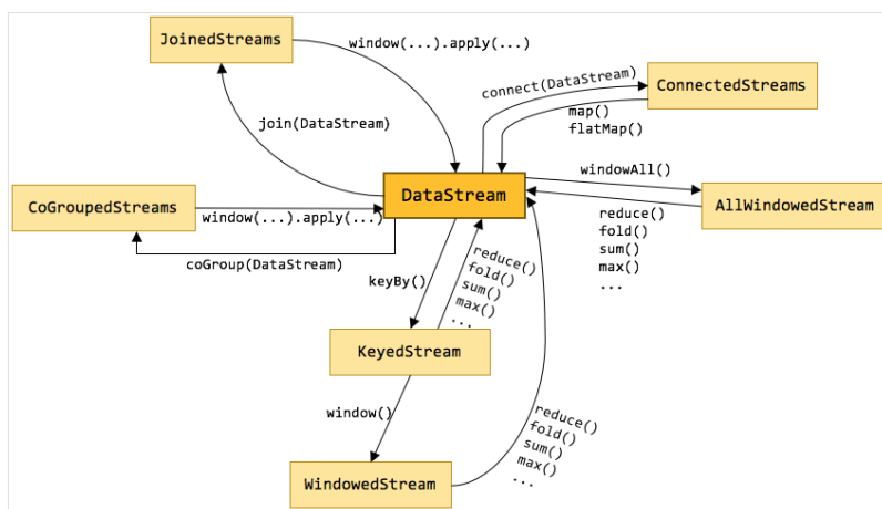
图 12-63 Flink Stream 的各种流类型转换
