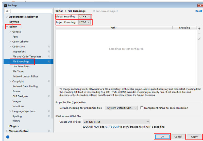
图 9-2 设置 IntelliJ IDEA 的编码格式
