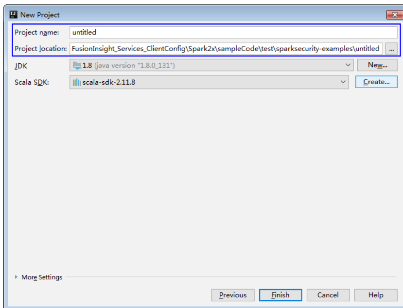
图 31-34 填写工程信息
