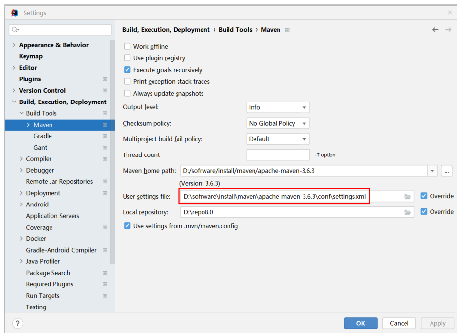
图 12-35 “settings.xml” 文件放置目录
