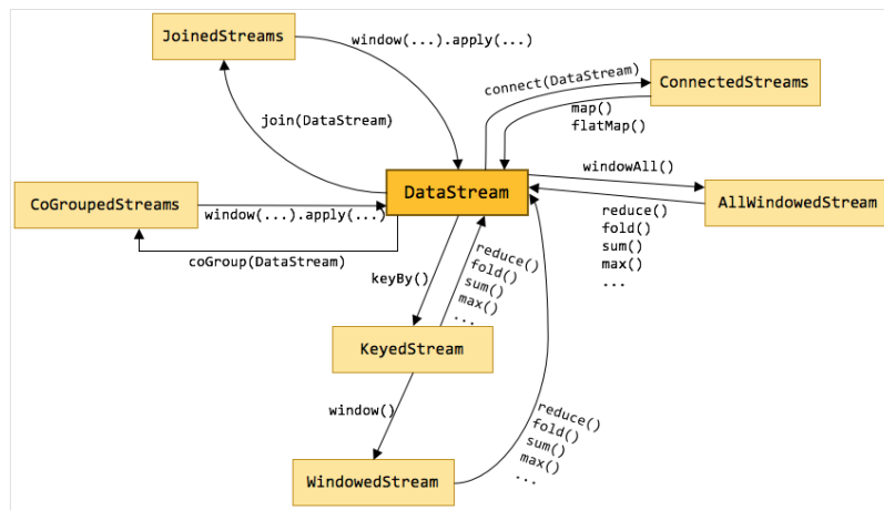
图 10-60 Flink Stream 的各种流类型转换
