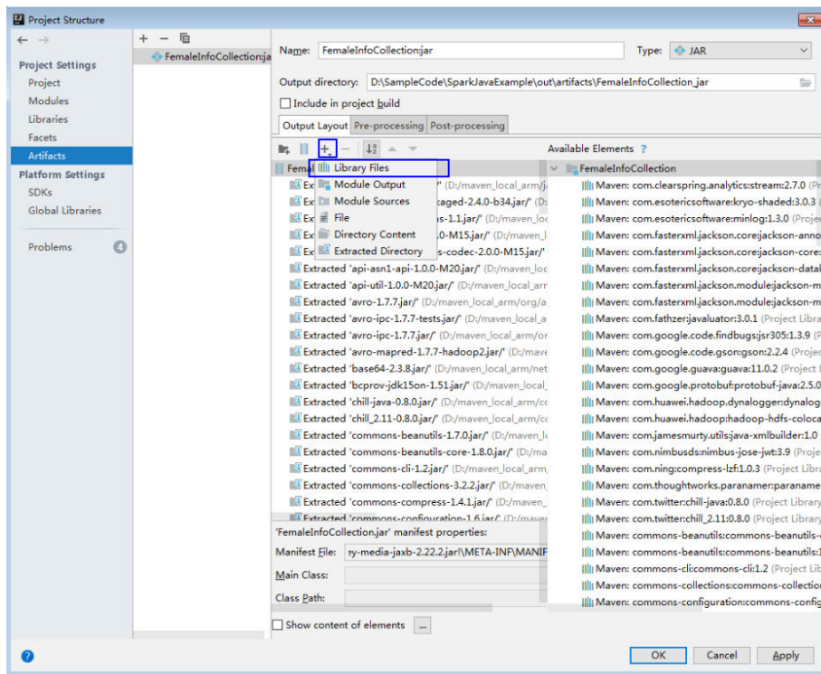
图 31-42 添加 Library Files
