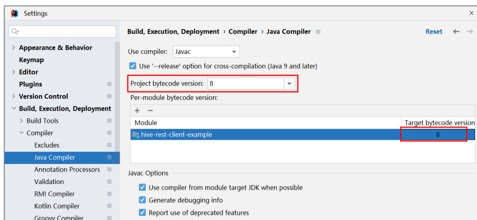
图 18-12 设置“Target bytecode version”
