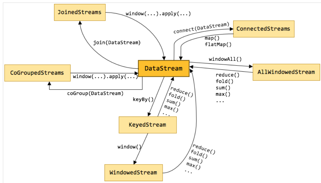
图 10-61 Flink Stream 的各种流类型转换
