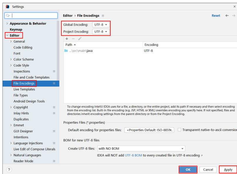
图 10-31 设置 IntelliJ IDEA 的编码格式
