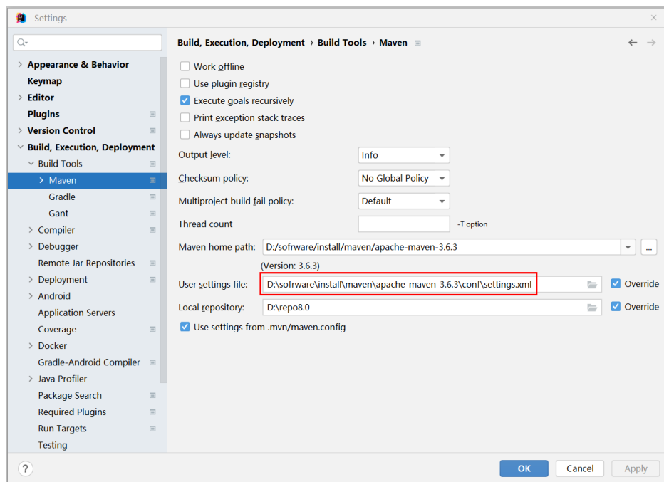
图 18-17 “settings.xml” 文件放置目录
