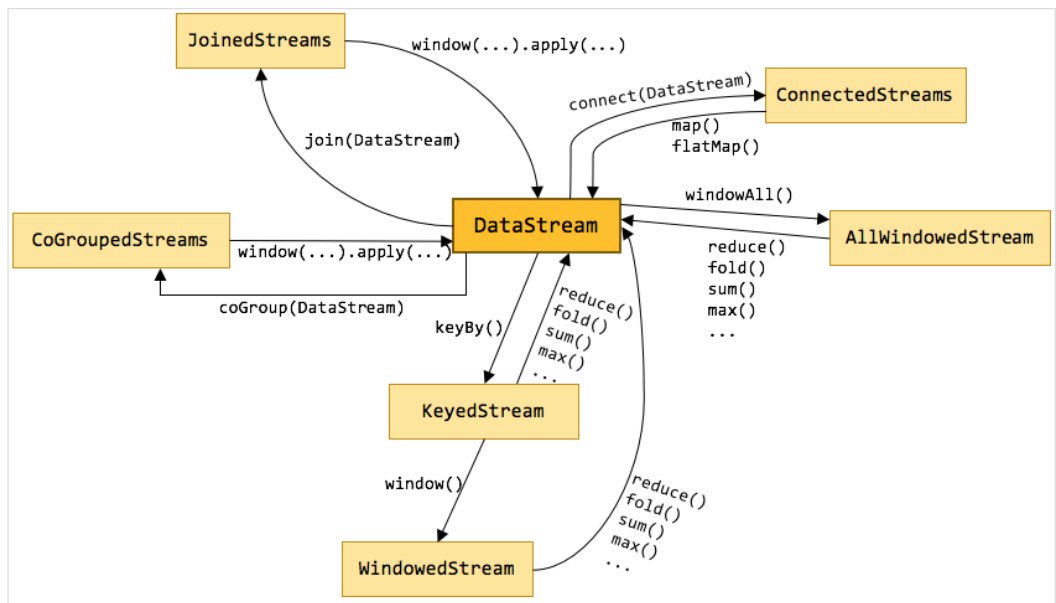
图 13-60 Flink Stream 的各种流类型转换
