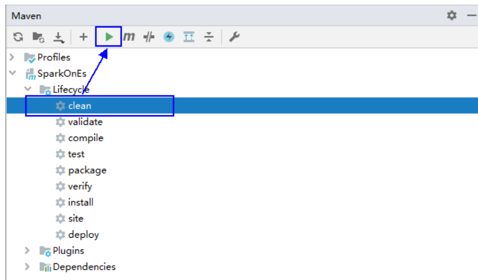
图 30-37 选择 clean 生命周期，执行 Maven 构建过程
