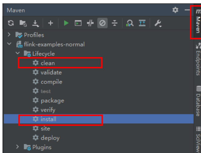
图 13-41 maven 工具 clean 和 install
