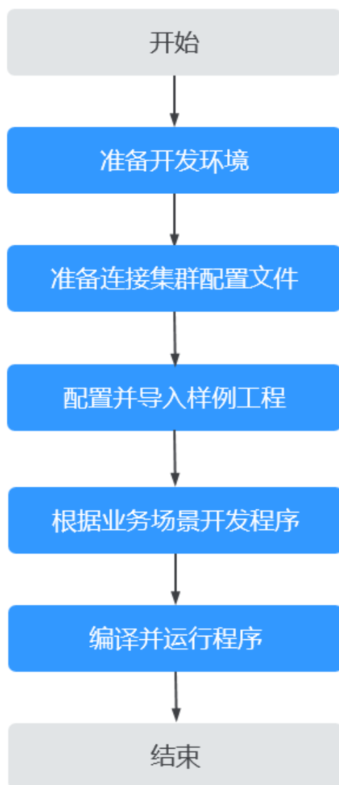
图 22-2 IoTDB 应用程序开发流程
