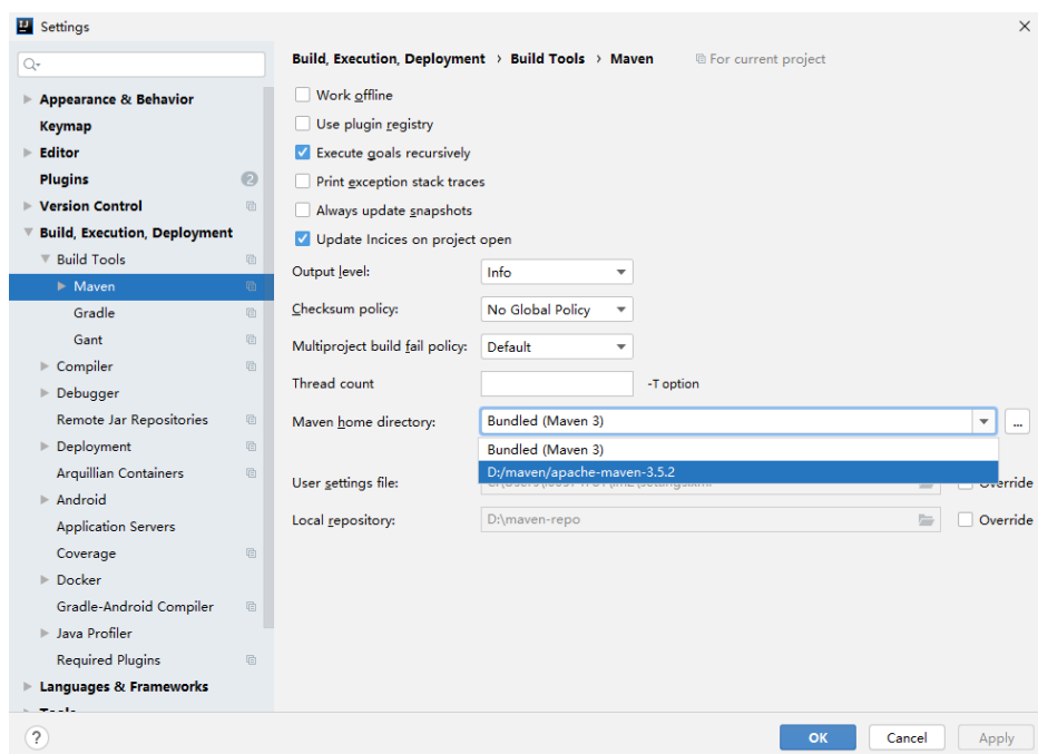
图 22-12 选择本地 Maven 安装目录
