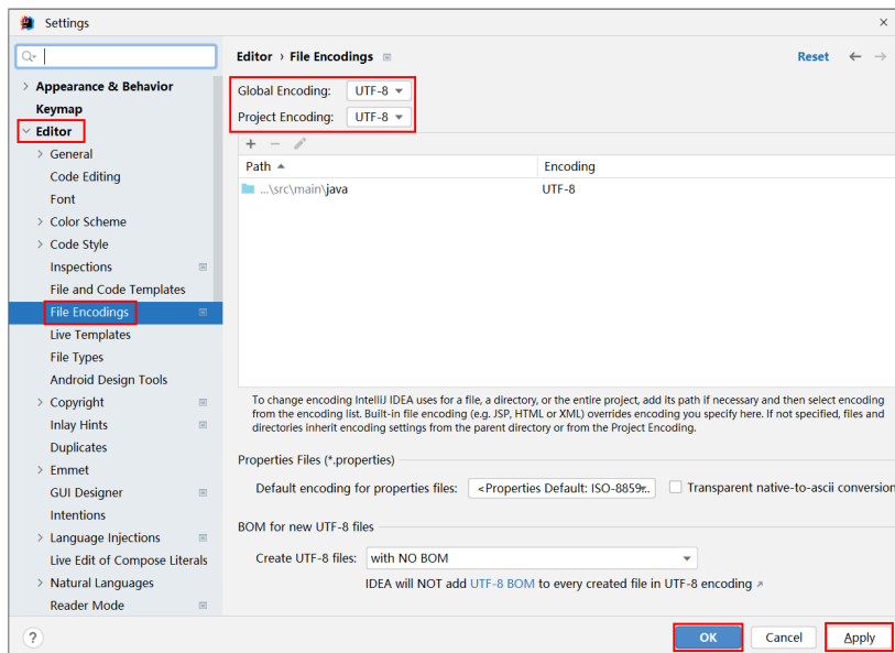
图 18-11 设置 IntelliJ IDEA 的编码格式
