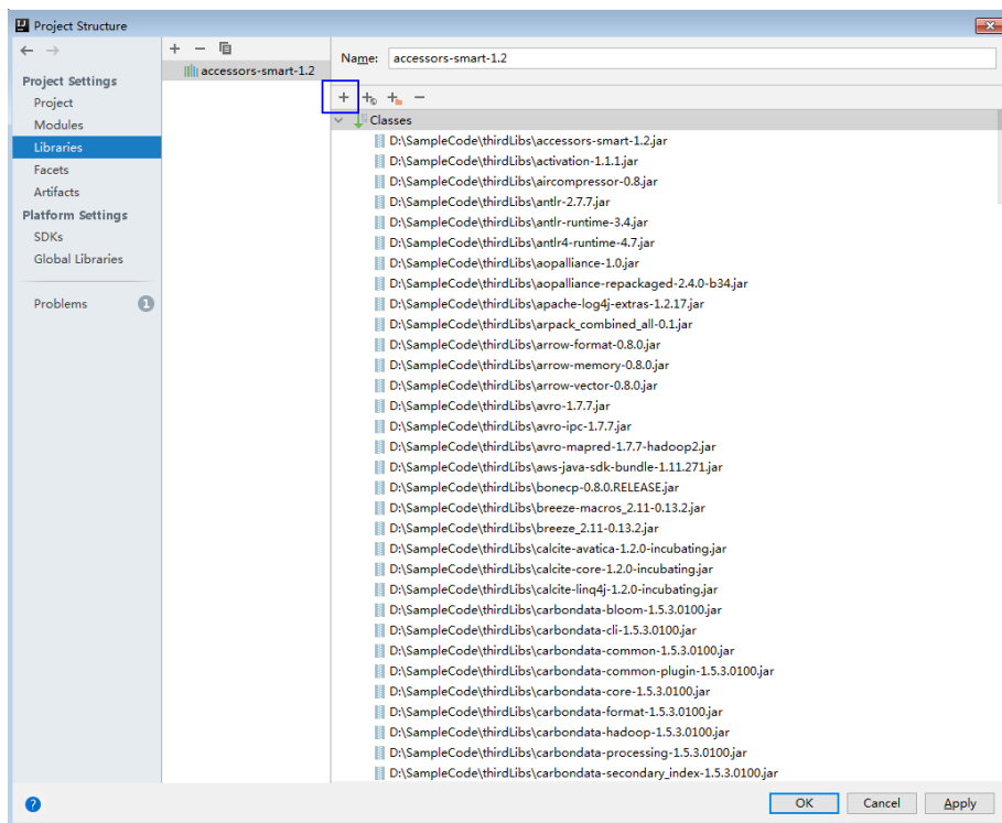
图 31-41 添加依赖包
