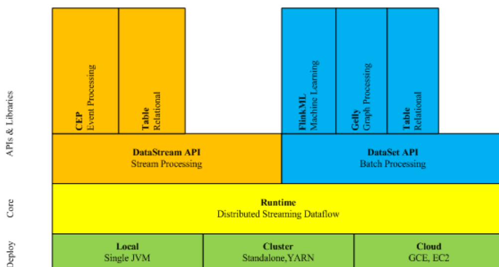
图 13-1 Flink 技术栈
