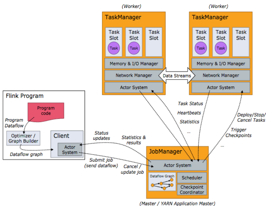
图 12-2 Flink 架构
