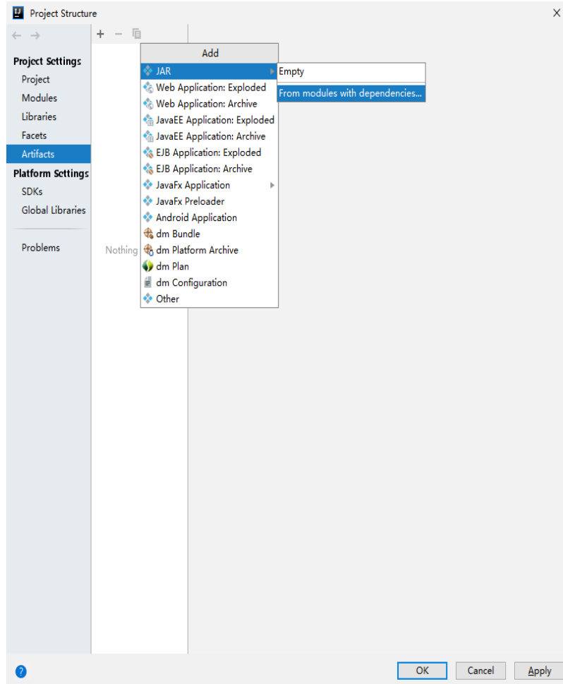
图 22-20 添加 Artifacts
