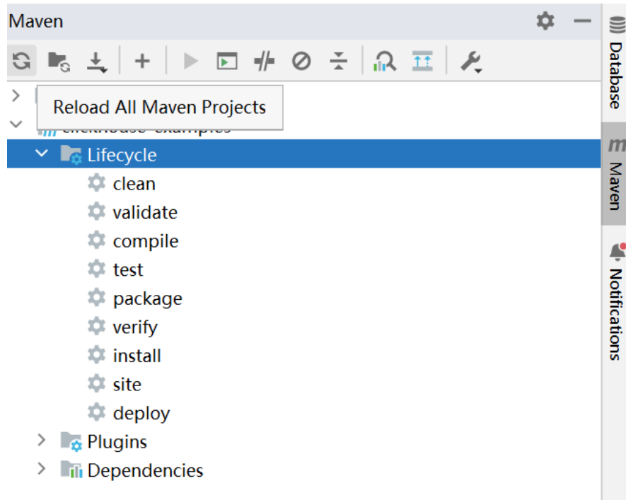
图 8-2 reload projects
