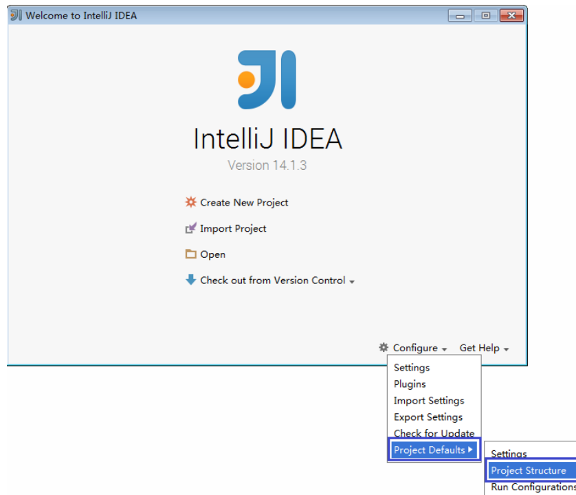
图 13-7 Project Defaults
