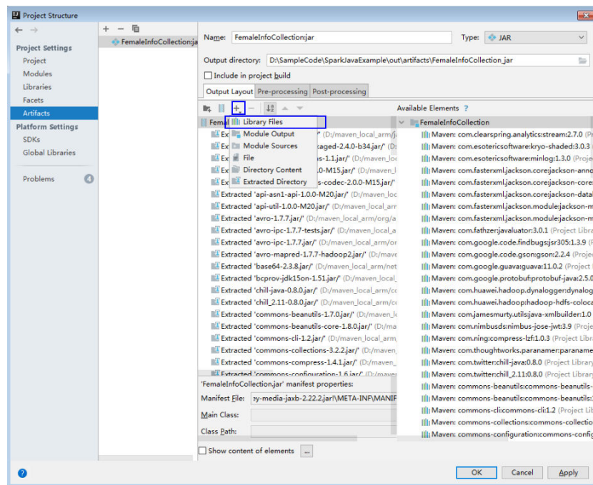
图 30-42 添加 Library Files
