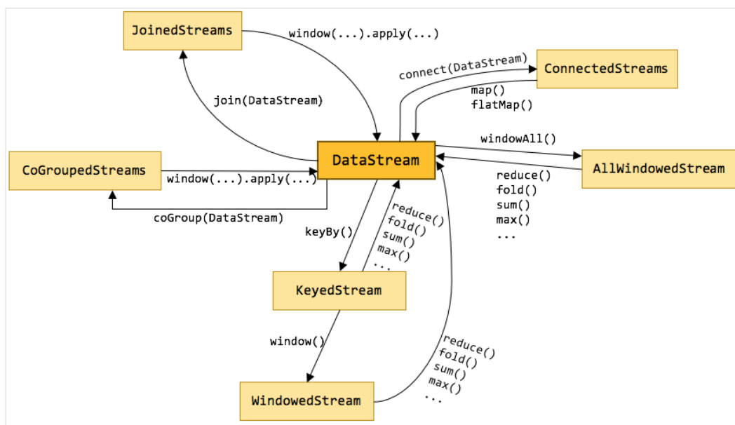
图 11-57 Flink Stream 的各种流类型转换
