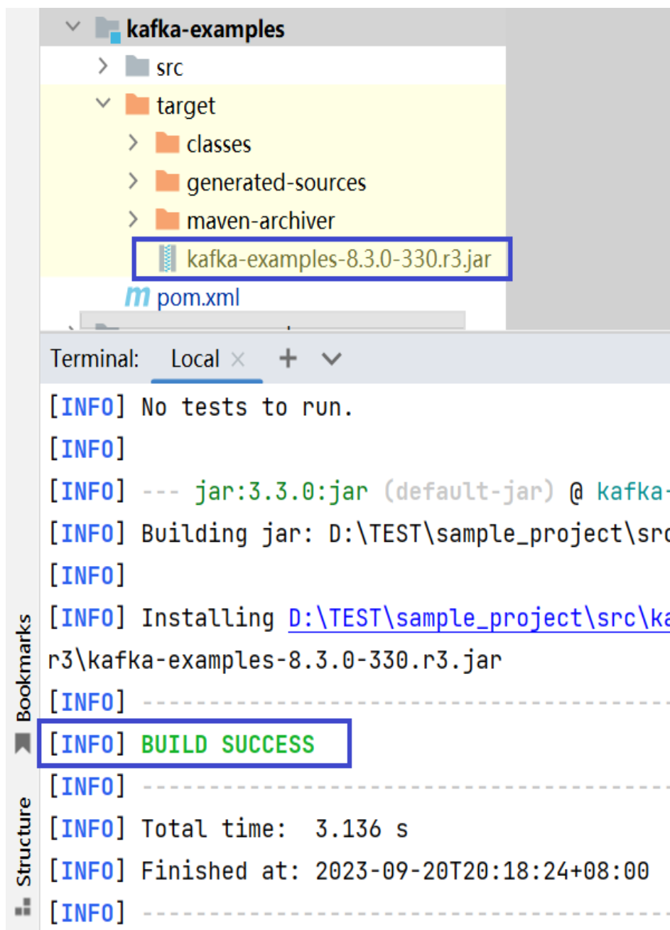
图 25-14 编译完成，生成 jar 包
