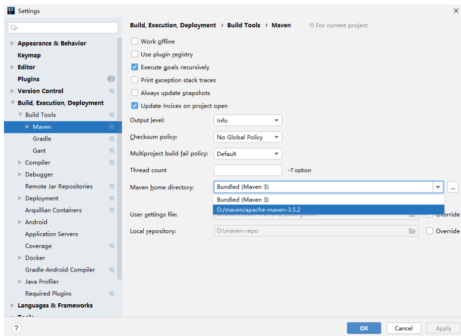
图 24-8 选择本地 Maven 安装目录
