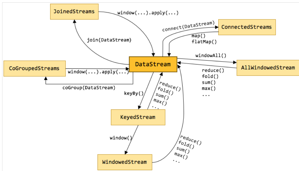
图 13-59 Flink Stream 的各种流类型转换
