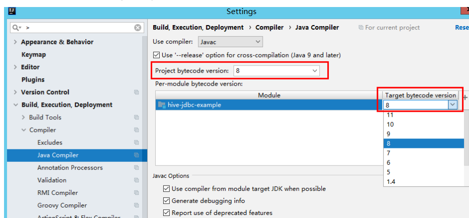
图 19-3 修改 “Target bytecode version”
