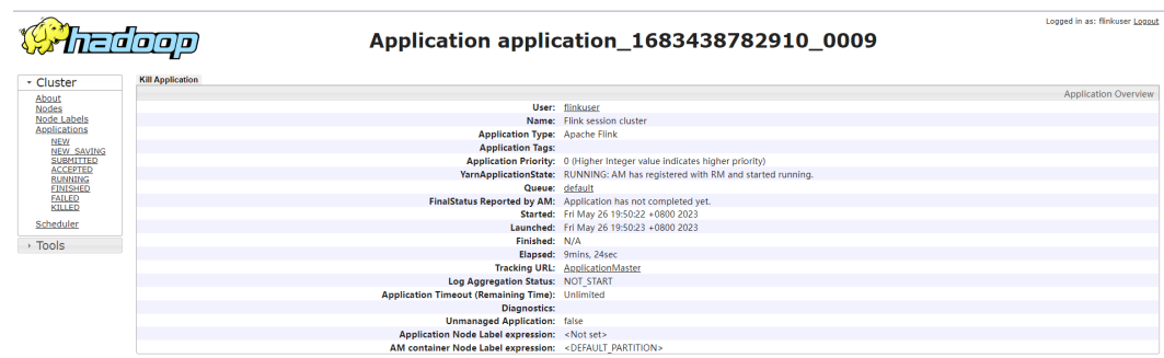
图 5-17 查看 Yarn 作业详情
