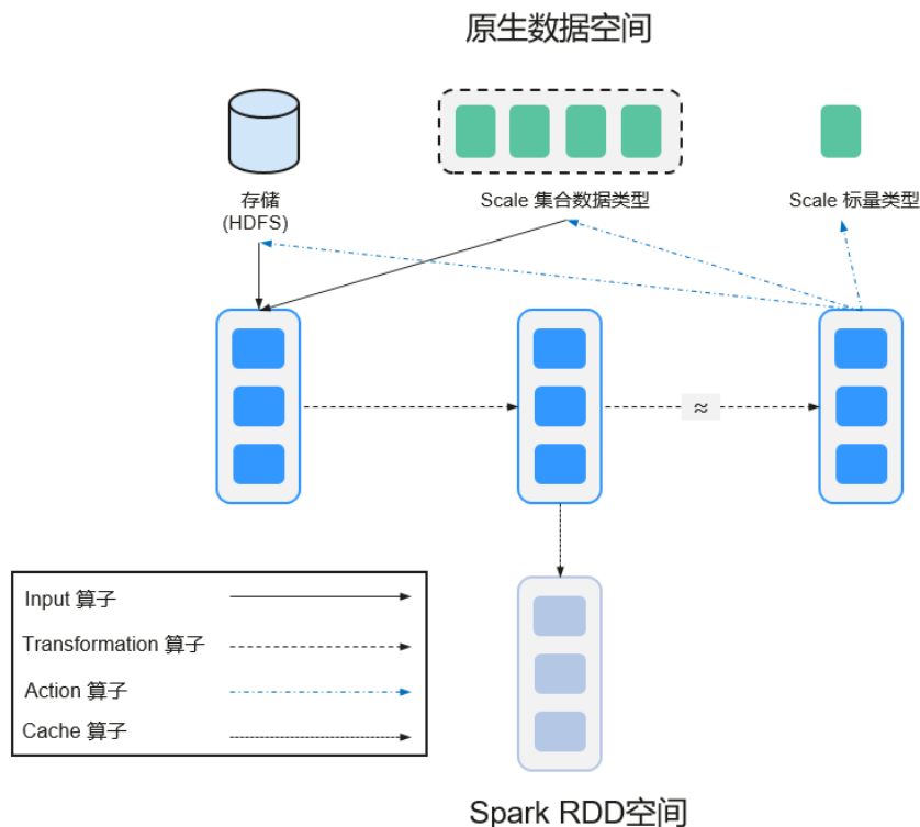
图 30-2 RDD 操作示例
