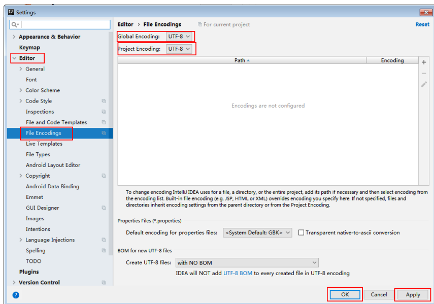
图 25-9 设置 IntelliJ IDEA 的编码格式
