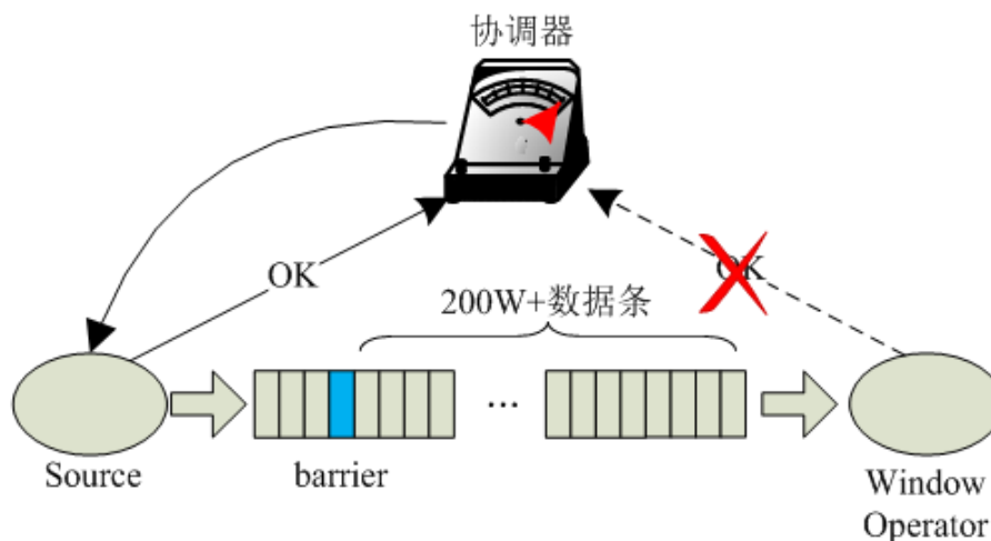
图 13-65 关系图
