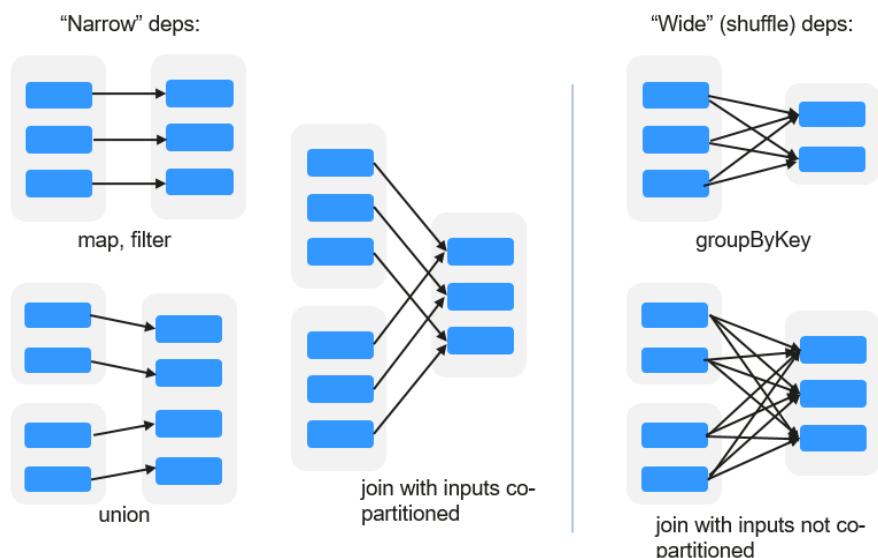
图 30-1 RDD 的依赖
