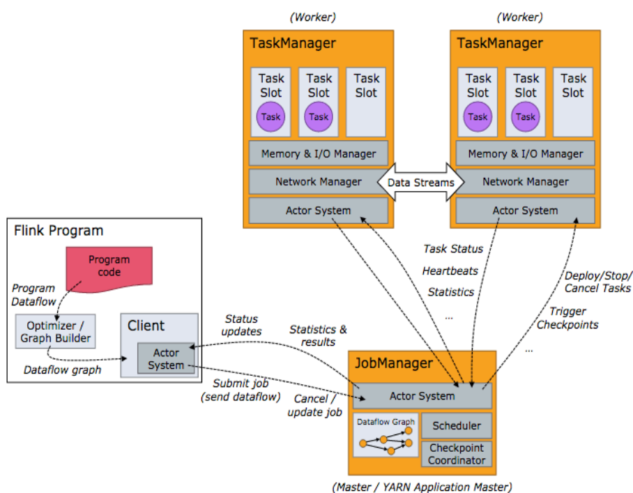
图 13-2 Flink 架构
