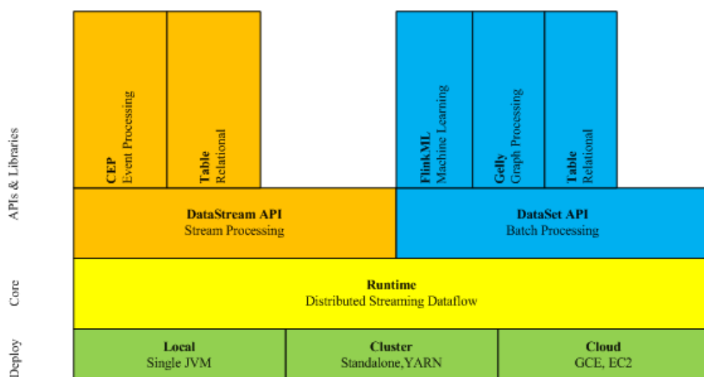
图 12-1 Flink 技术栈
