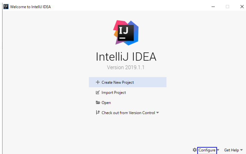
图 22-4 Quick Start
