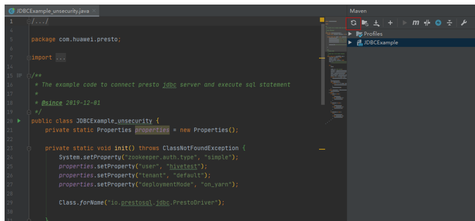
图 19-2 导入依赖
