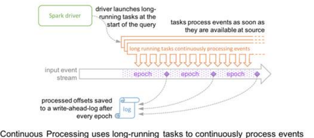
图 31-7 连续模式运行过程简图
