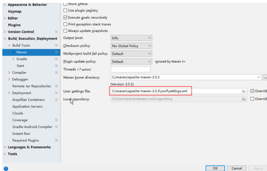
图 20-3 “settings.xml” 文件放置目录
