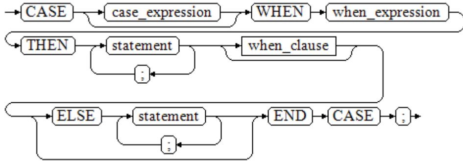
图 9-24 case_when::=
