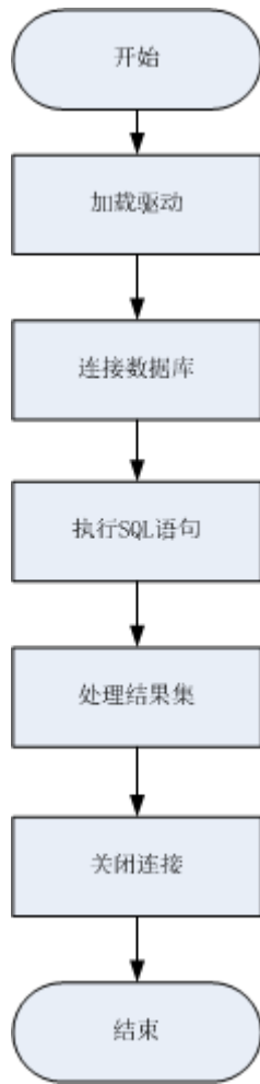
图 11-1 采用 JDBC 开发应用程序的流程
