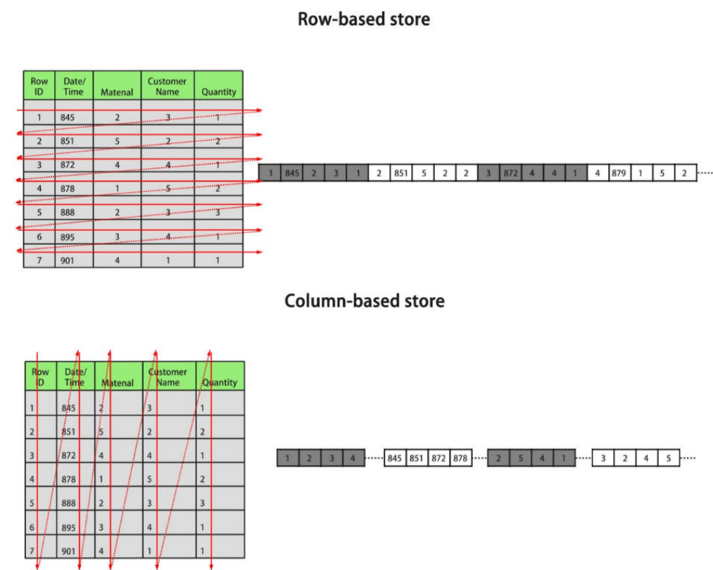
图 3-1 行存储和列存储的差异
