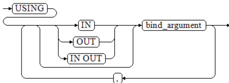
图 9-12 using_clause-3
