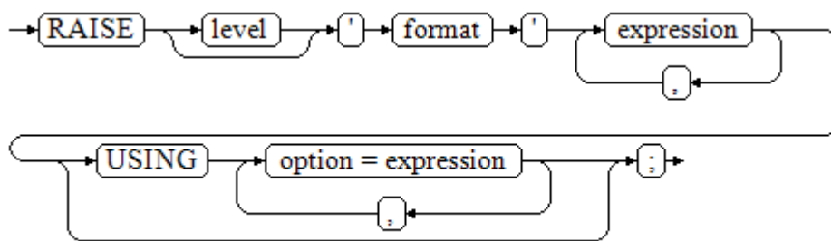
图 9-34 raise_format::=
