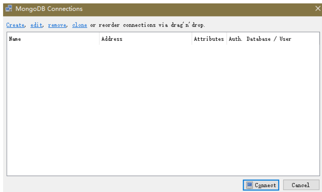
图 10-4 工具主界面
