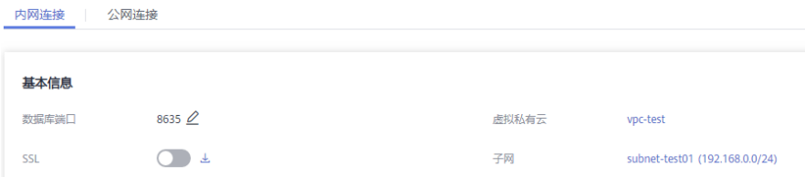
图 9-3 SSL 关闭
