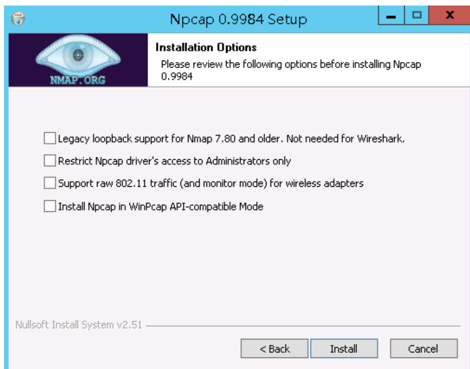
图 4-8 安装 “Npcap”
