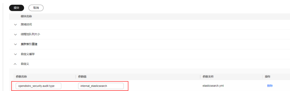
图 3-5 自定义参数
