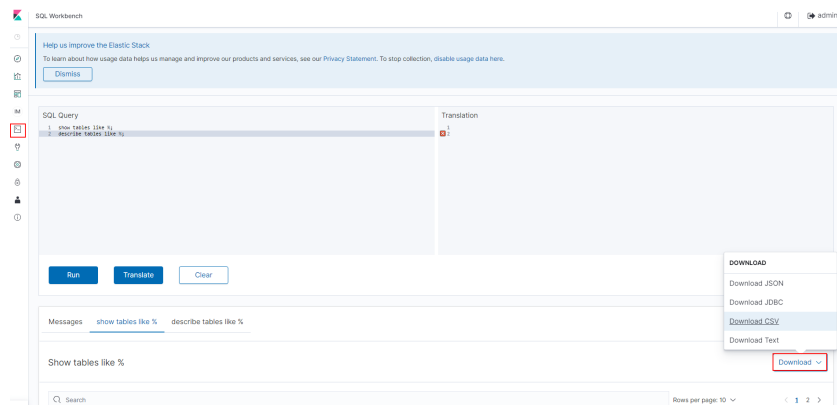
图 10-2 SQL Workbench
