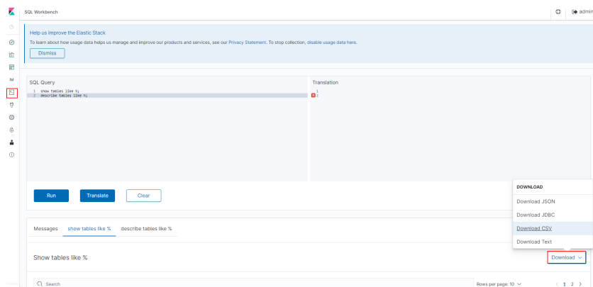
图 1-1 SQL Workbench
