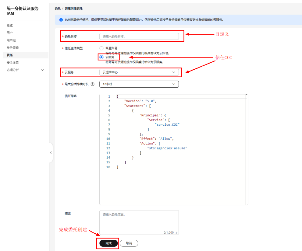
图 1-26 创建委托
