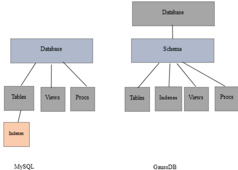
图 1-1 MySQL 和 GaussDB 中 Database 和 Schema 之间的差异
