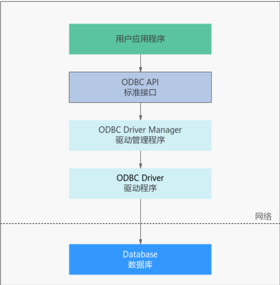
图 5-3 ODBC 系统结构
