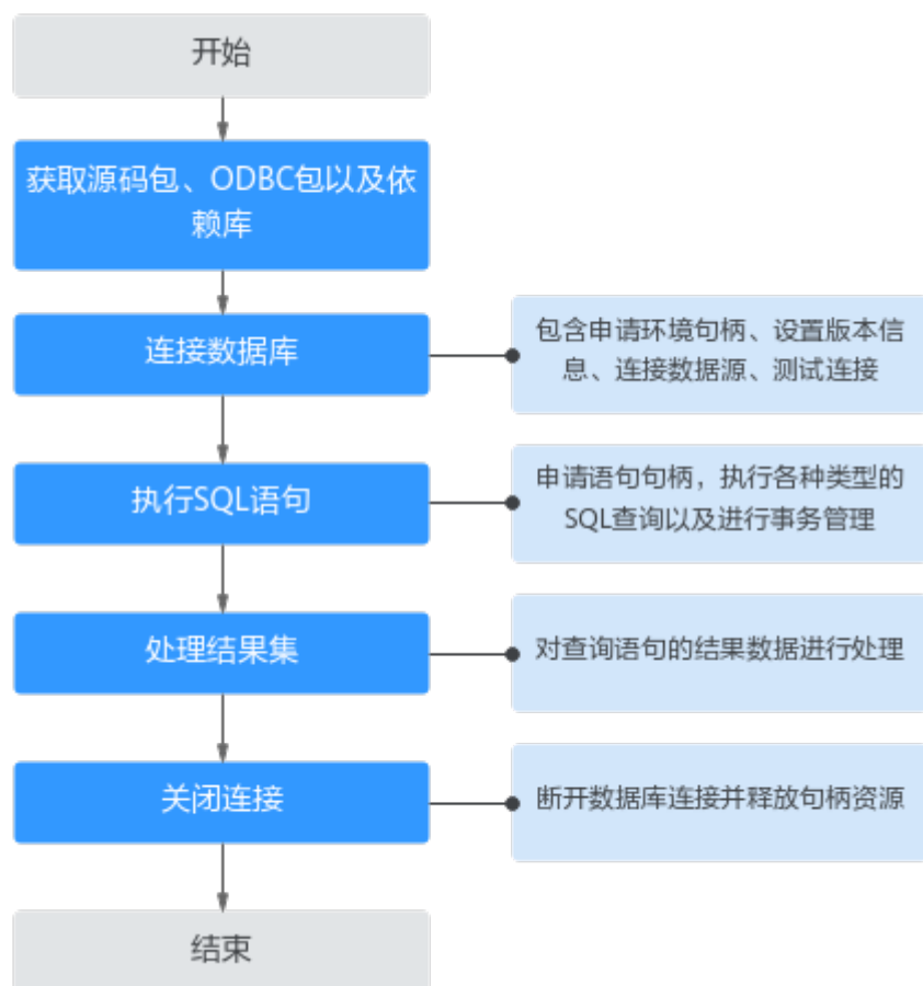
图 5-4 ODBC 开发流程
