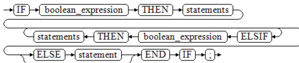
图 10-19 IF_THEN_ELSIF_ELSE::=
