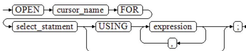
图 10-31 open_dynamic_cursor::=
