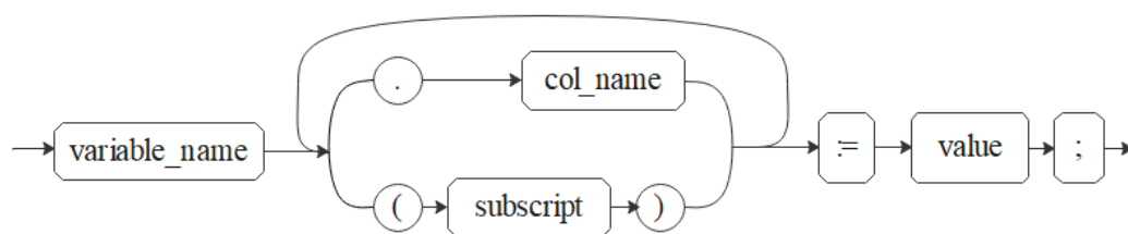
图 10-5 nested_assignment_value::=
