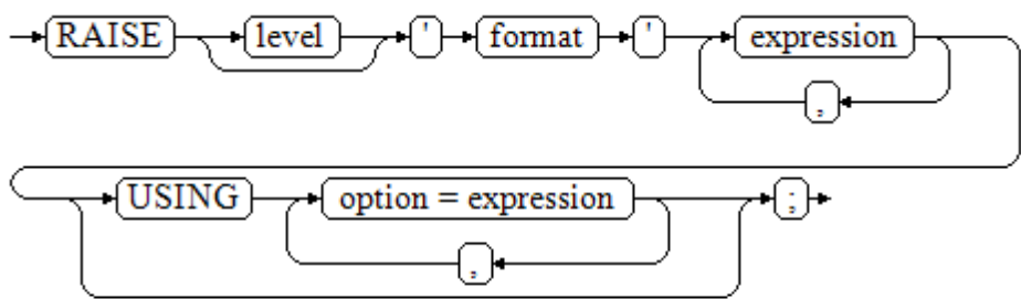
图 10-35 raise_format::=
