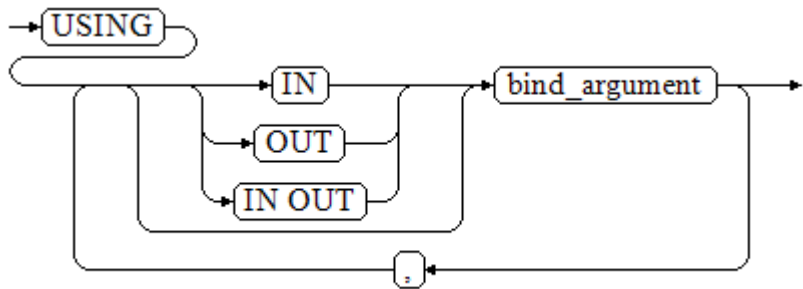
图 10-13 using_clause::=
