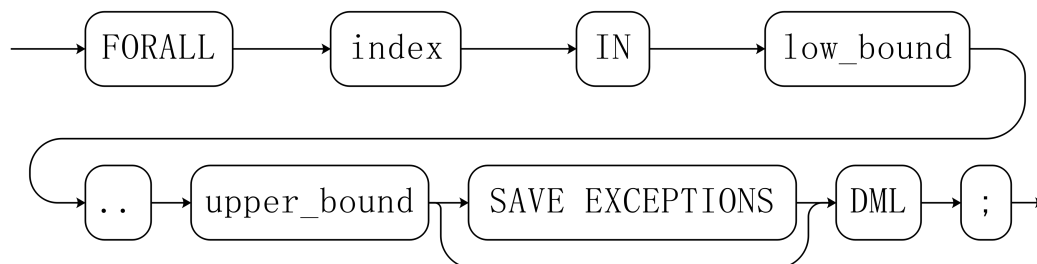
图 10-24 forall::=
