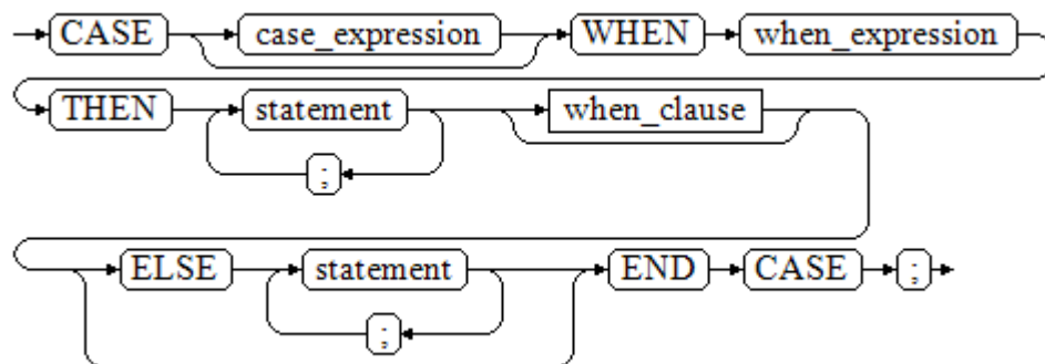
图 10-25 case_when::=
