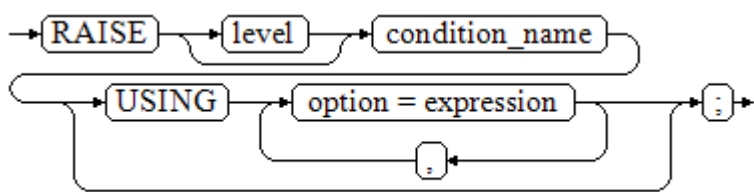
图 10-36 raise_condition::=
