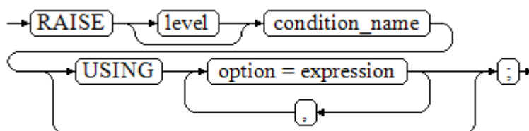
图 12-36 raise_condition::=
