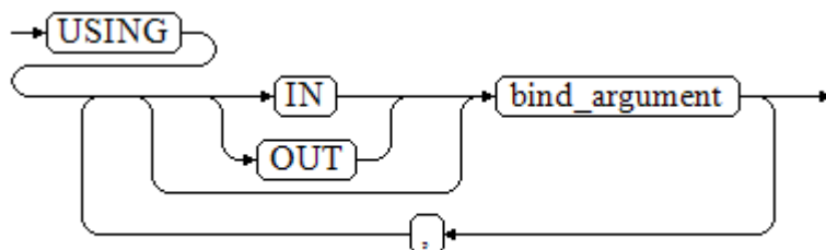
图 12-8 using_clause::=
