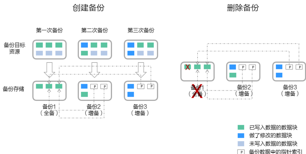
图 4-1 备份机制
