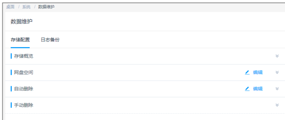
图 7-12 存储配置
