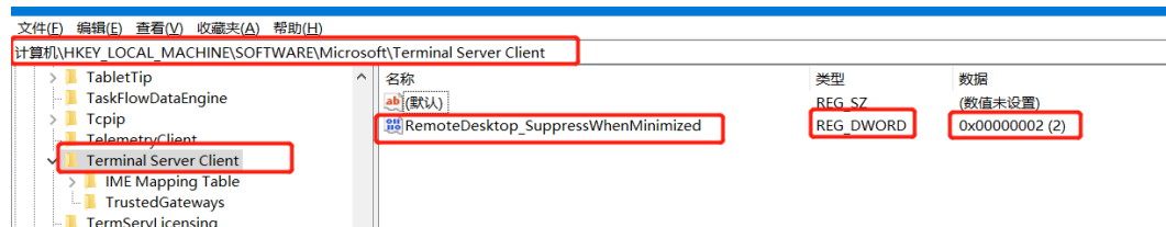
图 13-10 设置值大小
