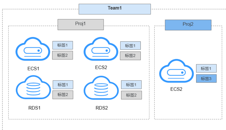
图 11-9 标签示例
