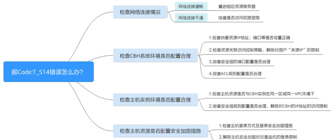
图 13-2 排查思路
