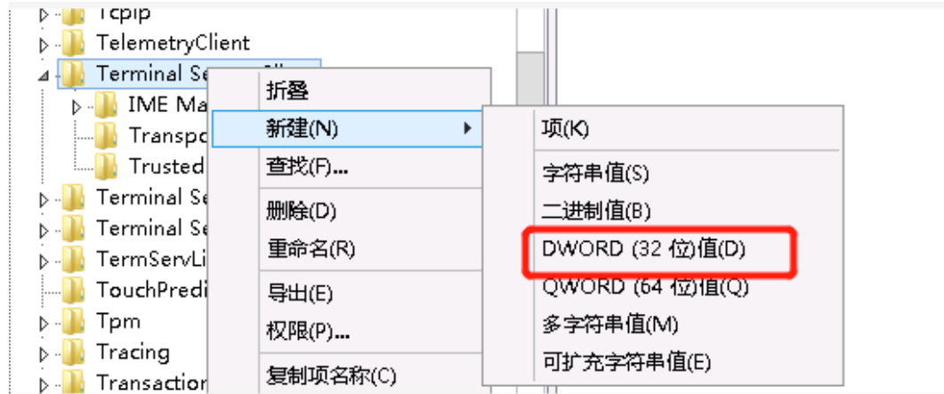
图 13-9 新建 DWORD
