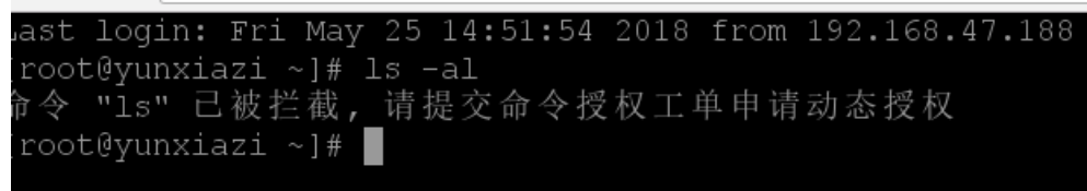
图 10-14 动态拦截
